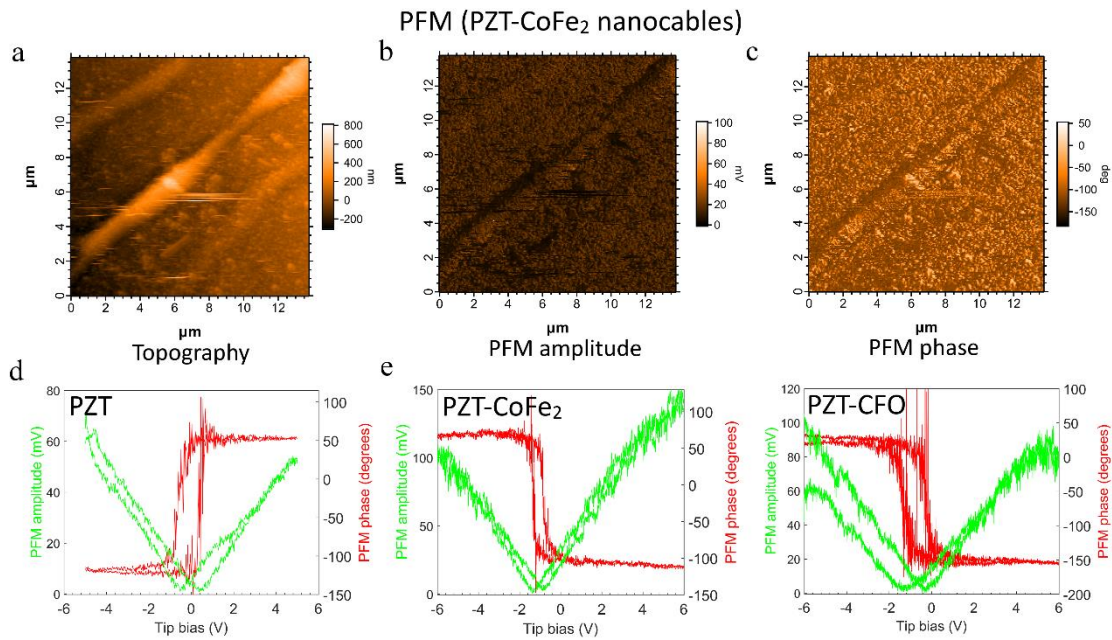
Figure 7: Microscopie à Force Piezoélectrique de nanocables PZT 500 -CoFe 2 : topographie (a), amplitude (b), et phase (c). Le renversement des domaines est illustré par les cycles d'hystérésis en phase (en rouge) and en amplitude (en vert) pour (d) un nanotube PZT 500 (3 imprégnations); (e) un nanocable PZT 500 -CoFe 2 ; (f) un nanocable PZT 500 -CFO 600 .
