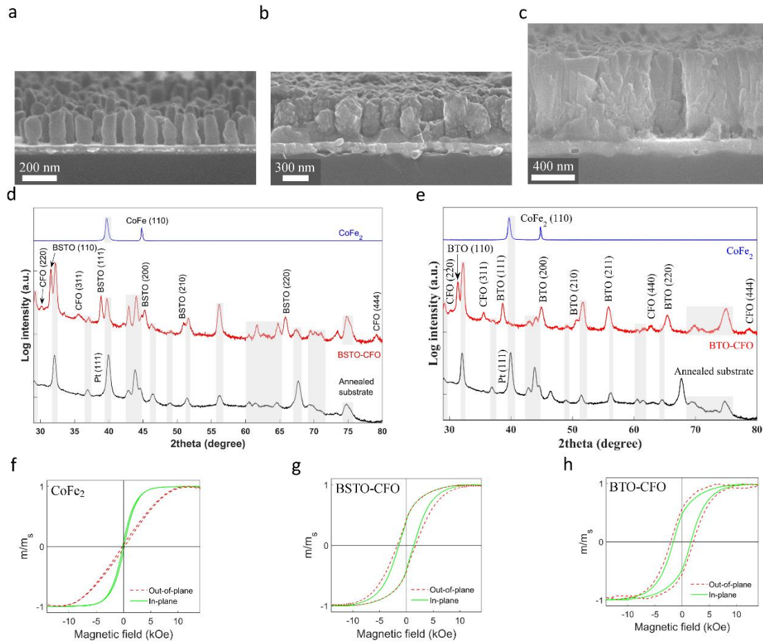
Figure 8: (a) Micrographies MEB : réseau de nanopiliers \text{CoFe}_2 . (b,c) nanostructures BSTO-CFO et BTO-CFO – Les films BSTO et BTO sont déposés par pulvérisation cathodique (d,e) Diagrammes de diffraction des rayons X en incidence rasante dans le plan pour un réseau de nanopiliers \text{CoFe}_2 (bleue), pour les nanostructures BSTO-CFO (d) et BTO-CFO (e) (rouge), le substrat Pt/Ti/Si recuit à \sim 600^\circ\text{C} est représenté en noir. Cycles d’hystérésis à température ambiante dans le plan (trait plein) and hors plan (traits pointillés) pour un réseau de nanopiliers \text{CoFe}_2 (f), pour les nanostructures BSTO-CFO (g) et BTO-CFO (h).
