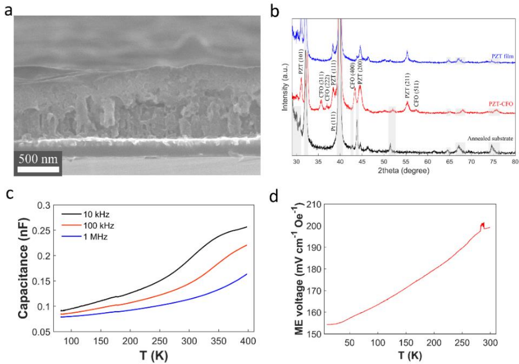
Figure 11: (a) Micrographie MEB du nanocomposite PZT-CFO obtenu par multi-impregnation de la couche PZT (b) Diffractogrammes des rayons X d'un film mince de PZT (bleue), du nanocomposite PZT-CFO (rouge) et du substrat Pt/Ti/Si (noir). PZT-CFO : variations thermiques (c) de la capacité et d) du coefficient magnétoélectrique
