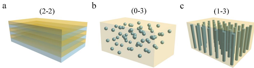
Figure 2: Illustrations schématiques des trois types de connectivité adaptés aux composites multiferroïques. (a) hétérostructure horizontale alternant des couches ferroélectriques et magnétiques, (2-2), (b) composite constitué de nanoparticules dans une matrice (0-3) et (c) hétérostructure verticale avec des nanopilliers dans une matrice (1-3).
