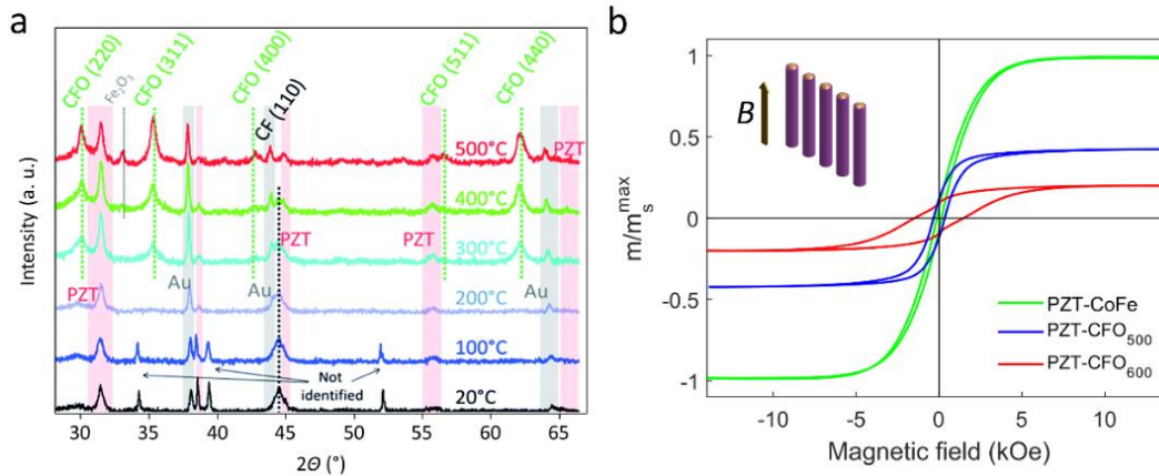
Figure 6: (a) Suivi de l'oxydation in-situ des nanofils \text{CoFe}_2 en CFO dans les nanotubes PZT par diffraction des rayons X à différentes températures (pas de 100^\circ\text{C} ). Le diffractogramme référence de \text{CoFe}_2 est représenté en noir et le diffractogramme de CFO (oxydation complète) est représenté en rouge. (b) Cycles d'hystérésis à température ambiante hors plan (parallèlement à l'axe des nanofils) pour un réseau de nanocables \text{PZT}^{500}\text{-CoFe}_2 (en vert), \text{PZT}^{500}\text{-CFO}^{500} (bleue) et \text{PZT}^{500}\text{-CFO}^{600} (rouge).
