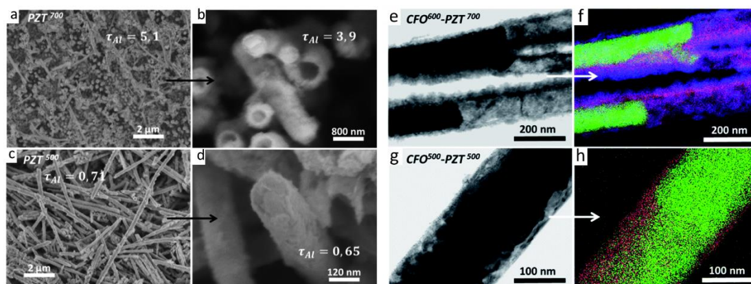
Figure 4: (a) and (b) Micrographies MEB-HR de nanocables \text{PZT}^{700}\text{-CFO}^{600} ( D_{\text{pore}} \sim 150 \text{ nm} ; P_{\text{membrane AAO}} \sim 35\% ) après dissolution dans \text{NaOH} 1 M. (c) et (d) Micrographies des nanocables \text{PZT}^{500}\text{-CFO}^{500} (températures de cristallisation et d'oxydation abaissées de 700^\circ\text{C} à 500^\circ\text{C} et de 600^\circ\text{C} à 500^\circ\text{C} , respectivement). (e) Micrographies STEM-BF des nanocables coeur-écorce \text{PZT}^{700}\text{-CFO}^{600} après dissolution de la membrane dans \text{NaOH} 1M and dispersion dans l'éthanol. (g) nanocables \text{PZT}^{500}\text{-CFO}^{500} . (f,h) cartographies élémentaires correspondantes, avec Pb, Fe and Al représentés en rouge, vert, et bleue, respectivement.
