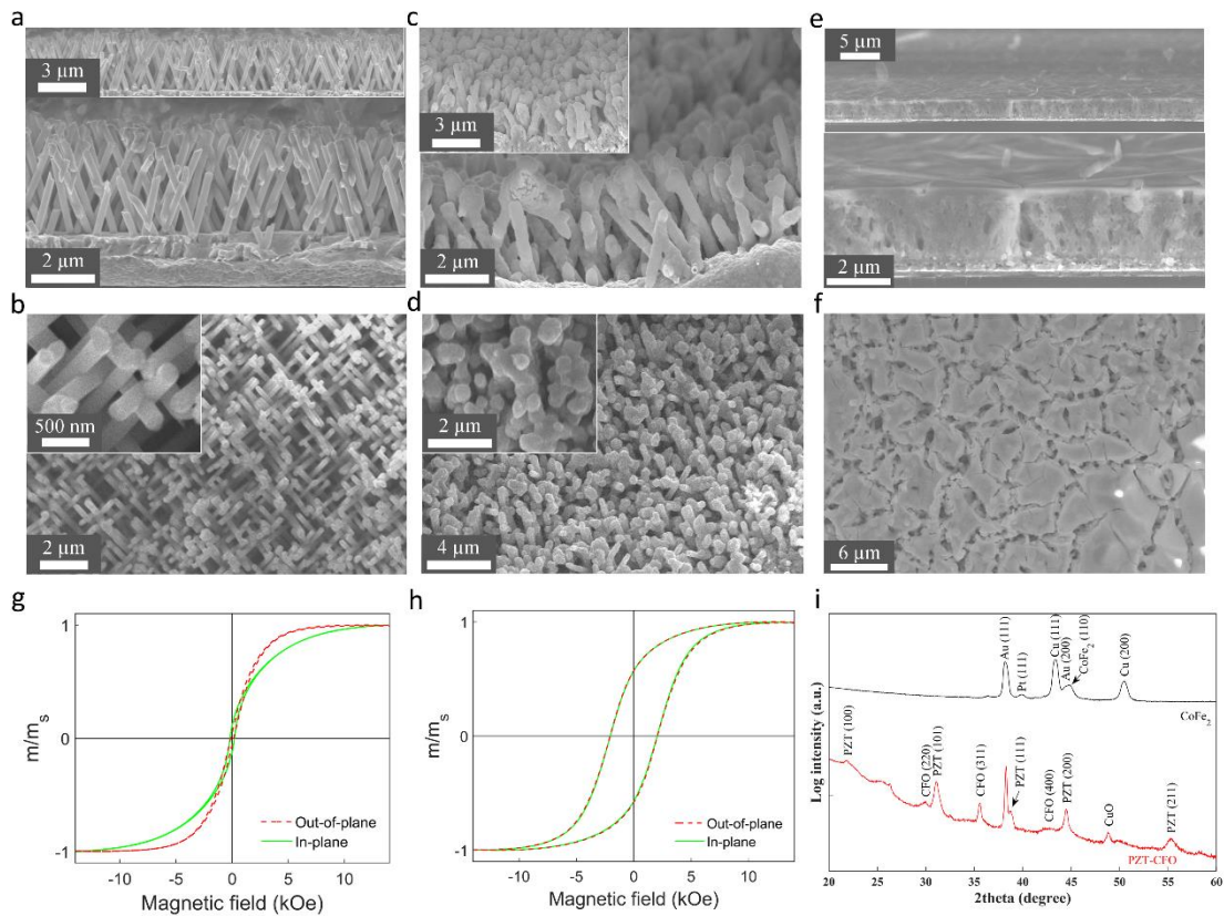
Figure 12: Micrographies MEB (vues inclinée et de dessus) : (a,b) réseau 3D de nanofils interconnectés CoFe 2 3D de diamètre D_{NW} \sim 230 nm (c,d) ces nanofils après oxydation en CFO par traitement thermique, (e,f) nanostructure PZT-CFO après : i) traitement thermique pour cristalliser la couche PZT, ii) oxydation in situ des nanofils CoFe 2 , et iii) un recuit supplémentaire.
