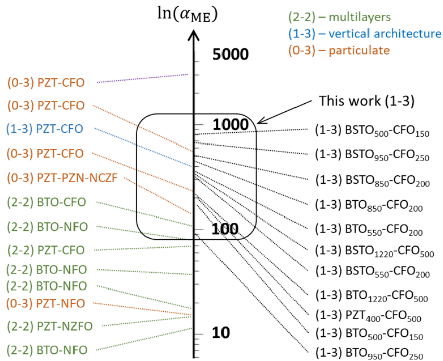
Figure 13: Comparaison entre les valeurs de coefficients magnétoélectriques obtenues au cours de ce travail de thèse (à droite) pour les architectures de connectivité (1-3) BSTO-CFO, BTO-CFO, et PZT-CFO et les valeurs de coefficients magnétoélectriques reportées dans la littérature (à gauche) pour des hétérostructures de diverses connectivités (multicouches (2-2), particules dans une matrice (0-3) et structures verticales constituées de nanopiliers dans une matrice (1-3))
