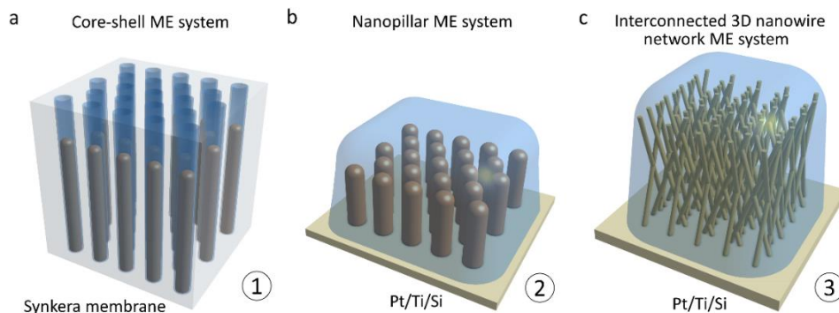
Figure 3: Illustrations des trois architectures de nanocomposites magnétoélectriques verticalement alignés. (a) PZT-CFO Cœur-écorce : réseau de nanocables dans une membrane commerciale d'alumine AAO (Synkera Co.) (b) BSTO-CFO, BTO-CFO, et PZT-CFO (1-3): réseau de nanopiliers ferromagnétiques dans une matrice ferroélectrique (c) PZT-CFO (3-3): réseau de nanofils ferromagnétiques interconnectés dans une matrice ferroélectrique.
