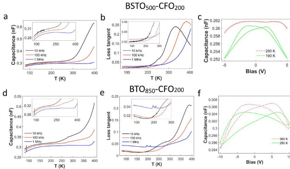
Figure 9: Evolutions de la capacité et des pertes diélectriques en fonction de la température et de la tension pour les nanocomposites BSTO-CFO (a-c) et BTO-CFO (d-f)
