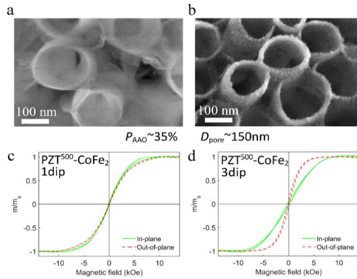
Figure 5: Images par microscopie électronique à balayage haute résolution de nanotubes \text{PZT}^{500} (température de cristallisation 500^\circ\text{C} - D_{\text{pore}} \sim 150 \text{ nm} , P_{\text{membrane AAO}} \sim 35 \% ) obtenus après (a) une et (b) trois imprégnations sol-gel successives dans la membrane d'alumine AAO. Cycles d'hystérésis à température ambiante dans le plan de la direction facile d'aimantation (trait plein) et hors plan (traits pointillés) pour un réseau de nanocables \text{PZT}^{500}\text{-CoFe}_2 constitués de nanotubes PZT obtenus après 1 imprégnation (c) et 3 imprégnations (d)
