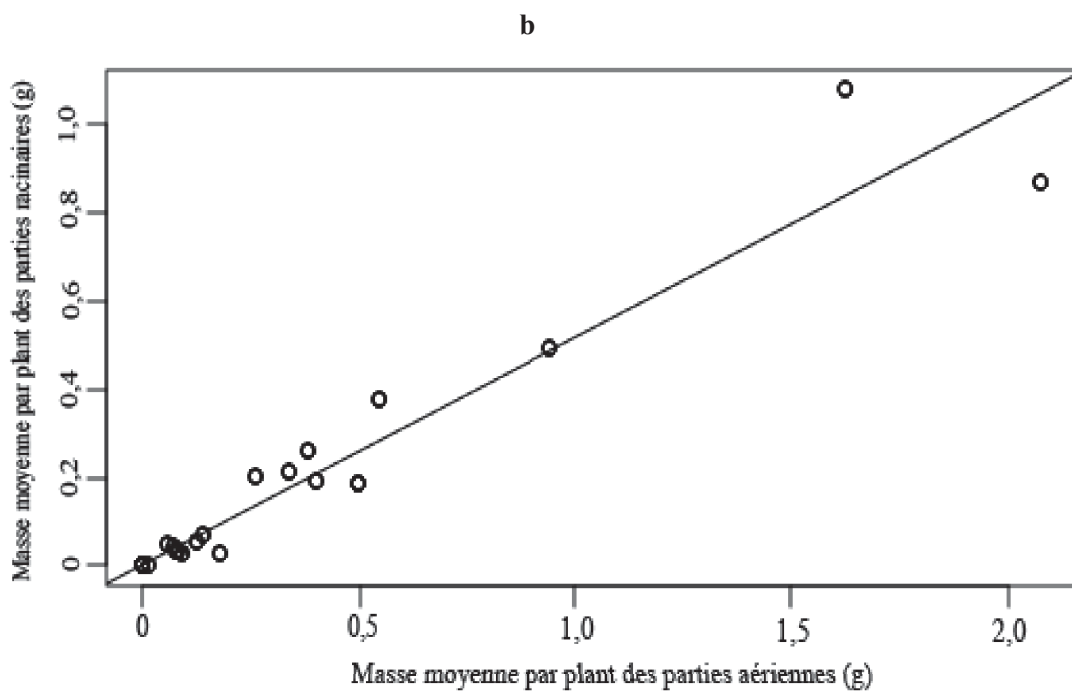
Figure 2 : Droite de régression de la biomasse moyenne par plant entre les parties aériennes et racinaires sur les plants après 14 mois de développement : a : A. spirorbis ; b : E. terreticornis
