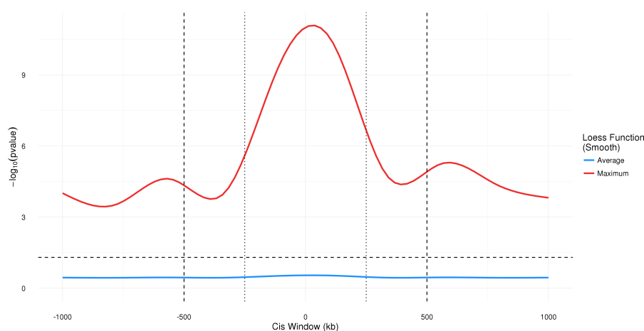
FIGURE 28. Distribution des valeurs-p d'association entre les SNPs et l'expression des gènes à moins d'un mégabase du promoteur du gène.
