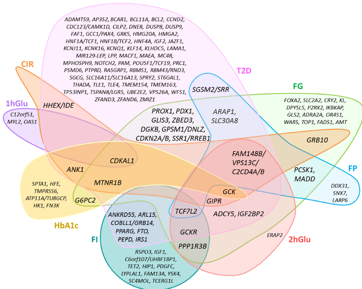
FIGURE 9. Diagramme de Venn des loci identifiés par études d'association pangénomiques pour leur effet sur différents traits glycémiques et le diabète de type 2 [Marullo et al., 2014]. T2D : diabète de type 2 ; FG : glycémie à jeun ; FI : insulinémie à jeun ; FP : proinsulinémie à jeun ; 2hGlu : glycémie à 2 heures ; HbA1c : hémoglobine glyquée ; CIR : ratio carbohydrate-insuline.
