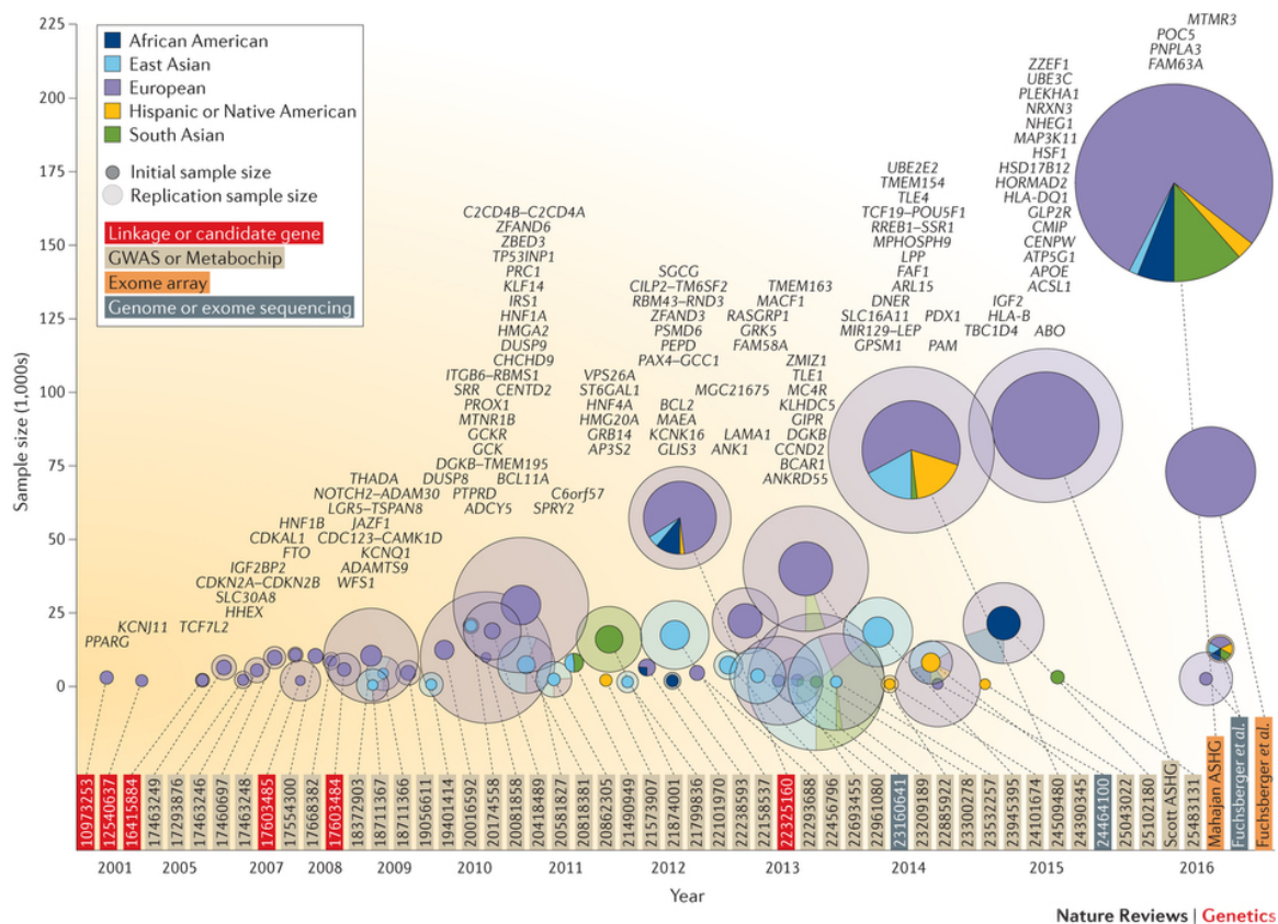
FIGURE 10. Historique des loci de susceptibilité au diabète de type 2 identifiés par études d'association pangénomiques [Flannick and Florez, 2016].
