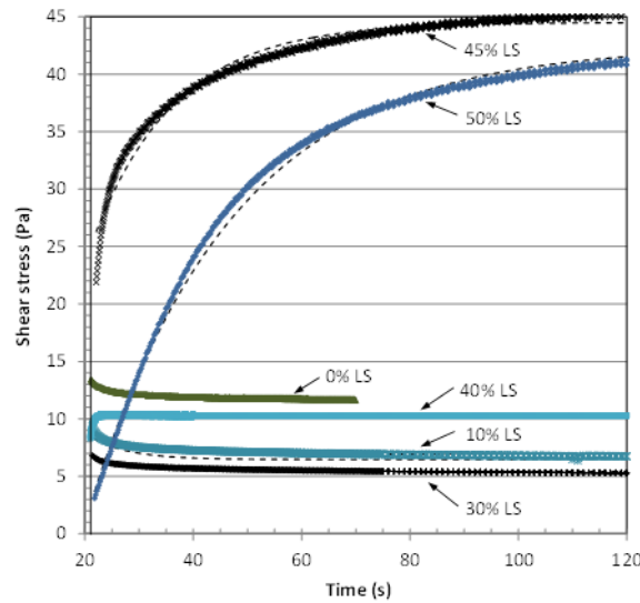
Figure 2 La réponse de la contrainte de cisaillement après une chute brutale du taux de cisaillement de 1000 à 0.1 s -1 pour la série de 2% MFC. Les lignes pointillées représentent les résultats de fitting selon Équation 3.
