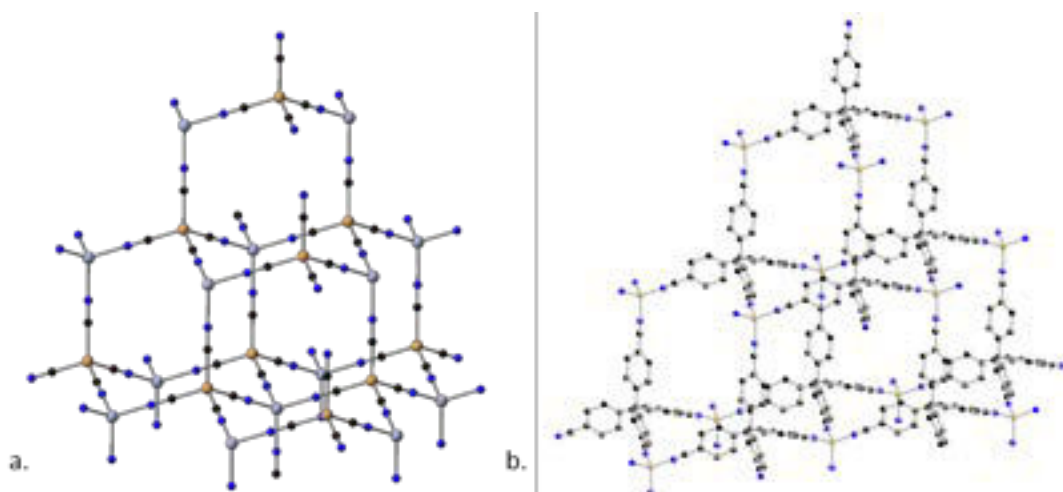
Fig. 8. Structures cristallines des réseaux obtenus à partir de \text{Zn}(\text{CN})_2 et de sels de cuivre (I) (a) et à partir de tétra-(cyanophényl)-méthane et de sels de cuivre (I) (b) par le groupe de Robson. 29
