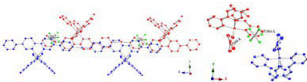
Fig. 118.a. Portion de la structure cristalline de [\text{Ir}(\text{Fppy})_2(\text{bpy-4py})][\text{PF}_6^-]\cdot\text{Ag} montrant l'arrangement parallèle de chaînes homochirales \Delta , et l'empilement centrosymétrique, parallèle, décalé, des plans homochiraux. (L'énantiomère \Delta est représenté en bleu et l'énantiomère \Lambda en rouge. Les atomes d'hydrogène, les anions \text{PF}_6^- ainsi que les molécules de solvant ont été omis par soucis de clarté.)
