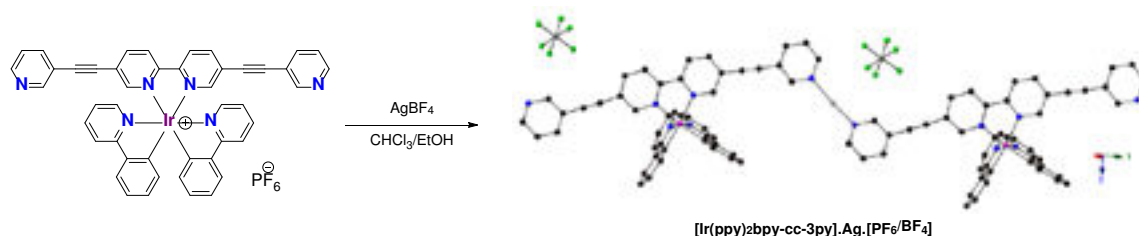
Fig. 119. Schéma de synthèse et structure cristalline du réseau [\text{Ir}(\text{ppy})_2(\text{bpy-cc-3py})][\text{PF}_6/\text{BF}_4]\cdot\text{Ag}
