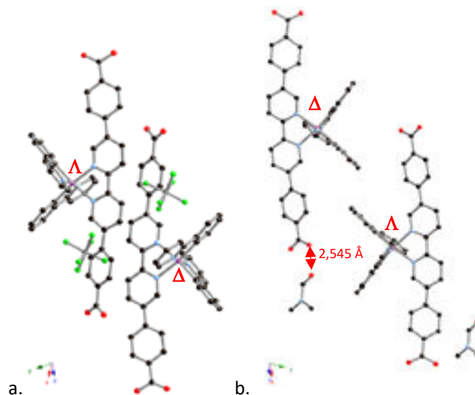
Fig. 90. a. Structure cristalline de [Ir(ppy)_2(bpy-4CO_2H)][PF_6] montrant les deux énantiomères. Les atomes d'hydrogène ainsi que les molécules de solvant ont été omis pour plus de clarté. b. Représentation de la liaison hydrogène entre le complexe et le solvant.
