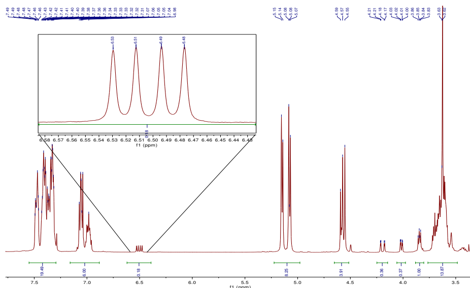
Fig. 152. Spectre RMN ^1\text{H} ( \text{CDCl}_3 , 300 MHz) du brut réactionnel après réaction entre les composés 143b et le ( S,S )-1,2-cyclohexanediol mettant en évidence la formation d'alcène par réaction d'élimination du groupement mésylate.
