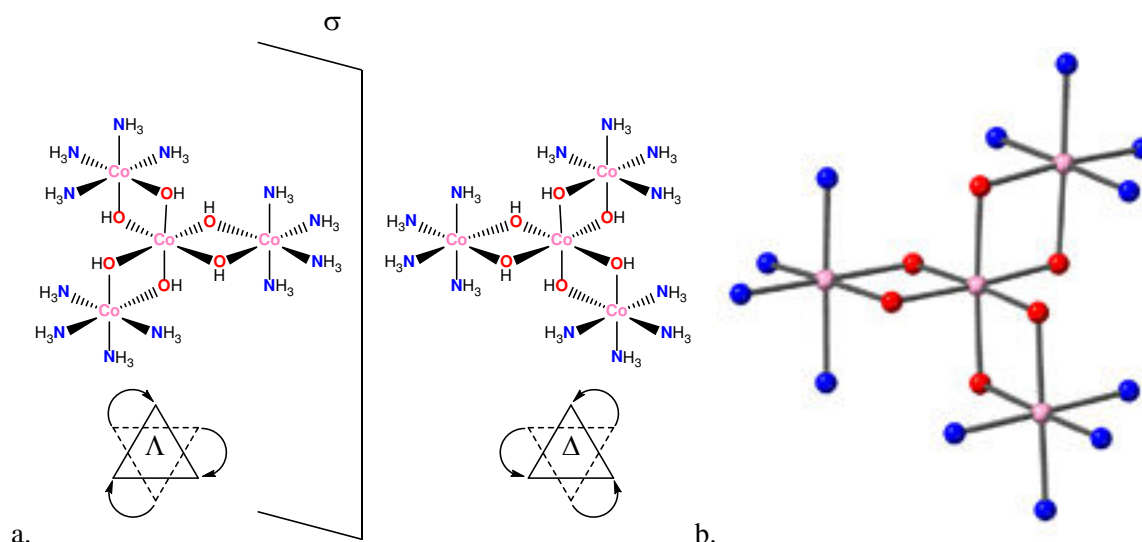
Fig. 32. a. Représentation des énantiomères \Lambda et \Delta de l'hexol de A. Werner. b. Structure cristalline de \Delta -[Co 4 (NH 3 ) 12 (OH) 6 ] 6+ .
