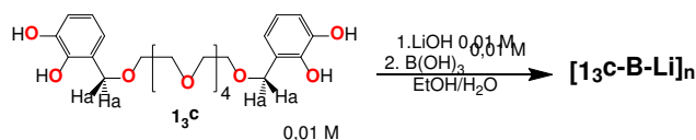
Schéma 27. Schéma de synthèse de la réaction en présence de bore pour la formation de [\mathbf{1}_3\mathbf{c}\text{-B-Li}]_n .
