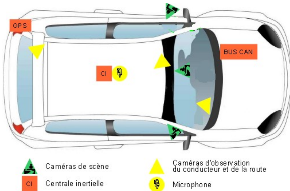
Figure 21 : Illustration de l'instrumentation du véhicule VOICIE utilisé en situation réelle de conduite
