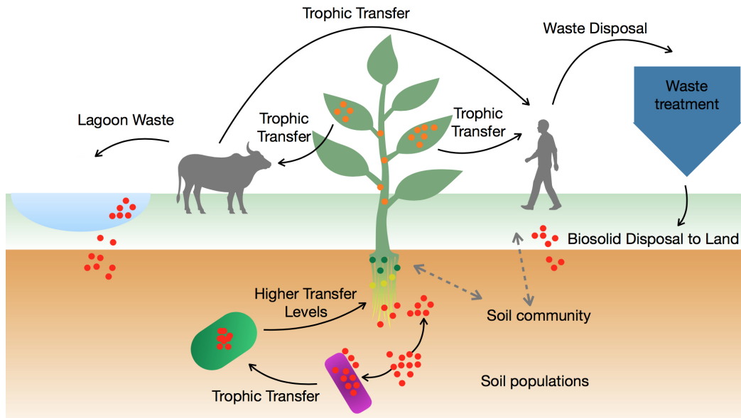
FIGURE 1.10 – Schéma conceptuel du transfert des nanomatériaux dans un écosystème terrestre (HOLDEN et al. 2012). Les nanomatériaux (points rouges) peuvent être ad/absorbés aux bactéries (violet) et aux protozoaires (vert) à partir du sol ou via le transfert trophique. Les nanomatériaux peuvent également interagir avec les racines des plantes, incluant les relations symbiotiques (points jaunes et verts des racines). Transférés aux parties aériennes des plantes, les nanomatériaux peuvent changer chimiquement (points oranges). Les nanomatériaux peuvent impacter le développement des populations et des communautés bactériennes (graphiques). Le transfert trophique (flèches noires), la bioaccumulation et la bioconcentration des nanomatériaux sont envisageables pour l'ensemble des organismes de l'écosystème terrestre. À noter également, les flux de nutriments (flèches serpentiformes) peuvent être modifiés en raison des changements des communautés microbiennes du sol et des plantes, ou indirectement si la présence des nanomatériaux induit une altération de la physicochimie du sol, et donc des flux d'eau et de nutriments.
