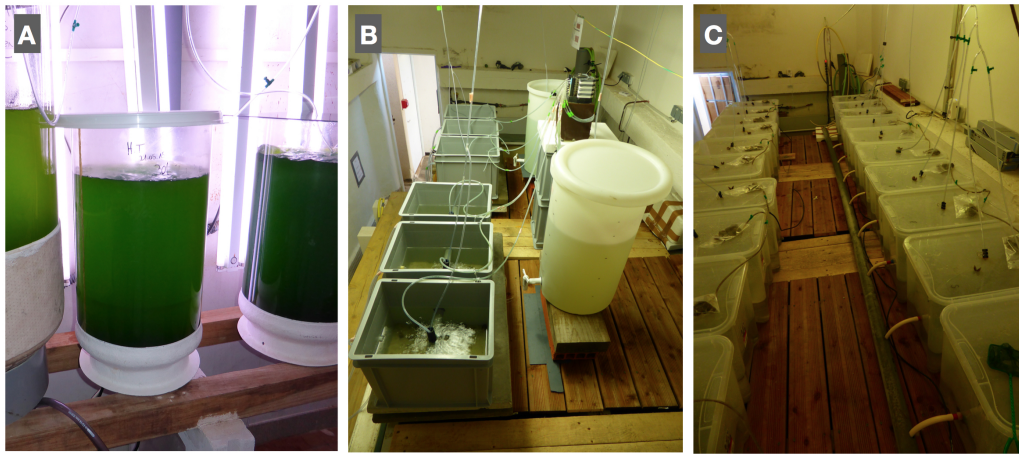
FIGURE 2.6 – Photographies des différentes étapes de l'expérimentation à trois maillons trophiques. (A) Cultures des algues Scenedesmus sp. (B) Réserve d'algues (à droite) alimentant les bacs d'exposition des bivalves (à gauche). (C) Exposition trophique et individualisée des anguilles dans un dispositif en circuit ouvert.
