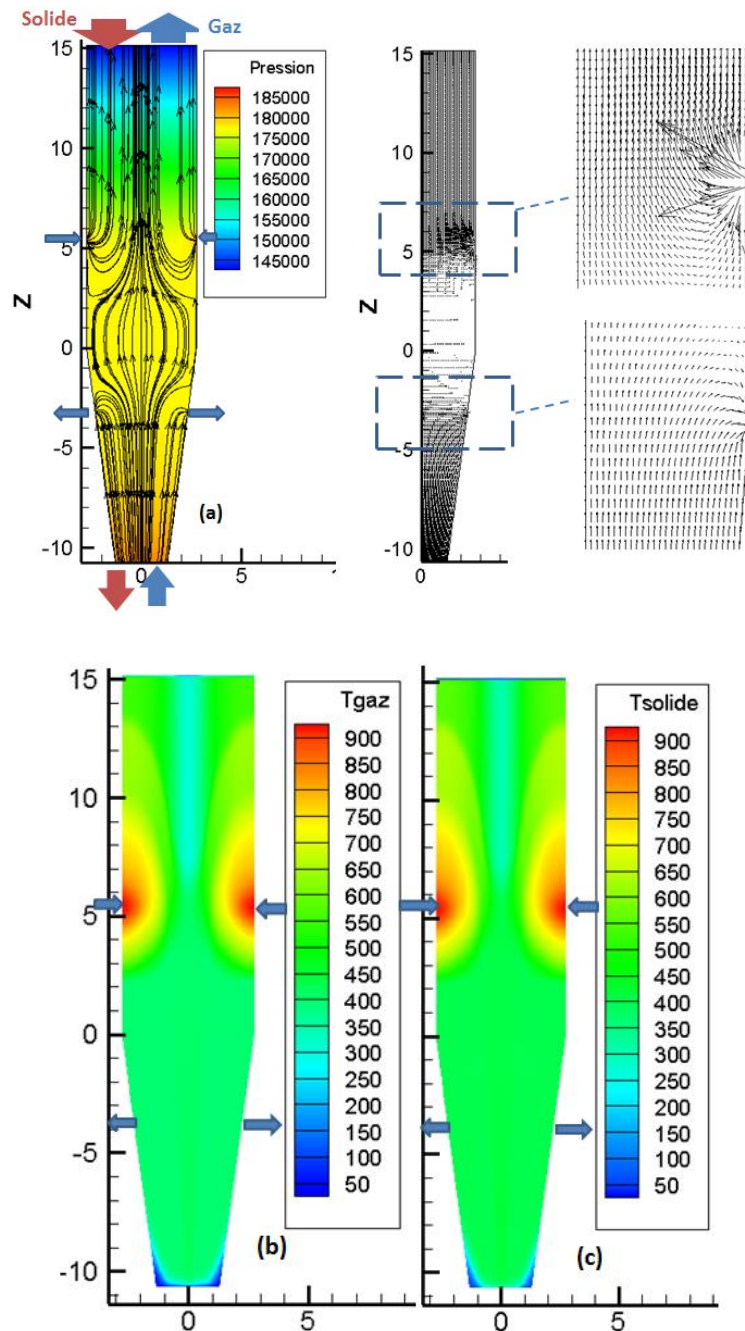
Figure II-12 : (a) Champ de pression (Pa), lignes de courant et vecteurs vitesses du gaz dans le réacteur, (b) distribution de température (°C) dans la phase gazeuse, (c) distribution de température (°C) dans les solides
