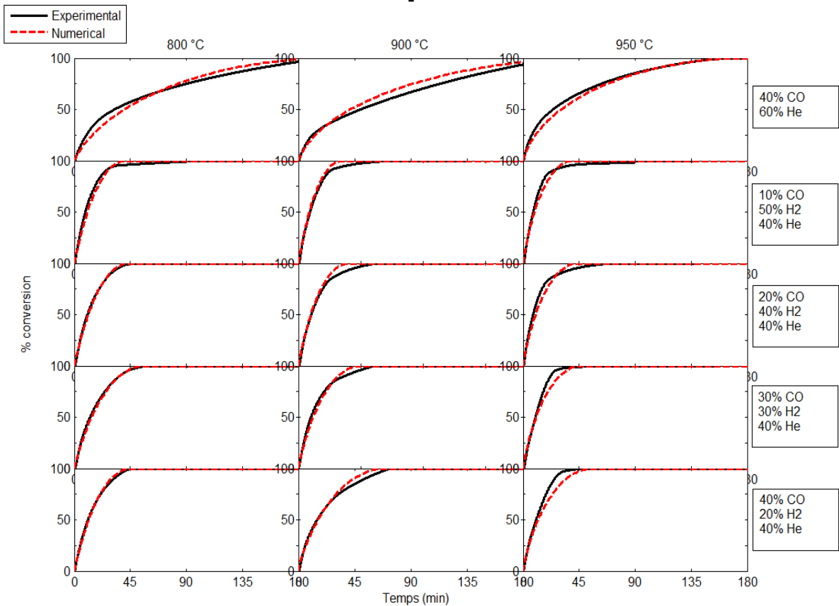
Figure I-16 : Seconde comparaison des résultats cinétiques du modèle avec les essais thermogravimétriques avec CO pur (dans He) et avec les mélanges H 2 -CO-He, après la prise en compte du dépôt de carbone
