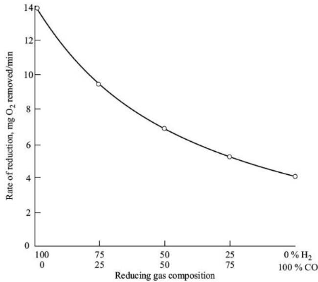
Figure I-7 : L'effet de composition de gaz sur la vitesse de réduction de boulette dense à 1000°C [29]
