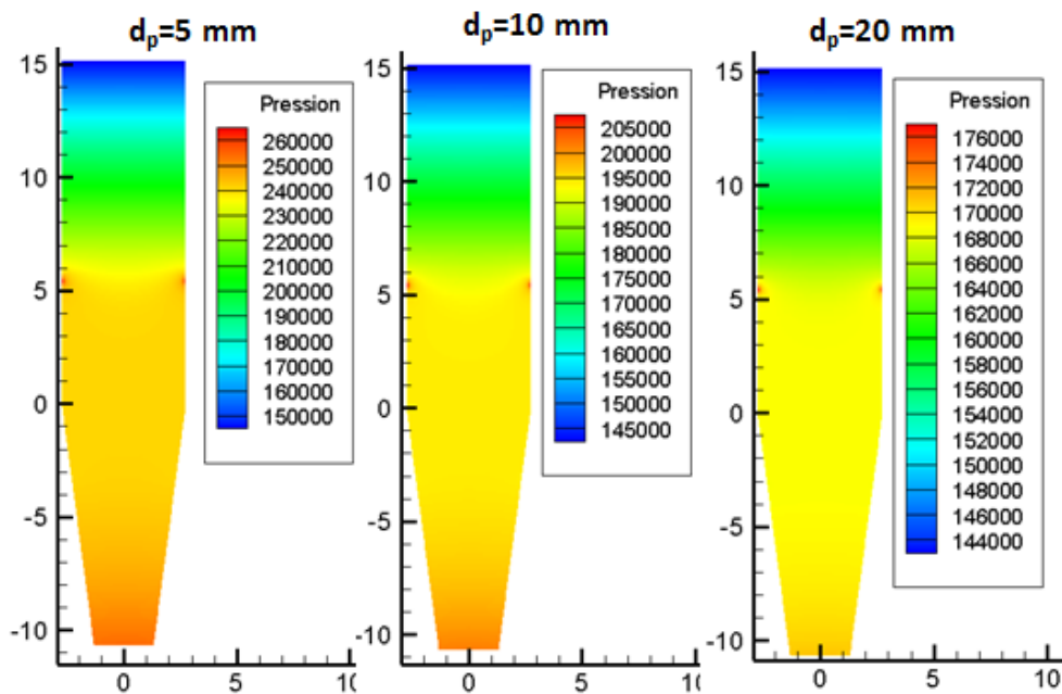
Figure III-17 : Effet du diamètre des boulettes sur le champ de pression en Pa
