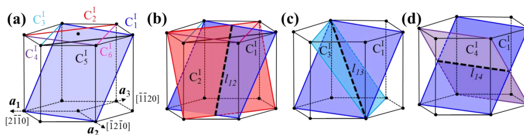
Fig. 5. 4 (a) les 6 variants de macle \{11\bar{2}2\}\langle 11\bar{2}\bar{3}\rangle (notés C_i^I ) forment 3 types de jonctions maclées (notées TTJ pour Twin-Twin Junction). (b) le Type I C_{i,j+1}^I avec la ligne d'intersection [0\bar{2}23] ; (c) le Type II C_{i,j+2}^I avec la ligne d'intersection [2\bar{4}23] ; (d) le Type III C_{i,j+3}^I avec la ligne d'intersection [1\bar{1}00] . La ligne d'intersection est représentée par une ligne noire en gras et en pointillé.
