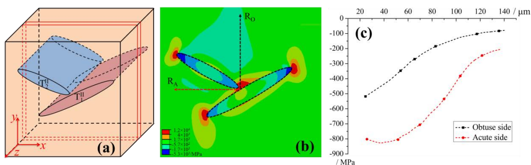
Fig. 3. 2 (a) Schéma du modèle en éléments finis. (b) RSS associées aux 2 variants de macles T_2^I et T_5^I . (c) Variation de la RSS (MPa, axe vertical) le long des 2 directions R_O et R_A ( \mu\text{m} , axe horizontal). La RSS provient des contraintes résiduelles dues à la jonction macle-macle.
