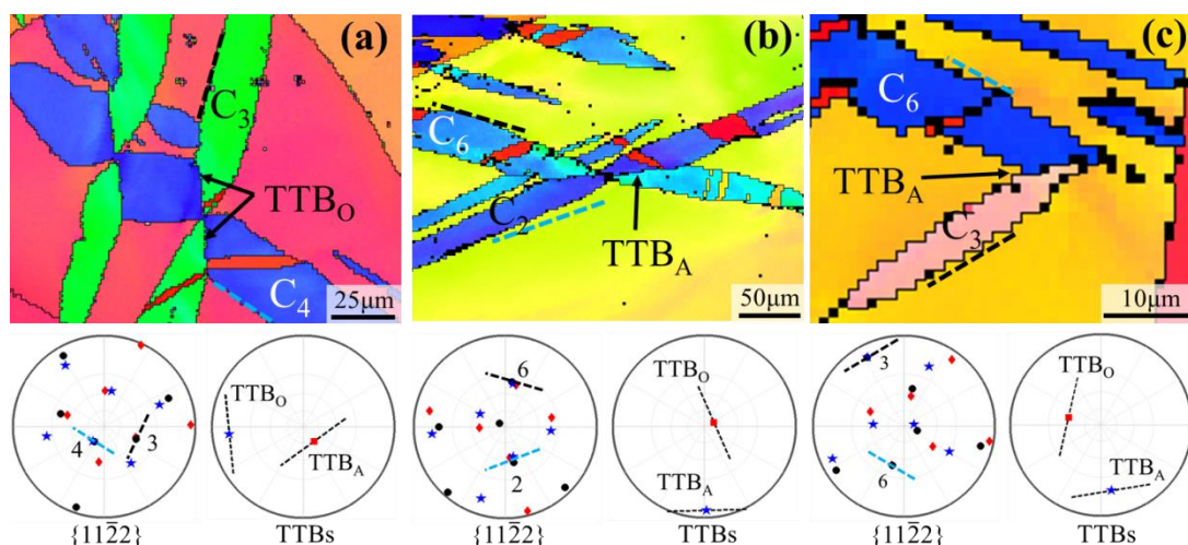
Fig 5.2. Différentes microstructures avec des jonctions maclées : (a) type C_1^I-C_2^I , (b) type C_1^I-C_3^I , (c) type C_1^I-C_4^I et leurs figures de pôles \{11\bar{2}2\} . Les lignes pointillées dans la figure de pôle \{11\bar{2}2\} indiquent les traces TTB_A et TTB_O associées aux jonctions maclées.
