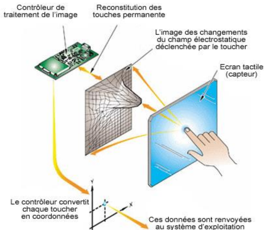
Image 27 : Schéma d'un écran utilisant la technologie capacitive
