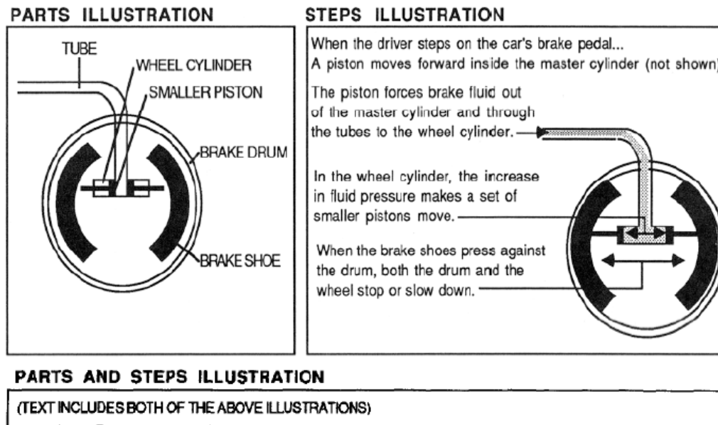
Image 34 : Document contenant illustration + noms, illustration + texte explicatif, illustration + noms + texte explicatif du système de freinage (Mayer et Gallini, 1990).
