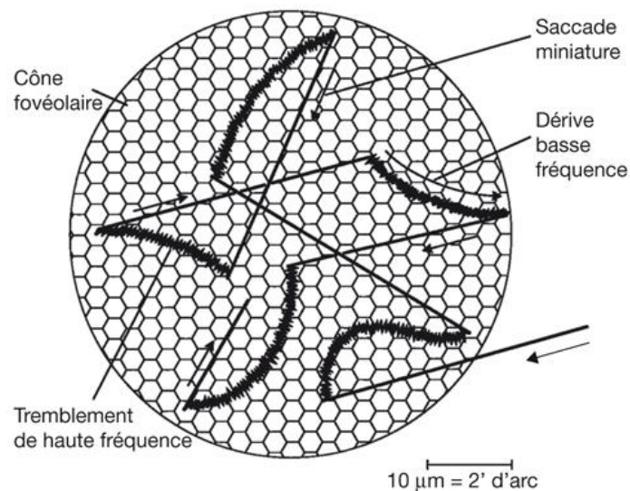
Figure 13 : Mouvements microscopiques de l'œil pendant la fixation.
