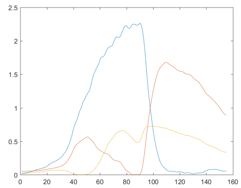
(d) NMF-BPP
