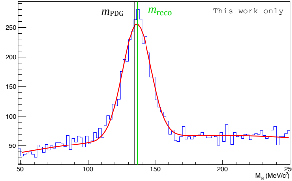
FIGURE 5.3 – Distribution en masse invariante pour une tour donnée avec ajustement (courbe rouge). La valeur de masse reconstruite provenant de l'ajustement est indiquée par la ligne verte et celle de la valeur PDG par la ligne noire.
