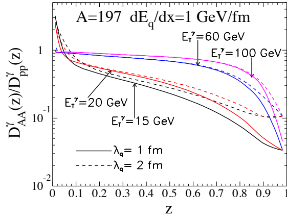
FIGURE 8.1 – Rapport des fonctions de fragmentation d'un jet émis dos à dos à un photon direct pour des collisions Au – Au centrales avec un libre parcours moyen de 1 fm (lignes pleines) et 2 fm (lignes pointillées) [208].
