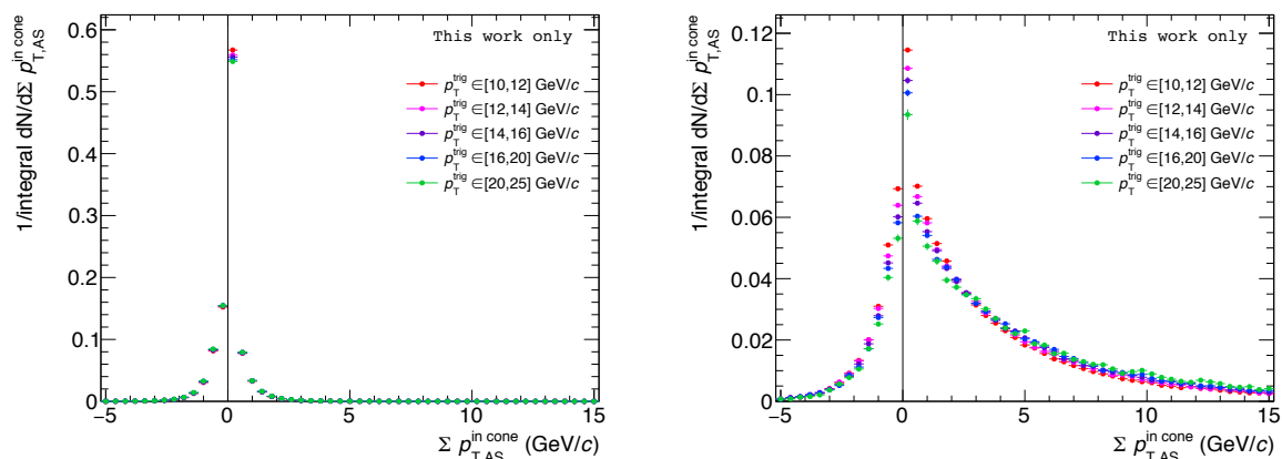
FIGURE 7.9 – Distributions en \Sigma p_{T,AS}^{in\ cone} après soustraction de l'événement sous-jacent pour différents intervalles en p_T^{trig} (différentes couleurs), pour la simulation GJ (gauche) et les données à petit \lambda_0^2 (droite).
