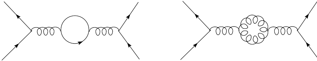
FIGURE 1.2 – Diagrammes de Feynman représentant la polarisation du vide avec une boucle de quark (gauche) et une boucle de gluon (droite).
