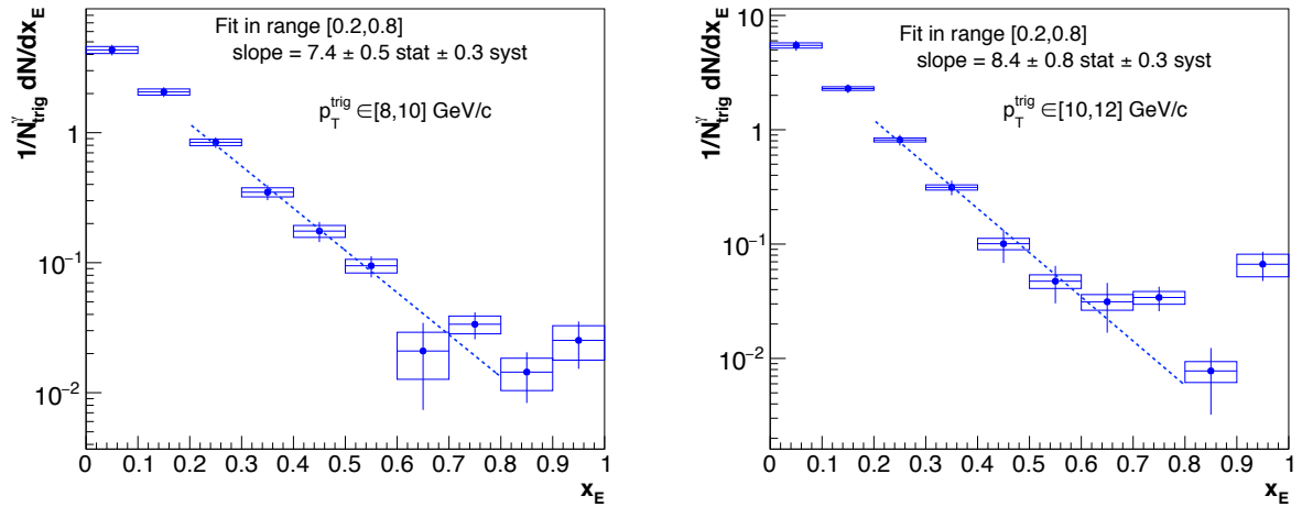
FIGURE C.4 – Distributions en x_E pour un p_T^{\text{trig}} compris entre 8 et 10 GeV/c (à gauche) et entre 10 et 12 GeV/c (à droite).
