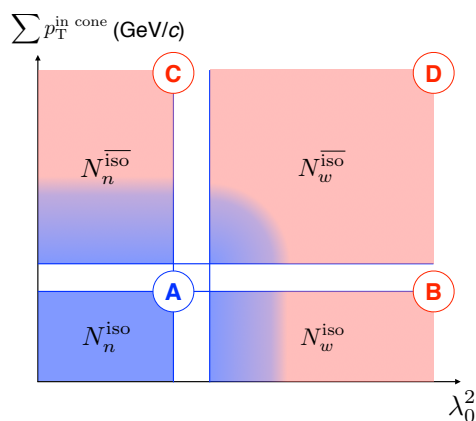
FIGURE 6.16 – Schéma de l'espace des phases en isolation et \lambda_0^2 , avec les quatre zones nécessaires au calcul de la pureté.
