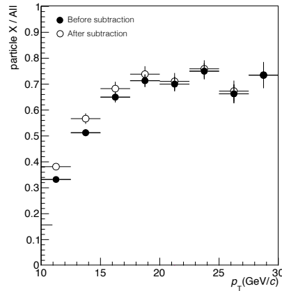
FIGURE 8.4 – Pureté obtenue par simulation GJ + JJ_{3,5} . Les ronds ouverts noirs correspondent à la pureté obtenue après soustraction de la contribution des photons de décroissance appariés provenant de \pi^0 et \eta .
