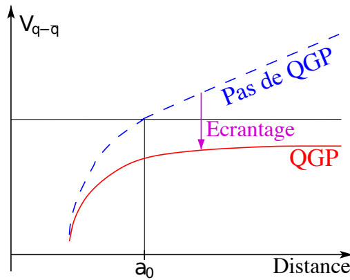
FIGURE 2.1 – Potentiel d'interaction entre quarks V_{q-\bar{q}} en fonction de la distance r les séparant. La courbe bleue en pointillés représente l'interaction pour des conditions standard de densité de charges de couleur. La courbe rouge pleine représente le potentiel écranté lorsque la densité de charges de couleur est élevée.
