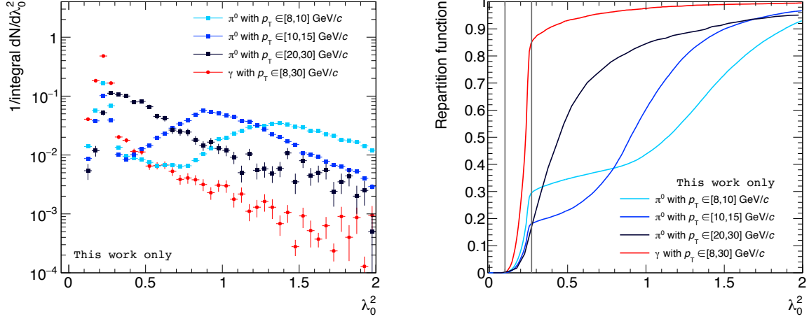
FIGURE 6.8 – Gauche : Distributions normalisées à l'intégrale du paramètre \lambda_0^2 pour les photons directs avec un p_T \in [8,30] GeV/c (carrés rouges), les \pi^0 avec un p_T \in [8,10] GeV/c (ronds bleu clair), [10,15] GeV/c (ronds bleus) et [20,30] GeV/c (ronds bleus foncés). Droite : Fonctions de répartition des distributions en \lambda_0^2 . La coupure en \lambda_0^2 appliquée pour sélectionner les photons est indiquée par les traits gris verticaux.
