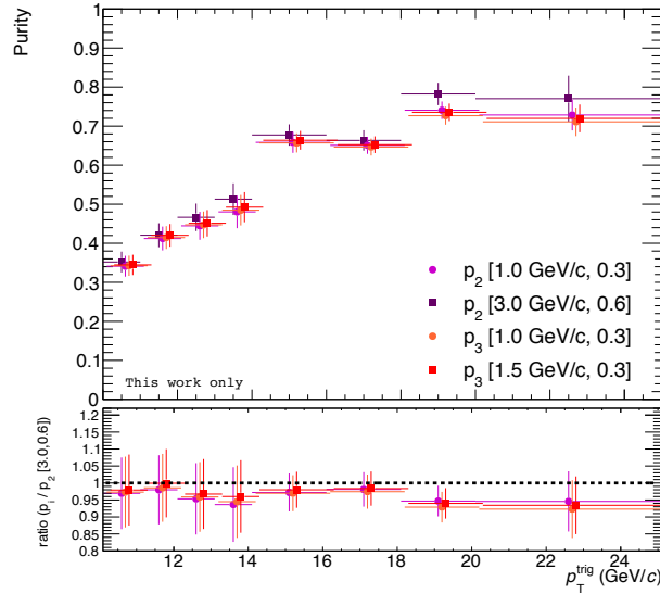
FIGURE 6.32 – Puret  \mathbb{P}_2 et \mathbb{P}_3 en fonction de p_T^{trig} pour les valeurs de coupures indiqu es dans le tableau 6.6.
