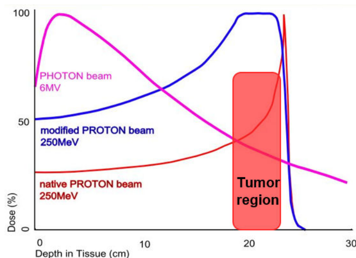
Figure 7.1 Dose déposée en fonction de la profondeur du tissu pour trois méthodes de traitement différentes : irradiation par un faisceau de photon de 6 MeV (en rose), par un faisceau de protons de 250 MeV natif (en rouge) et modifié (en bleu). Figure adaptée à partir du site internet de University College London ( https://www.hep.ucl.ac.uk/pbt/ ).
