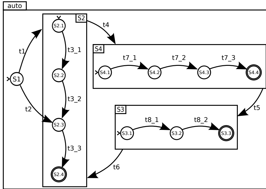
figure 3.3 – Un exemple d'automate
