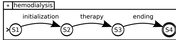
figure 5.13 – Spécification abstraite
