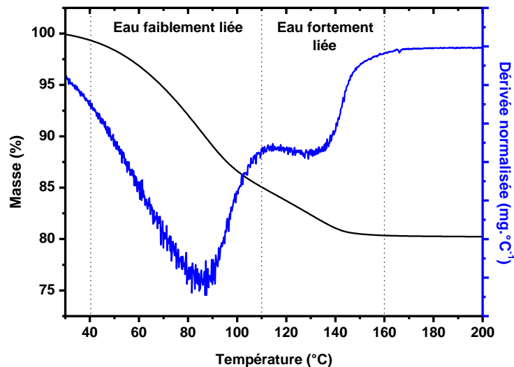
Figure II-13. Courbes ATG (en noir) et DTG (en bleu) de la saponite placée à 97% d'humidité relative. La courbe DTG permet de mieux visualiser les différentes zones de perte de masse. Il est ainsi possible de déterminer les pourcentages d'eau plus ou moins liée
