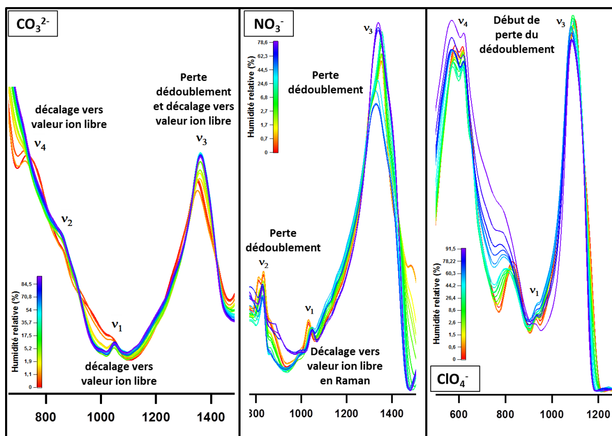
Figure V-24. Agrandissement des bandes infrarouge associées aux modes de vibration des anions en fonction de l'humidité relative. Certains dédoublements mal résolus ne sont pas visibles et se traduisent par une bande large avec des épaulements qui disparaissent avec l'augmentation de l'humidité relative
