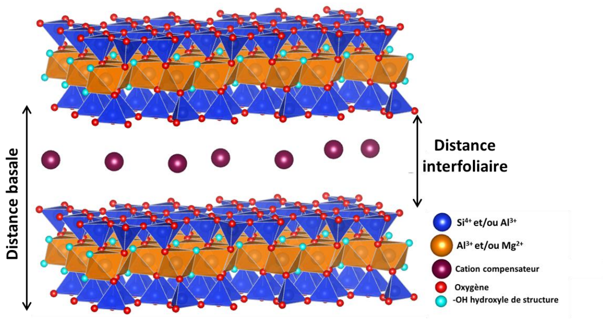
Figure I-9. Représentation d'une argile 2:1 présentant un déficit de charge dans les feuillets compensé par l'insertion de cations compensateurs dans l'espace interfoliaire
