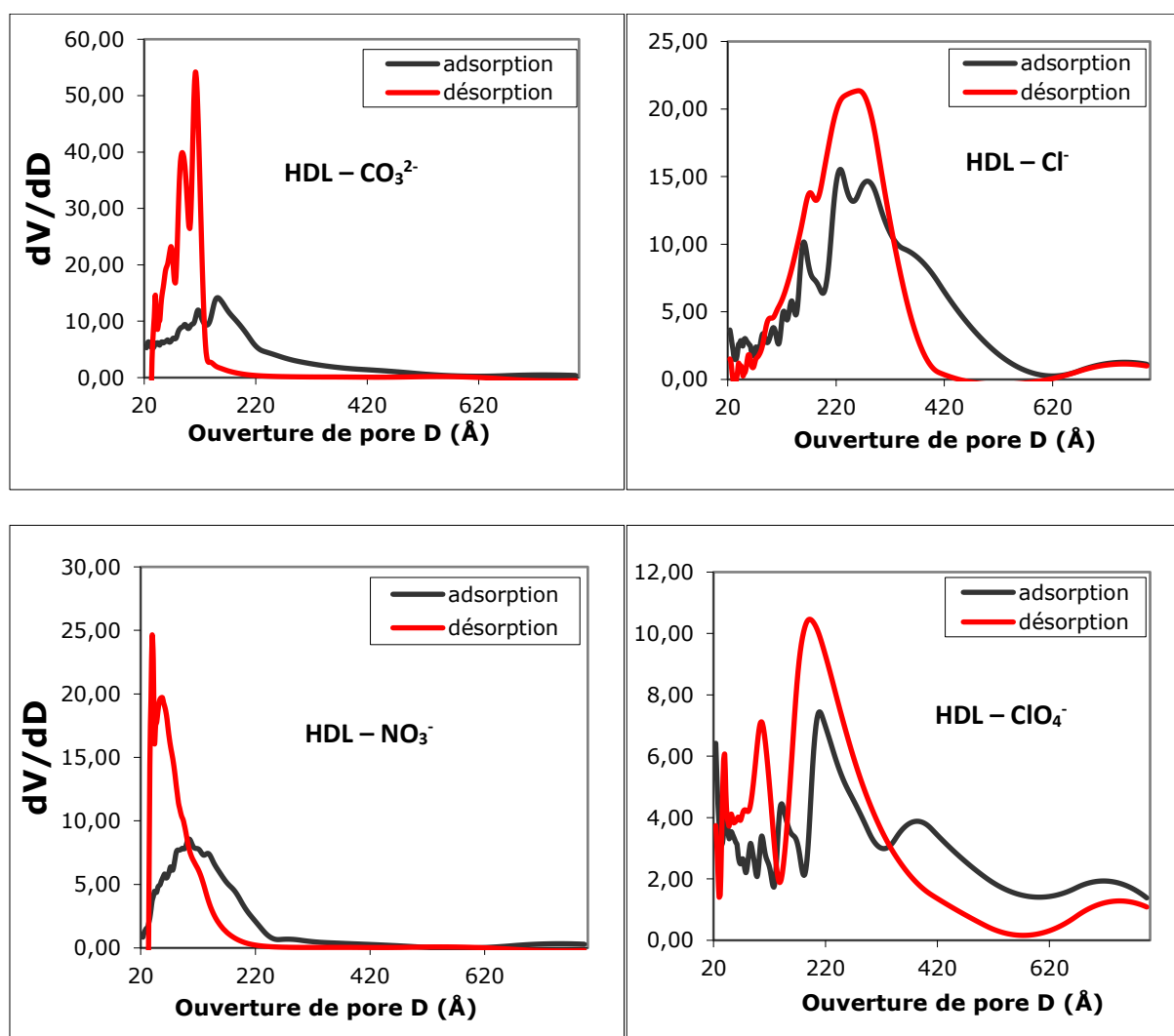
Figure V-13. Graphiques représentant la distribution en taille de la mésoporosité lors de l'adsorption, en noir, et de la désorption, en rouge
