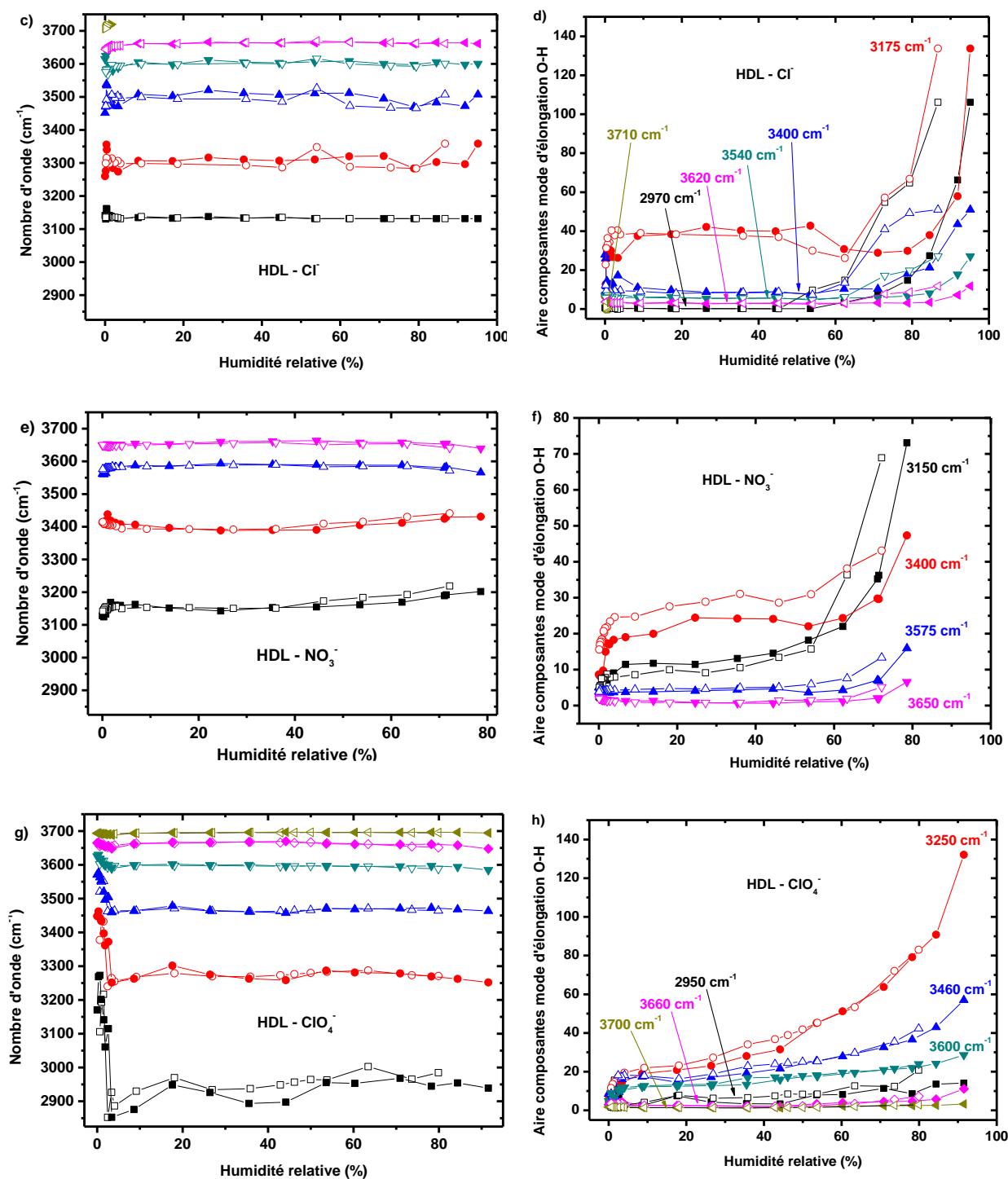
Figure V-31. Position et aire des bandes de décomposition du mode d'élongation O-H en fonction de l'humidité relative pour : (a) et (b) HDL - \text{CO}_3^{2-} , (c) et (d) HDL - \text{Cl}^- , (e) et (f) HDL - \text{NO}_3^- et (g) et (h) HDL - \text{ClO}_4^- . Sur la figure de droite, c'est la valeur stabilisée du nombre d'onde lors de l'adsorption qui est reportée. Les symboles pleins correspondent à l'adsorption et les symboles creux à la désorption
