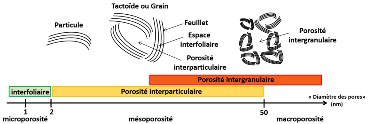
Figure I-10. Schéma de la structure des argiles à différentes échelles avec les différentes porosités créées ainsi que le classement des différentes porosités selon leur taille 8
