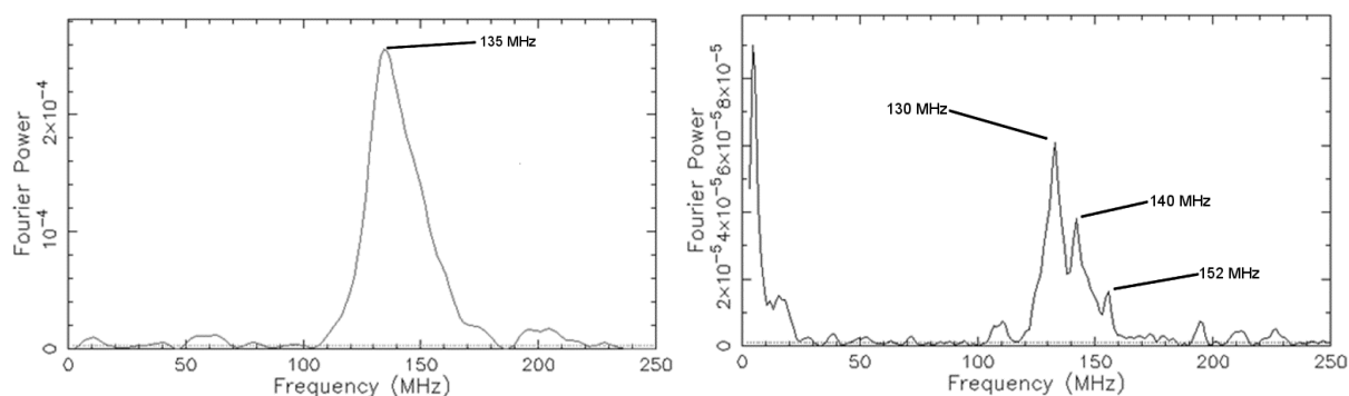
Figure III-39. Spectres de densité spectrale de puissance du talc synthétique placé dans un champ magnétique d'environ 100 G à 25 K (à gauche) et à 250 K (à droite)
