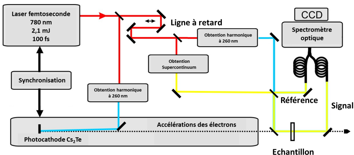
Figure II-8. Schéma de principe simplifié du fonctionnement du système pompe-sonde synchrone utilisé dans ELYSE
