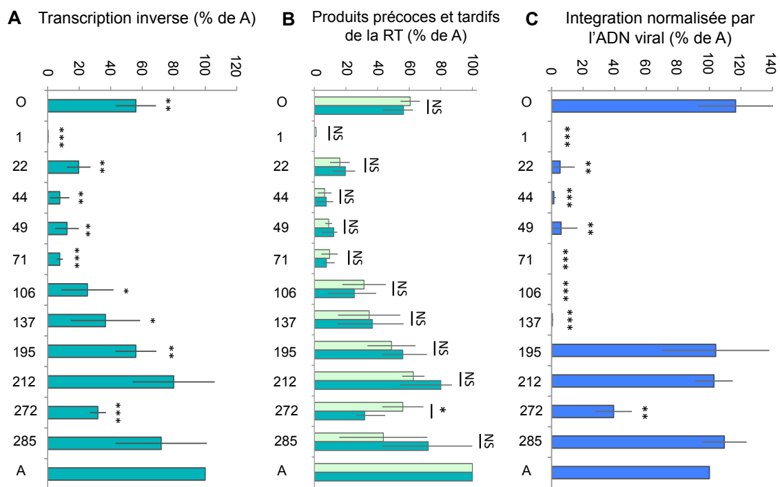
Figure 30 : Fonctionnalités des chimères AO. A. Efficacité de transcription inverse (quantité d'ADN viral tardif) comparé au parent A, fixé à 100%. Les étoiles reflètent la p valeur d'un test de Student à un échantillon comparé la valeur du parent (A=100%). B. Comparaison entre les quantités des produits précoces (en vert clair) et tardifs (en vert foncé) de la transcription inverse, exprimées en fonction du parent A, fixé à 100%. Un test de Student à deux échantillons indique si les moyennes sont statistiquement différentes pour chaque chimère C. Efficacité d'intégration (nombre de clones résistants à la puromycine) normalisée par la quantité totale d'ADN viral et exprimée par rapport au parent A, fixé à 100%. Les étoiles reflètent la p valeur d'un test de Student à un échantillon comparé à la valeur du parent (A=100%). Les expériences ont été répétées au moins 3 fois, les barres d'erreurs correspondent aux écart-types. (NS p > 0,05 ; * p < 0,05 ; ** p < 0,01 ; *** p < 0,0001 )
