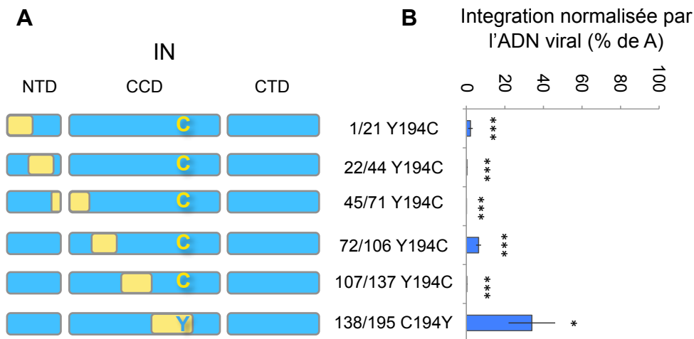
Figure 38 : Test de restauration du mutant Y194C. A. Schéma des IN chimères testées. Les positions des extrémités encadrant la région substituée par la séquence d'origine O sont indiquées à droite du schéma. L'acide aminé présent à la position 194 est indiqué, en bleu pour la tyrosine d'origine A et en jaune pour la cystéine d'origine O. B. Efficacité d'intégration normalisée par la quantité totale d'ADN viral et exprimée par rapport au parent A, fixé à 100%. Les étoiles reflètent la p valeur d'un test de Student à un échantillon comparé à A. Les expériences ont été répétées au moins 3 fois, les barres d'erreurs correspondent aux écart-types. (* p < 0,05 ; ** p < 0,01 ; *** p < 0,0001 )
