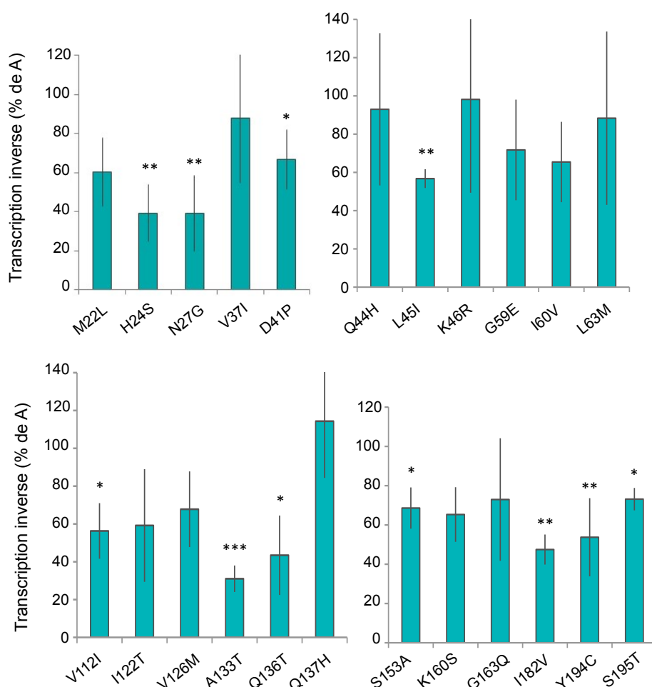
Figure 35 : Transcription inverse des virus portant les intégrases mutantes. Efficacité de transcription inverse (quantité d'ADN viral tardif) comparé au parent A, fixé à 100%. Les étoiles reflètent la p valeur d'un test de Student à un échantillon comparé à la valeur du parent A. Les expériences ont été répétées au moins 3 fois, les barres d'erreurs correspondent aux écart-types. (* p < 0,05 ; ** p < 0,01 ; *** p < 0,0001 )
