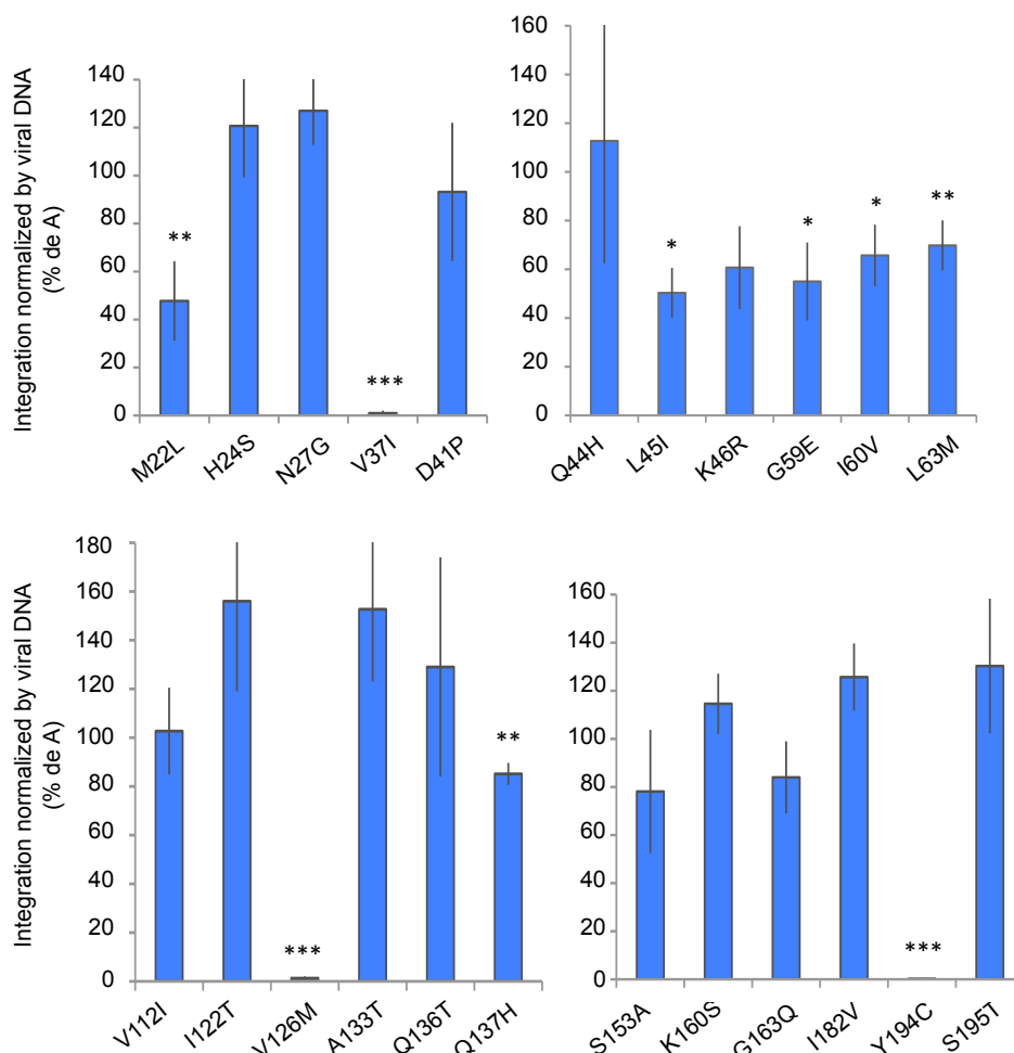
Figure 37 : Efficacité d'intégration des virus portant les intégrases mutantes. Efficacité d'intégration, normalisée par la quantité totale d'ADN viral et exprimée par rapport au parent A, fixé à 100%. Les étoiles reflètent la p valeur d'un test de Student à un échantillon comparé au parent A. Les expériences ont été répétées au moins 3 fois, les barres d'erreurs correspondent aux écart-types. (* p < 0,05 ; ** p < 0,01 ; *** p < 0,0001 )
