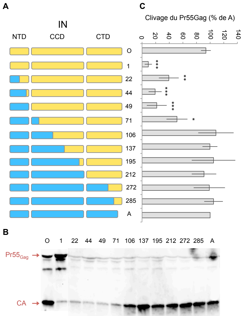
Figure 28 : Maturation des chimères AO. A. Schéma des onze intégrases chimères construites (1 à 285) ainsi que des deux parents O (en jaune) et A (en bleu). La position du point de recombinaison est indiquée à droite du schéma. B. Western blot avec un anticorps anti-capside. Les flèches rouges indiquent le précurseur Gag (Pr55Gag) et la capsid mature (CA). C. Taux de clivage du précurseur Gag correspondant au rapport entre la quantité relative de la CA mature et celle du précurseur Gag et des intermédiaires de clivage, détectée par Western blot (voir B). Les expériences ont été répétées au moins 3 fois, les barres d'erreurs correspondent aux écart-types. Les étoiles reflètent la p valeur d'un test de Student à un échantillon comparé à la valeur du parent (A=100%).
