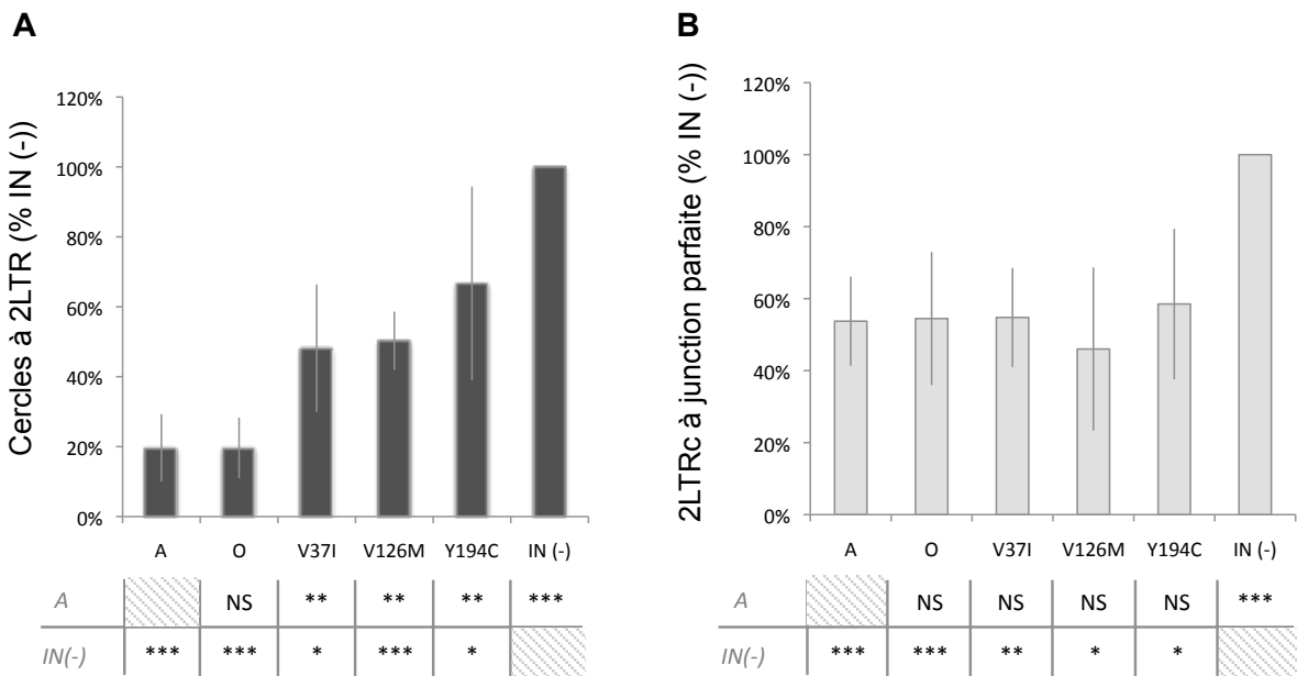
Figure 39 : Caractérisation fonctionnelle des mutants ponctuels. A. Quantités totales de cercles à 2LTRs détectées, exprimées par rapport à l'IN (-), fixé à 100. L'IN (-) est l'IN A dépourvue de son activité catalytique car mutée dans le site actif (mutation D116A). Le tableau en dessous du graphique contient les symboles qui reflètent la p valeur d'un test de Student comparé au parent A (ligne du haut) ou à l'IN(-) (ligne du bas). B. Rapports entre les quantités de cercles à 2LTRs à jonctions parfaites et les cercles à 2LTRs totaux, exprimés par rapport à l'IN (-), qui est fixée à 100 %. Le tableau en dessous du graphique contient les symboles qui reflètent la p valeur d'un test de Student comparé au parent A (ligne du haut) ou à l'IN(-) (ligne du bas). Les expériences ont été répétées au moins 3 fois, les barres d'erreurs correspondent aux écart-types. (NS p > 0,05 ; * p < 0,05 ; ** p < 0,01 ; *** p < 0,0001 )
