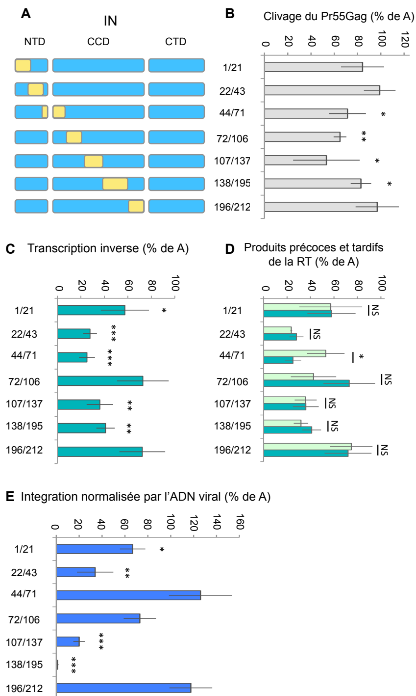
Figure 33 : Fonctionnalités des chimères AO. A. Schéma des intégrases testées, clonées en aval de la RT A. Les positions des extrémités encadrant la région substituée par la séquence d'origine O sont indiquées à droite du schéma. B. Taux de clivage du précurseur Gag détectée par Western blot. Les étoiles reflètent la p valeur d'un test de Student à un échantillon comparé à la valeur parentale (A=100%). C. Efficacité de transcription inverse (quantité d'ADN viral tardif) comparé au parent A, fixé à 100%. Les étoiles reflètent la p valeur d'un test de Student à un échantillon comparé à la valeur de A. D. Comparaison entre les quantités des produits précoces (en vert clair) et tardifs (en vert foncé) de la transcription inverse, exprimées en fonction du parent A, fixé à 100%. Un test de Student à deux échantillons indique si les moyennes sont statistiquement différentes pour chaque chimère. E. Efficacité d'intégration normalisée par la quantité totale d'ADN viral et exprimée par rapport au parent A, fixé à 100%. Les étoiles reflètent la p valeur d'un test de Student à un échantillon comparé au parent A. Les expériences ont été répétées au moins 3 fois, les barres d'erreurs correspondent aux écart-types.
