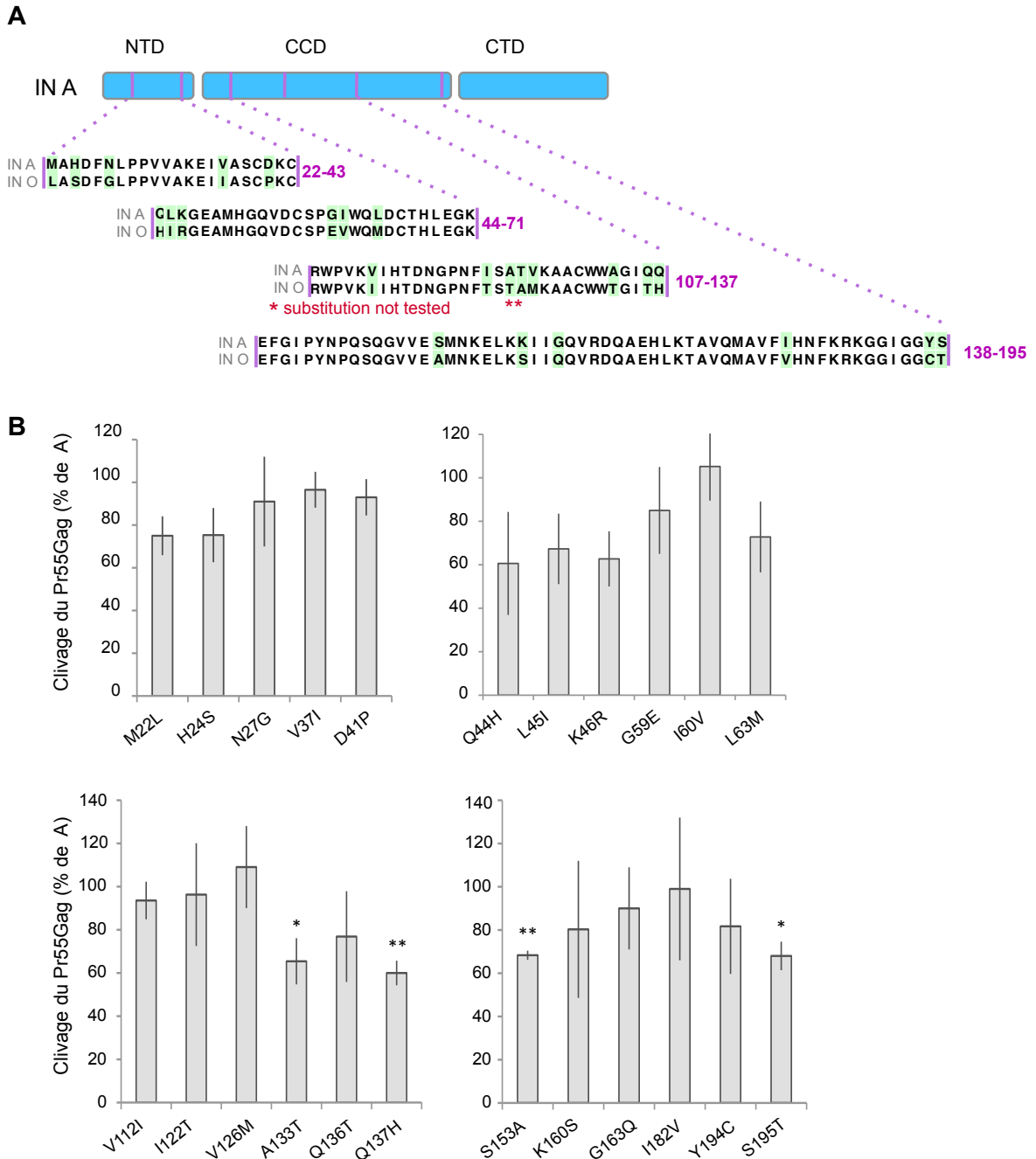
Figure 34 : Taux de clivage protéolytique du précurseur Gag des virus portant les intégrases mutantes. A. Schématisation des régions testées (en violet) sur l'IN parentale A (numérotation HXB2). L'alignement de la séquence de l'isolat A et O indique (en vert) les substitutions qui ont été testées individuellement. B. Taux de clivage du précurseur Gag déterminé par quantification des Western blot avec l'anticorps anti-CA. Les étoiles reflètent la p valeur d'un test de Student à un échantillon comparé à la valeur du parent (A=100%). Les expériences ont été répétées au moins 3 fois, les barres d'erreurs correspondent aux écart-types. (* p < 0,05 ; ** p < 0,01 ; *** p < 0,0001 )
