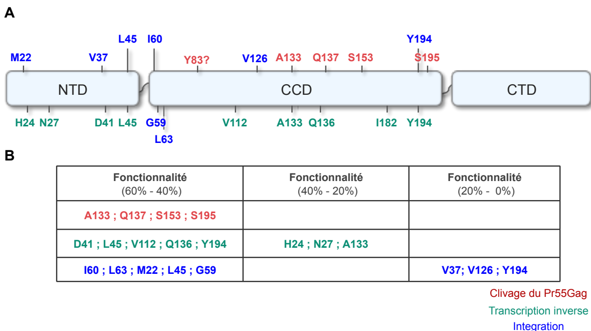
Figure 40 : Récapitulatif des résultats. A. Schéma des résidus non conservés de l'IN impliqués dans le maintien de sa fonctionnalité (maturation, en rouge ; transcription inverse, en vert ; intégration, en bleu). B. Tableau indiquant ces mêmes résidus classés par l'activité observée lorsqu'ils sont substitués par l'acide aminé de l'IN O.
