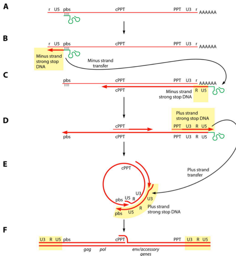
Figure 8 : Mécanisme de la transcription inverse. A. L'amorce ARN Lys,3 (en vert) s'hybride à sa séquence complémentaire sur l'ARN génomique viral (fine ligne rouge), le site de liaison de l'amorce (PBS). B. La synthèse du brin négatif d'ADN (épaisse ligne rouge) commence par l'ARNt et continue jusqu'à atteindre l'extrémité 5', générant le minus strand strong-stop DNA (-sssDNA). C. Après la dégradation du brin d'ARN hybridé à l'ADN par la RNaseH, le -sssDNA est libéré et peut s'hybrider sur la séquence complémentaire R à l'extrémité 3'. La synthèse du brin négatif d'ADN continue et l'ARN hybridé à l'ADN est dégradé en parallèle. D. Au fur et à mesure de la synthèse du brin négatif, la synthèse de l'ADN du brin positif est initiée à partir des séquences PPT, résistantes à la RNaseH. La synthèse à partir du PPT en 3' donne naissance au plus strand strong-stop DNA (+sssDNA). E. Après le clivage de l' ARN Lys,3 hybridé au PBS par la RNase H, le +sssDNA s'hybride sur la région PBS complémentaire du brin négatif, afin de permettre la synthèse complète des LTRs. F. La synthèse aboutit à un ADN bicaténaire avec un LTR à chaque extrémité, séparé par un court chevauchement appelé le flap central au niveau de la région PPT central (cPPT). Adapté de 182 .
