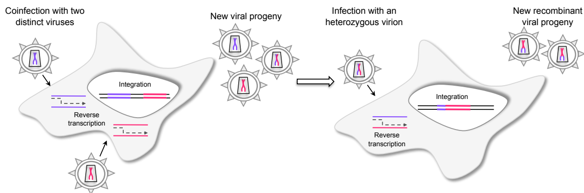
Figure 15 : Variabilité apportée par la recombinaison. La coinfection par deux virus différents (violet et rose) engendre la production d'une population virale hétérogène dont des virus dit hétérozygotes possèdent deux ARN encapsidés différents. Lors de l'infection d'une cellule par ce virus hétérozygote, le saut de brin lors de la transcription inverse génère un ADN recombinant, qui une fois intégré au génome cellulaire, amène à la production de virus recombinants. Adapté de 182 .
