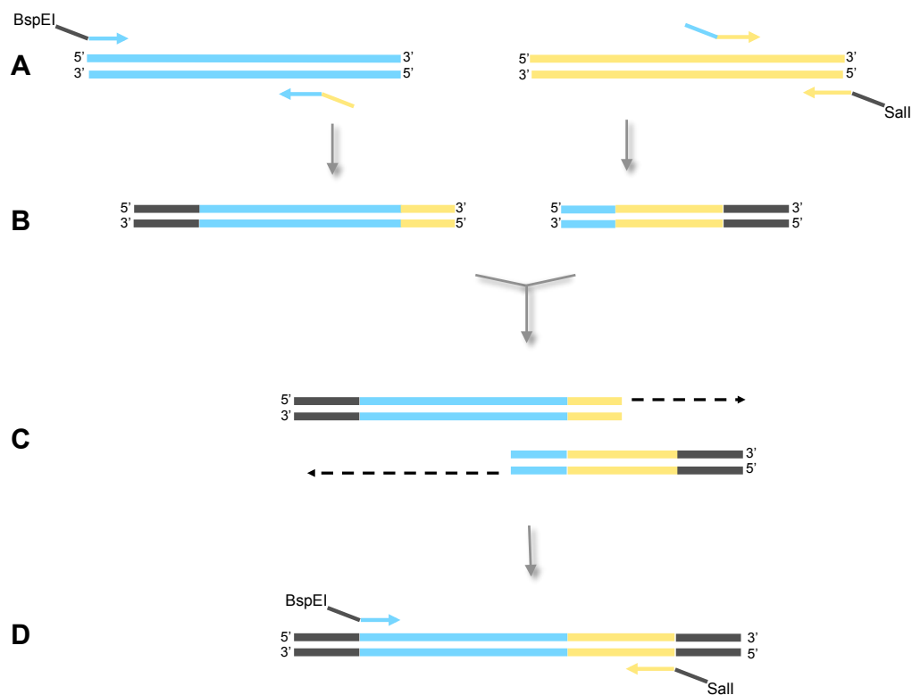
Figure 25 : Schématisation de la PCR reconstitutive. A. Les deux gènes parentaux sont indiqués en bleu et en jaune. Les amorces externes (aux extrémités du gène) sont composées en 5' des sites de restriction pour BspEI et Sall et en 3' des séquences complémentaires aux gènes parentaux. Les amorces internes (à l'intérieur du gène) sont complémentaires et s'hybrident au niveau du point de recombinaison entre les deux gènes. B. Les fragments 5' (à gauche) et 3' (à droite) qui permettent de reconstituer le gène chimère sont produits indépendamment par PCR. C. Les fragments 5' et 3' sont mélangés dans un mix réactionnel de PCR, ils s'hybrident par leurs extrémités complémentaires et subissent quelques cycles de PCR. La polymérase allonge les extrémités de chaque fragment afin de reconstituer le gène chimère. D. Le gène chimère est amplifié par PCR après ajout des amorces externes.
