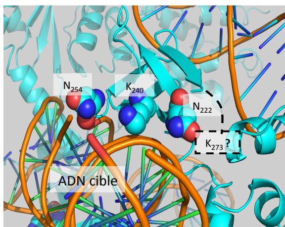
Figure 42 : Superposition des modèles obtenus par cryoélectromicroscopie du tétramère d'IN en complexe avec LEDGF et l'ADN viral et cellulaire des étapes de clivage des LTR et de transfert de brin. Les acides aminés visibles du motif ont été mis en évidence (N 222 , K 240 , N 254 ), la position présumée du K 273 est indiquée en pointillé. Adapté de 231 .
