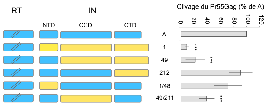
Figure 32 : Rôle du NTD et du CCD dans la maturation. Panneau gauche. Schéma des intégrases testées, clonées en aval de la RT A. Les positions du point de recombinaison ou des extrémités encadrant la région substituée par la séquence d'origine O sont indiquées à droite du schéma. Panneau droit. Taux de clivage du précurseur Gag correspondant au rapport entre la quantité relative de la CA mature et celle du précurseur Gag et de ses intermédiaires de clivage, détectées par Western blot. Les expériences ont été répétées au moins 3 fois, les barres d'erreurs correspondent aux écart-types. Les étoiles reflètent la p valeur d'un test de Student à un échantillon comparé à la valeur du parent (A=100%).
