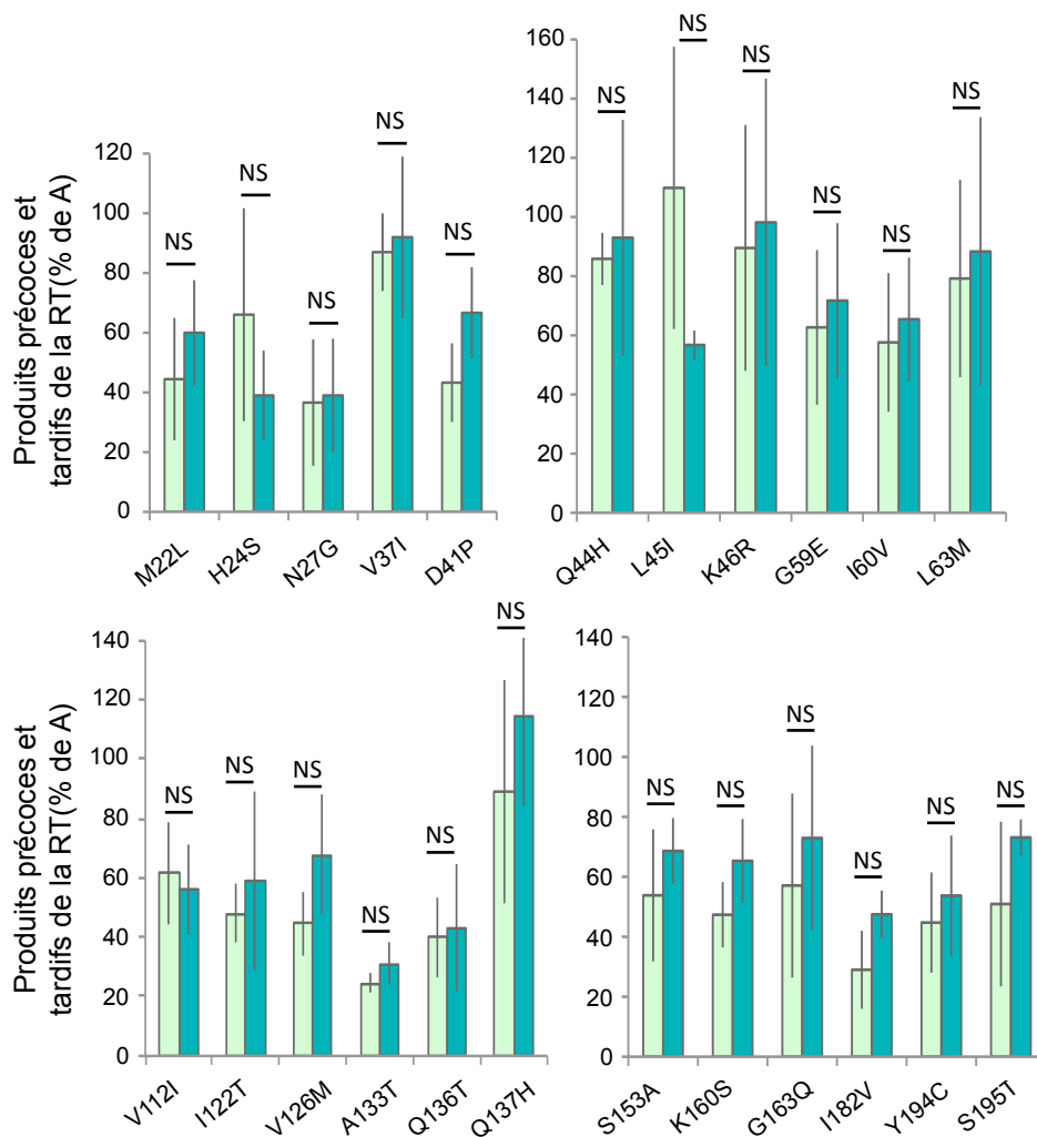
Figure 36: Produits de la transcription inverse. Comparaison entre les quantités des produits précoces (en vert clair) et tardifs (en vert foncé) de la transcription inverse, exprimées en fonction du parent A, fixé à 100%. Un test de Student à deux échantillons indique si les moyennes sont statistiquement différentes pour chaque chimère. Les expériences ont été répétées au moins 3 fois, les barres d'erreurs correspondent aux écart-types. (NS p > 0,05 ; * p < 0,05 ; ** p < 0,01 ; *** p < 0,0001 )
