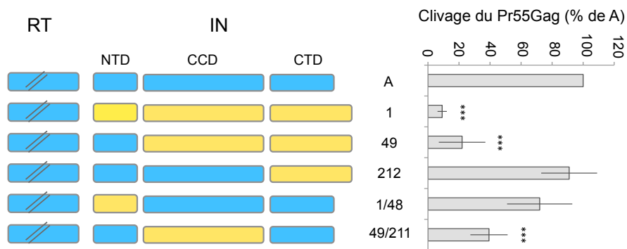
Figure 32 : Rôle du NTD et du CCD dans la maturation. Panneau gauche. Schéma des intégrases testées, clonées en aval de la RT A. Les positions du point de recombinaison ou des extrémités encadrant la région substituée par la séquence d'origine O sont indiquées à droite du schéma. Panneau droit. Taux de clivage du précurseur Gag correspondant au rapport entre la quantité relative de la CA mature et celle du précurseur Gag et de ses intermédiaires de clivage, détectées par Western blot. Les expériences ont été répétées au moins 3 fois, les barres d'erreurs correspondent aux écart-types. Les étoiles reflètent la p valeur d'un test de Student à un échantillon comparé à la valeur du parent (A=100%). (* p < 0,05 ; ** p < 0,01 ; *** p < 0,0001 )
