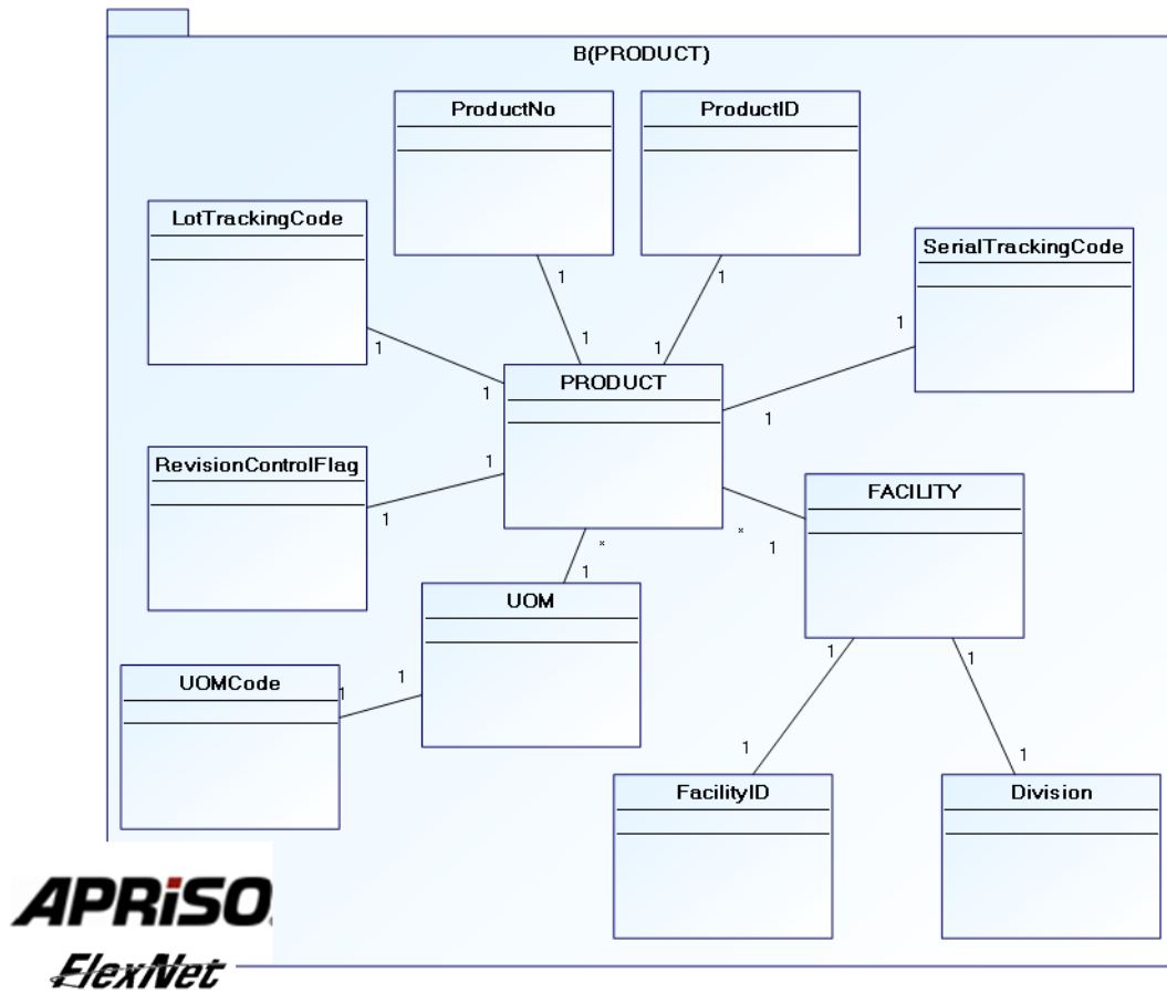
Figure 52. Le modèle conceptuel associé au bloc sémantique B(\text{PRODUCT})
