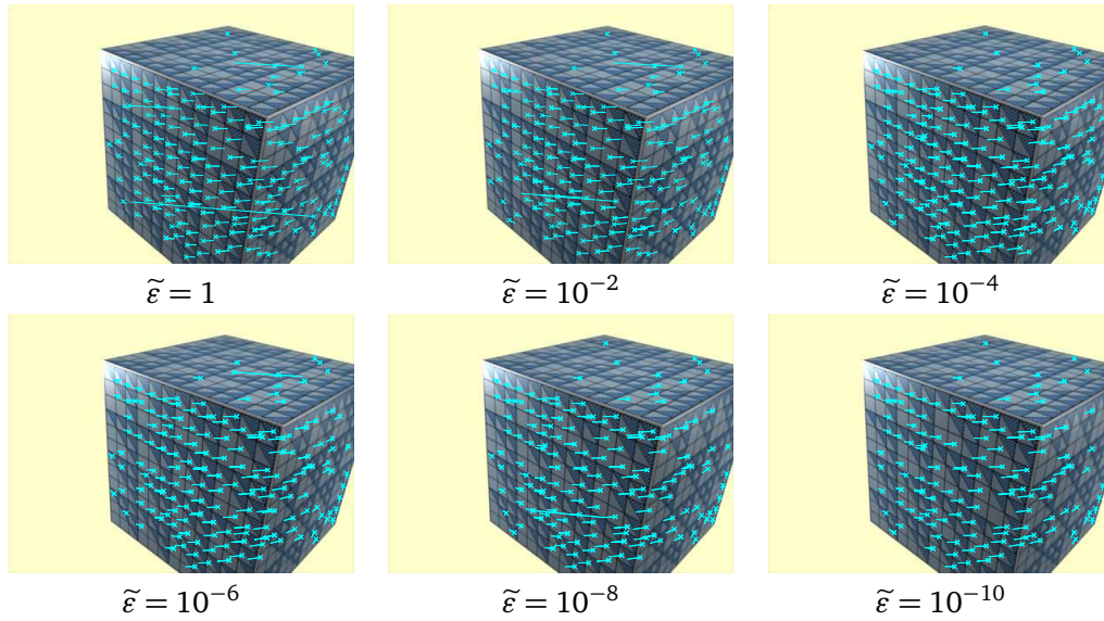
FIGURE 5.11 – Images Synthétiques. Dans cette expérience, nous recherchons le groupe le plus significatif compatible avec une matrice fondamentale entre deux vues, pour la distance CEMD-SUM, et six valeurs de \tilde{\epsilon} . Nous présentons ici uniquement les premières vues, les segments bleus correspondant au mouvement apparent d'un point d'intérêt (matérialisé par une croix) entre les deux vues. On constate que quelques appariements aberrants sont néanmoins sélectionnés. Un examen minutieux montre que ceux-ci sont situés le long des droites épipolaires qui leurs sont associées, et ne peuvent donc pas être détectés lors d'une mise en correspondance entre deux vues. Dans toutes les expériences (quels que soient la distance et \tilde{\epsilon} comme dans les tableaux 5.8 et 5.9), la distance moyenne d'un point à une droite épipolaire est environ de 0.2-0.3 pixel. 343 points d'intérêt SIFT ont été extraits de l'image 1, et 321 de l'image 2.
