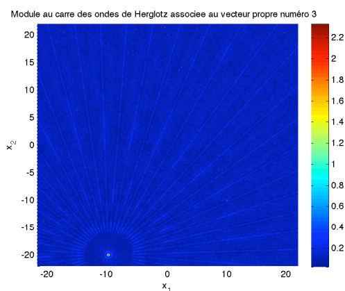
(c) Module de l'onde de Herglotz associée au troisième vecteur propre de \mathbb{T}
