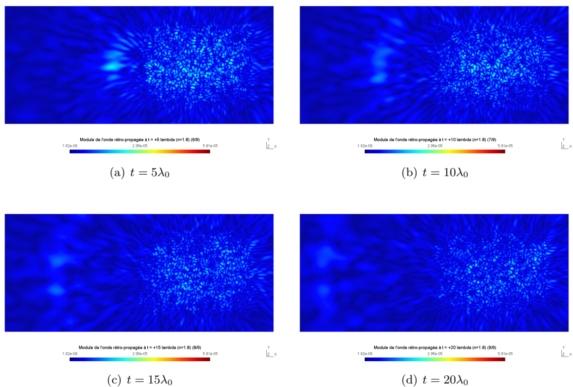
FIGURE 3.35 – Modulo de l'onde rétro-propagée par le MRT dans un milieu construit avec un contraste n = 1.8 . Les instants t sont ici positifs et correspondent à la propagation de l'onde après la focalisation sur le point source, présentée sur la figure 3.34.
