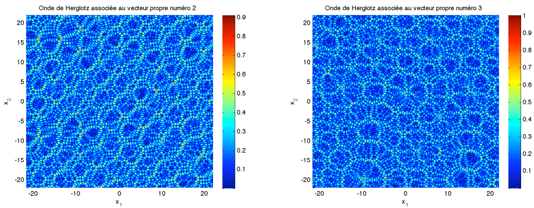
(c) Module de l'onde de Herglotz associée au deuxième vecteur propre de \mathbb{T}
