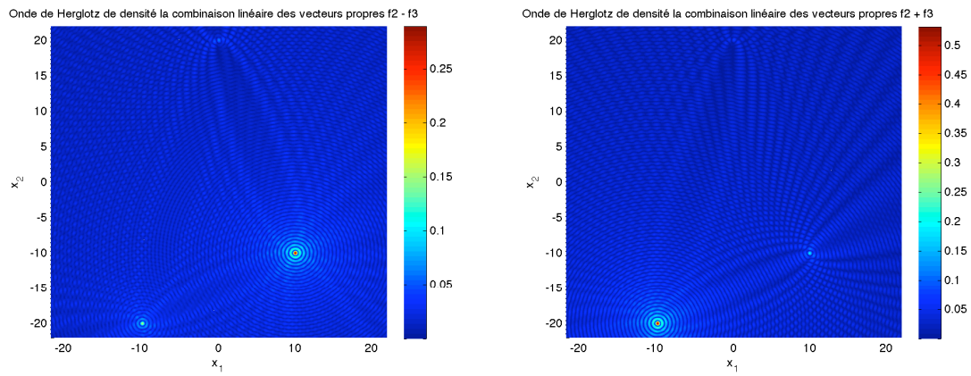
FIGURE 1.15 – Focalisation sélective sur les deux obstacles identiques, situés en (10, -10) et en (-10, -20) . Les ondes de Herglotz ont pour densité f_2 + f_3 (figure (a)) et f_2 - f_3 (figure (b)), où f_2 et f_3 sont deux vecteurs propres associés respectivement à la deuxième et la troisième plus grande valeur propre de \mathbb{T} .
