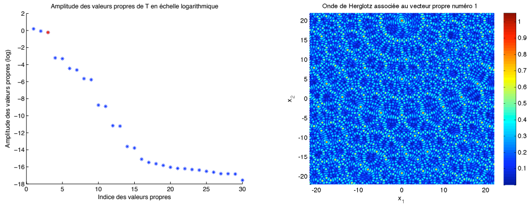
(a) Valeurs propres de \mathbb{T} (échelle logarithmique)
