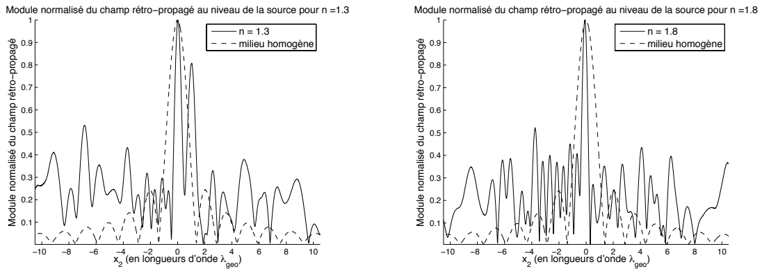
(a) n = 1.3 : présence de pics secondaires.
