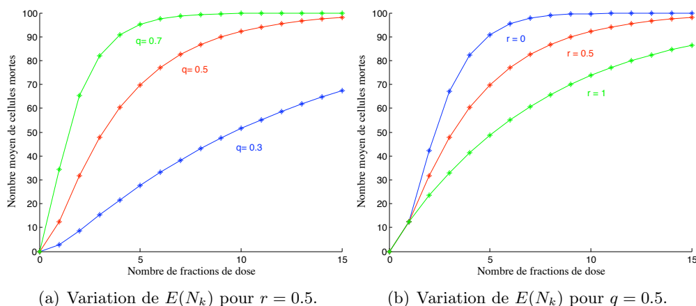
FIGURE 3.7 – Influence des paramètres q et r sur le nombre moyen de cellules mortes E(X_k(m)) , avec m = 3 et n_0 = 100 .
