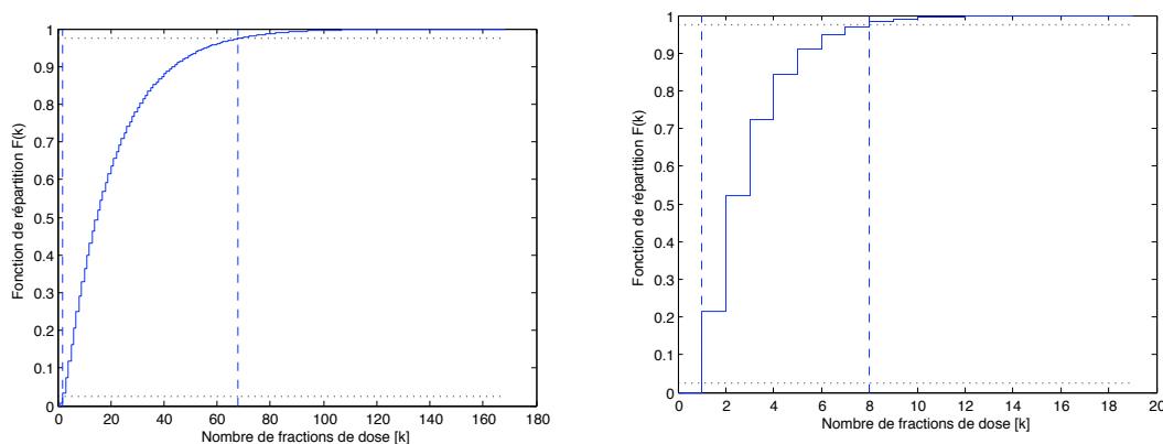
(a) La fonction de répartition F avec q = 0.2 . (b) La fonction de répartition F avec q = 0.6 .
