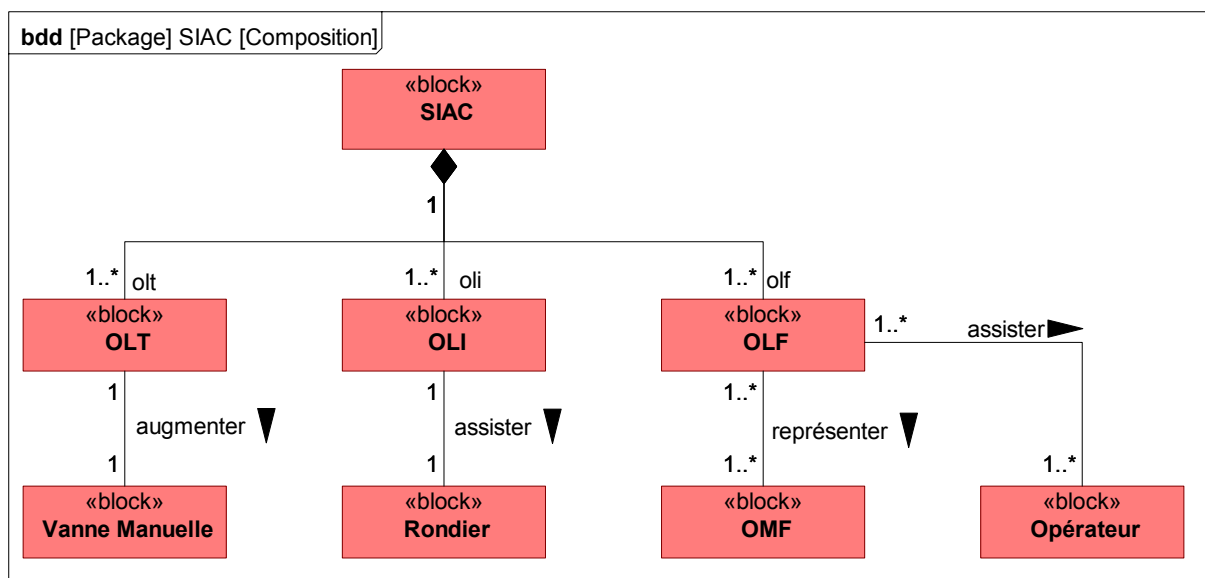
Figure 3.35 : Définition d'une structure hiérarchique par la composition du SIAC
