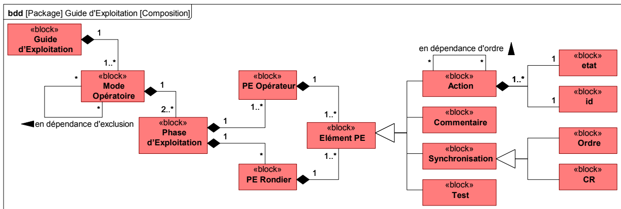
Figure 3.11 : Composition d'un Guide d'Exploitation
