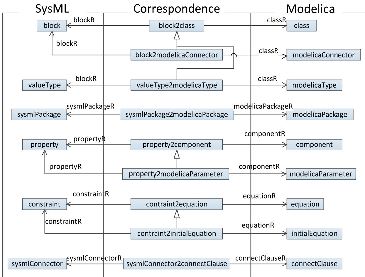
Figure 2.20 : Correspondance entre objets de modélisation SysML et Modelica (Johnson, 2008)
