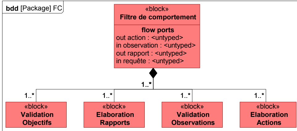
Figure 3.9 : Patron de conception pour le domaine de l'automatisation : le Filtre de Comportement
