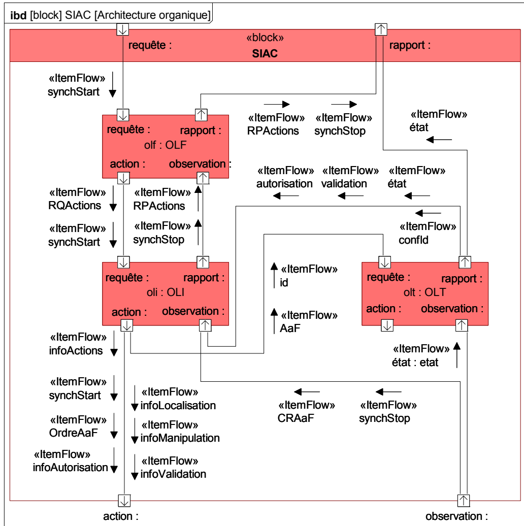
Figure 3.37 : Architecture organique du SIAC
