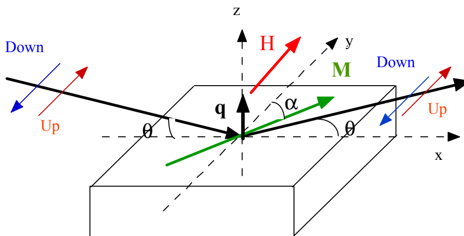
Figure III.9. Schéma de principe de la réflexion des neutrons polarisés sur un matériau magnétique possédant une aimantation uniforme faisant un angle \alpha avec la direction de polarisation des neutrons.
