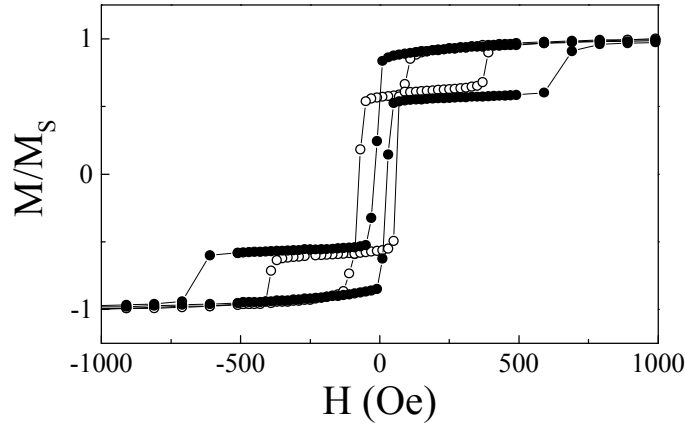
Figure III.55. Courbes d'aimantation en fonction du champ obtenue à 275K (symboles vides) et 225 K (symboles pleins) après refroidissement sous 7 T.
