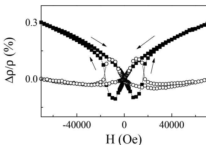
Figure II.29. Variation de la résistivité d'une couche de Tb_{12}Fe_{88} (50 nm) mesurée dans le cas où le champ est appliqué parallèlement (carrés pleins) ou perpendiculairement (carrés vides) au courant à 5 K. Les flèches indiquent le sens de lecture du premier cycle.
