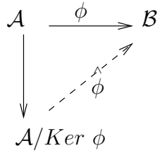
FIG. 1.6 – Factorisation d'un homomorphisme
