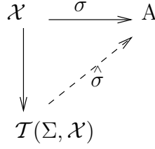
FIG. 1.4 – \Sigma -morphisme \hat{\sigma}
