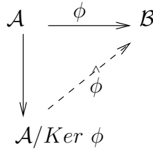
FIG. 1.6 – Factorisation d'un homomorphisme
