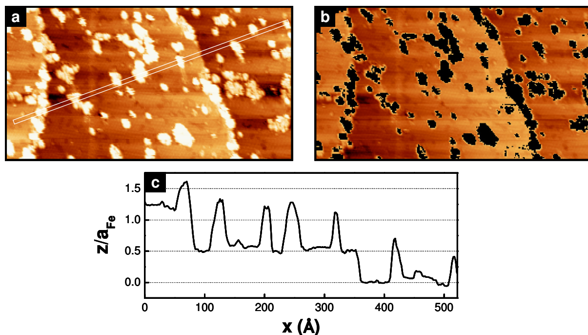
Fig. II-16 – (a) Image STM de la surface Fe/O(1.2 MC) ( 50 \times 27 \text{ nm}^2 ; tension pointe-surface : -500 mV ; courant : 1 nA ). (b) Traitement effectué pour déterminer le taux de recouvrement des îlots. (c) Distance pointe-surface le long du profil de la figure (a).
