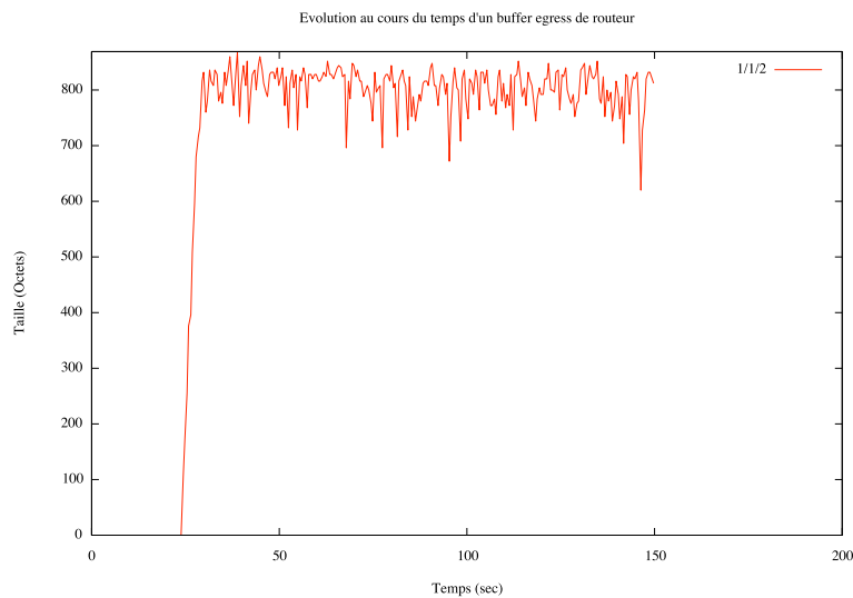
FIGURE 37: Evolution d'un buffer egress sur un port en coeur d'un routeur disposant d'une liaison congestionnée
