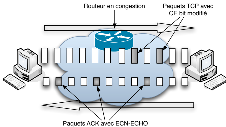
FIGURE 10: Principe du système ECN
