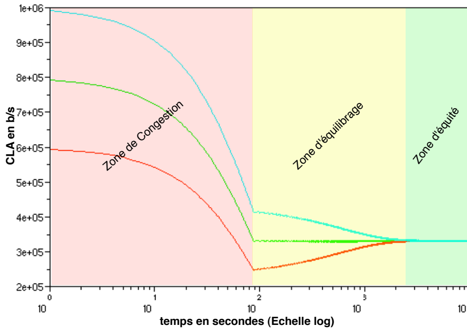
FIGURE 19: Système simple à base de DAR fractionnels
