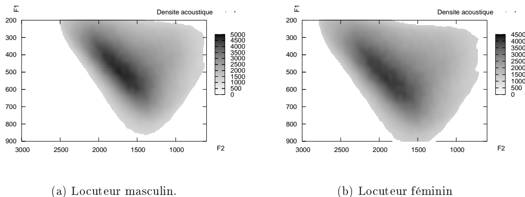
FIG. 3.2: Domaine acoustique pour un locuteur et une locutrice. L'abscisse correspond à F2 (Hertz), l'ordonnée à F1 (Hertz). La couleur indique la densité des images acoustiques, suivant une échelle linéaire.
