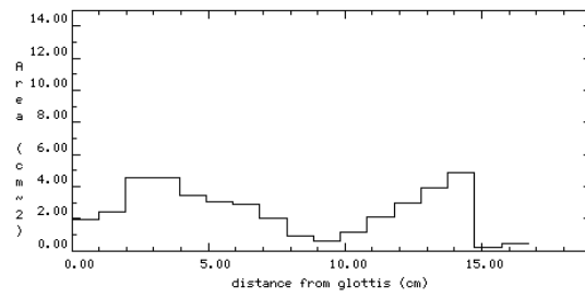
FIG. 6.6: Fonction d'aire pour un /u/ avec une constriction pharyngale.
