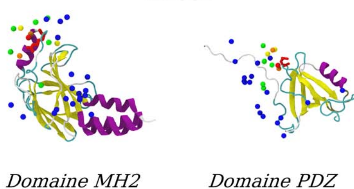
FIG. 2.20 – Graphique montrant la répartition du ligand par rapport au récepteur et inversement dans le cas où l'on donne R 279 en contact avec E 1321 comme information aux serveurs. Les sphères représentent les positions du résidu R 279 ou E 1321 pour chaque solution. Les sphères sont colorées en fonction de la distance R 279 -E 1321 : bleu pour une distance supérieure à 15 Å ; vert : pour une distance comprise entre 10 et 15 Å ; jaune : pour une distance comprise entre 7,5 et 10 Å ; orange : pour une distance comprise entre 5 et 7,5 Å et rouge : pour une distance inférieure à 5 Å. En rouge, le résidu R 279 au niveau de Smad3 et E 1321 au niveau d'Erbin.
