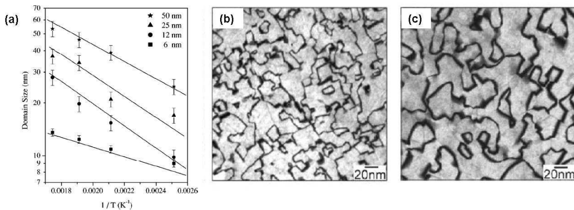
Figure 4.6 : (a) Taille des domaines en fonction de la température de dépôt et de l'épaisseur des couches de Fe 3 O 4 . Source [90]. (b) et (c) Images TEM en champ sombre obtenues à partir de la réflexion (220) d'une couche de, respectivement, 12 nm et 25 nm de Fe 3 O 4 sur MgO déposée à 250°C. Source [89].
