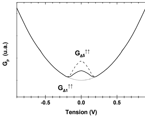
Figure 1.16 : Représentation schématique de la contribution des canaux \Delta_1^{\uparrow\uparrow} et \Delta_5^{\uparrow\uparrow} (courbes en pointillés) dans la conductance P (trait plein).
