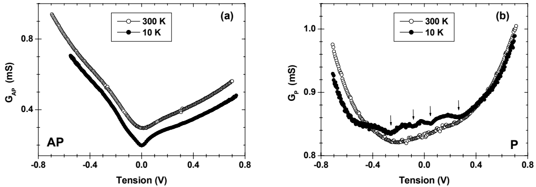
Figure 3.6 : Variation en tension des conductances dynamiques à 300 K et 10 K : (a) G_{AP} et (b) G_P . Les flèches indiquent la position des minima à |0.08| V et |0.25| V dans G_P .
