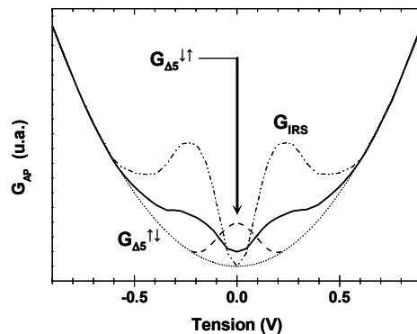
Figure 1.17 : Représentation schématique de la contribution des canaux \Delta_5^{\downarrow\uparrow} , \Delta_5^{\uparrow\downarrow} et \Delta_1^{IRS} (courbes en pointillés) dans la conductance AP (trait plein).
