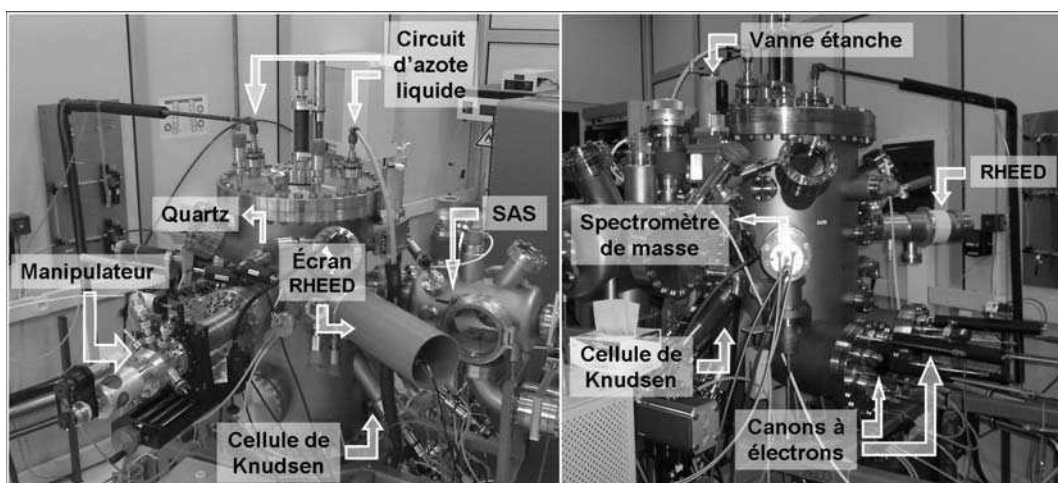
Figure A.1 : Photographies avant et arrière de la chambre d'épithaxie par jets moléculaires avec l'emplacement des différents éléments (cellules de Knudsen, canons à électrons, etc.)
