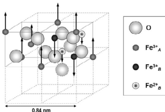
Figure 4.4 : Contribution magnétique des ions \text{Fe}^{2+} et \text{Fe}^{3+} dans la spinelle inverse \text{Fe}_3\text{O}_4 . Un fort couplage antiferromagnétique entre les cations \text{Fe}^{3+}_A et \text{Fe}^{3+}_B domine les interactions magnétiques complexes de \text{Fe}_3\text{O}_4 .
