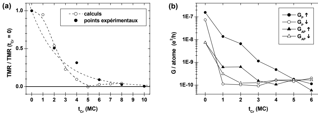
Figure 2.11 : (a) Variations expérimentale (cercles pleins) et calculée (cercles vides) de TMR normalisées en fonction de l'épaisseur de Cr(001). (b) Conductances calculées pour chaque canal de spins ( \uparrow , \downarrow ) et configuration magnétique (P ou AP) en fonction de l'épaisseur de Cr(001) (échelle logarithmique en ordonnée). Toutes les courbes sont des guides visuels.
