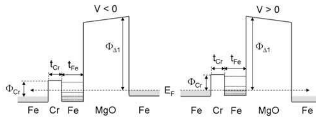
Figure 2.15 : Profils de potentiel perçus par les électrons \Delta_1^\uparrow en tension positive ( V > 0 ) et négative ( V < 0 ). Les niveaux de puits quantiques sont matérialisés par les traits discontinus horizontaux dans la couche de Fe(001) intermédiaire. Les flèches en pointillés indiquent le sens de parcours des électrons tunnel.
