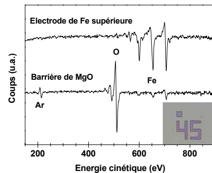
Figure A.3 : Suivi par spectroscopie Auger de la première étape de gravure ionique. En encart : image prise au microscope optique après l'étape de gravure. Les motifs de jonctions sont définis. Voir texte pour détails.
