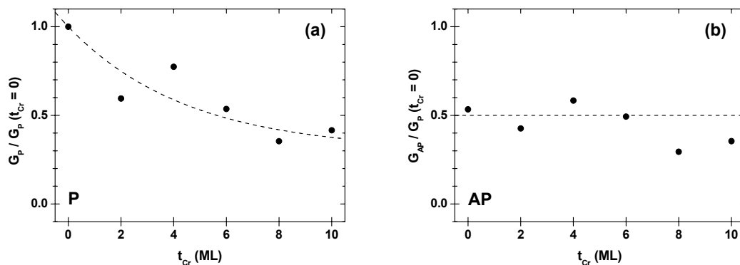
Figure 2.8 : Variation de G_P (a) et G_{AP} (b) en fonction de l'épaisseur de Cr(001) dans des JTMs épitaxiées Fe/Cr( t_{Cr} )/MgO/Fe(001) ; la courbe en pointillés en (a) est un guide visuel, en (b) la ligne en pointillés correspond à G_{AP} / G_P(t_{Cr} = 0) = 0.5 .
