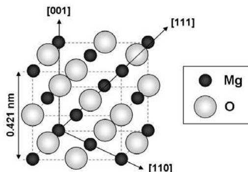
Figure 1.1 : Maille cubique du MgO et directions cristallographiques
