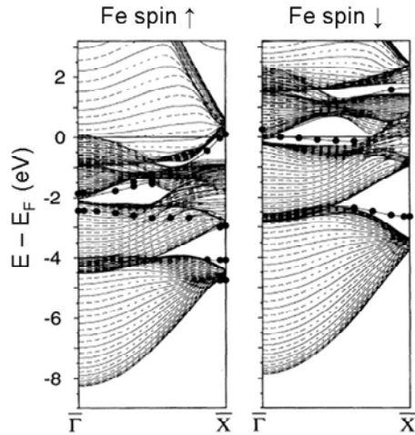
Figure 1.10 : Structure de bandes du bcc Fe(001) dans la direction \bar{\Gamma}-\bar{X} . Les parties grisées représentent le continuum des états du volume, les cercles noirs les états localisés en surface. D'après [28].
