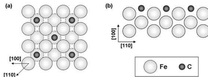
Figure 3.2 : Modèle structural de la reconstruction C(2x2) après ségrégation du C à la surface de Fe(001). (a) vue de dessus, (b) coupe transverse dans la direction [110].
