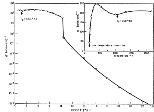
Figure 4.5 : Dépendance en température de la conductivité électrique de Fe_3O_4 . Source [75].
