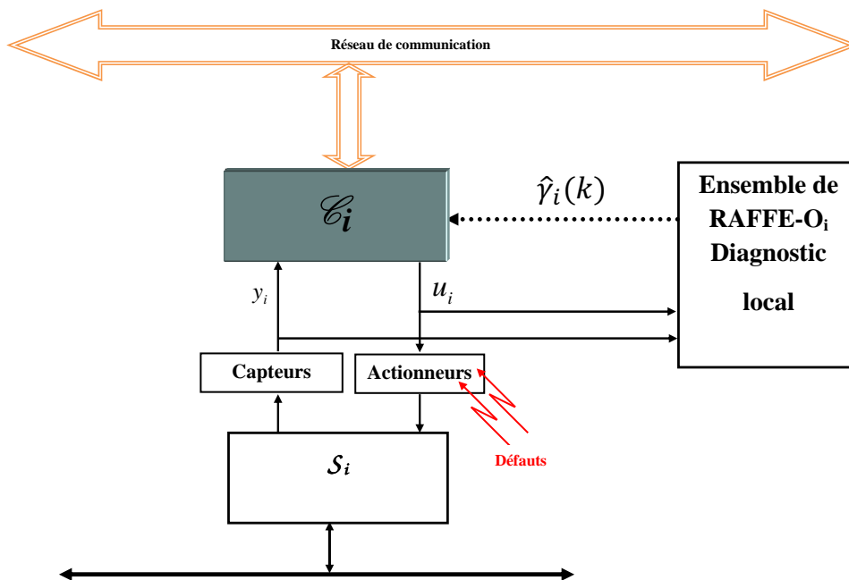
FIG. 4.9 – Diagramme interne d'un FTC/FDI local- défauts actionneurs.
