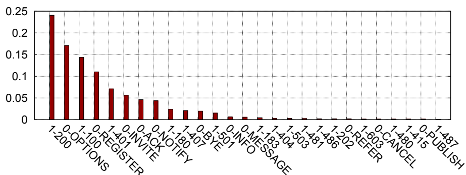
FIGURE 8.2 – Distribution empirique des messages SIP (le préfixe 0 indique une requête tandis que 1 préfixe les réponses)
