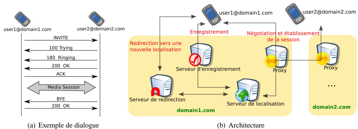
FIGURE 8.1 – Généralités sur SIP
