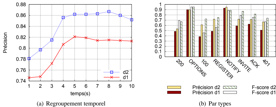
FIGURE 9.5 – Fingerpointing syntaxique non supervisé amélioré
