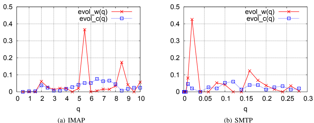
FIGURE 8.11 – SVC – Paramétrage automatique de q
