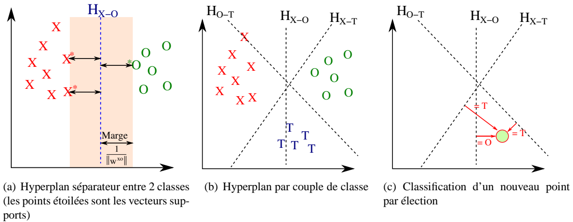
FIGURE 6.1 – Classification multi-classes avec les SVM
