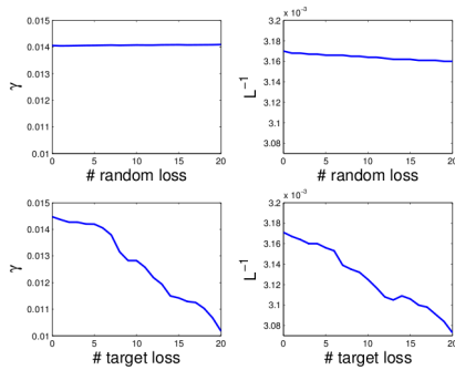
FIGURE 1.9 – Effet des défenses (aléatoire ou ciblée) dans un réseau P2P non structuré
