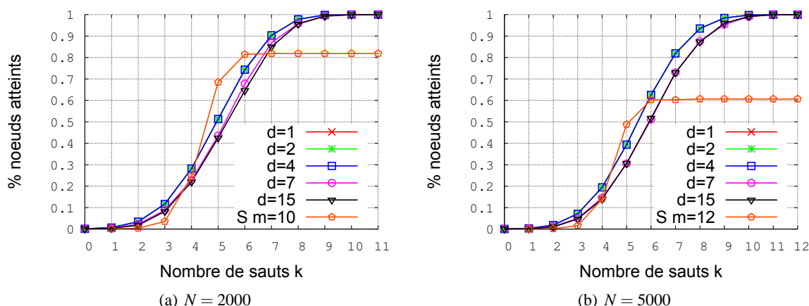
FIGURE 7.9 – Chord — Atteignabilité selon le nombre total de nœuds ( S = \text{Slapper} )
