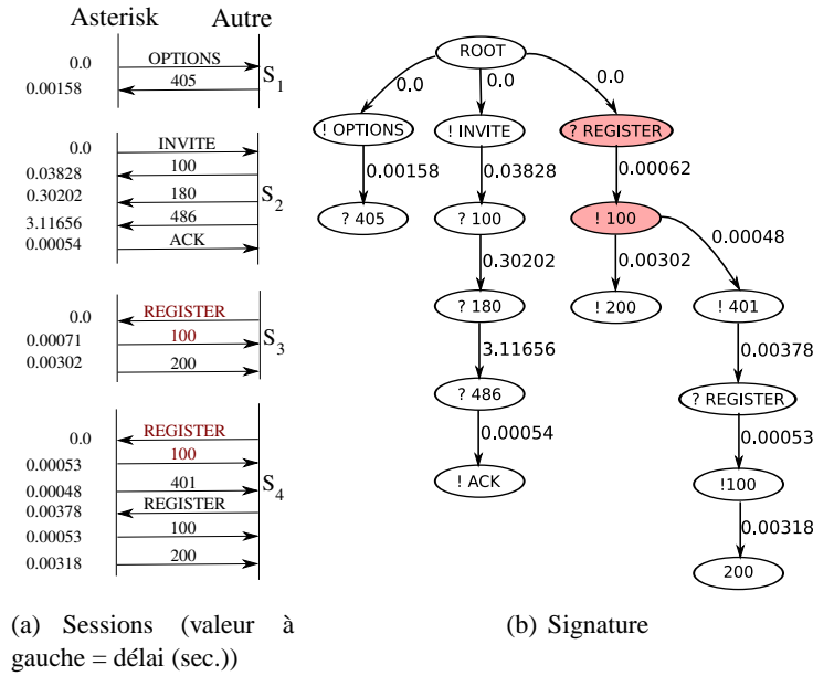
FIGURE 6.3 – Exemple de génération d’une signature pour un équipement de type Asterisk (SIP)
