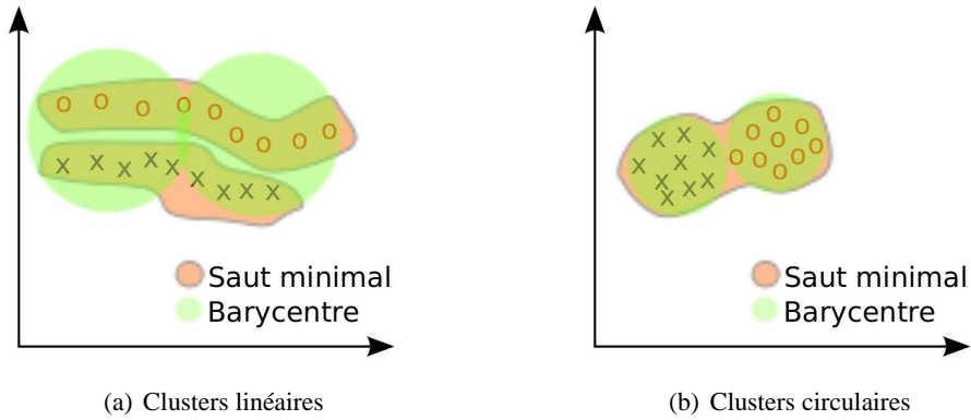
FIGURE A.2 – Clustering hiérarchique selon deux types de distances inter-clusters
