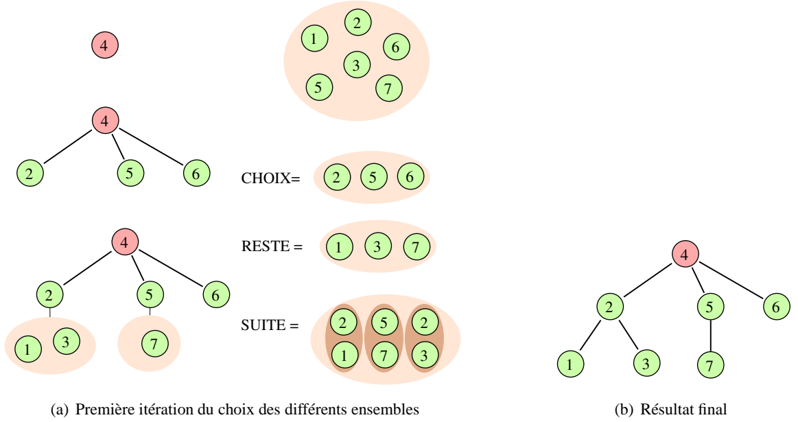
FIGURE 4.6 – Calcul des probabilités de distances minimales dans un arbre aléatoire
