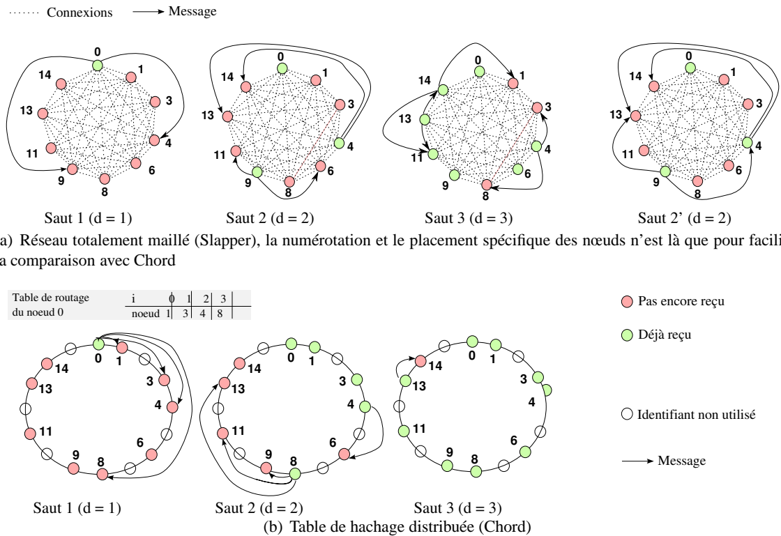
FIGURE 4.10 – Mécanisme de broadcast dans les réseaux P2P à partir du nœud 0
