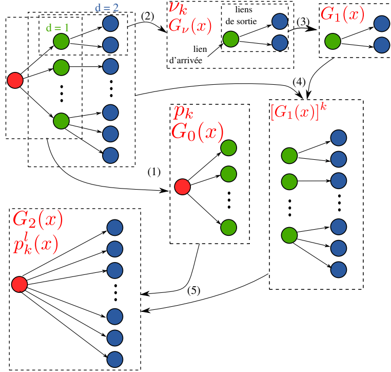
FIGURE 4.8 – Calcul du nombre de voisins au second saut pour le second modèle de botnets IRC
