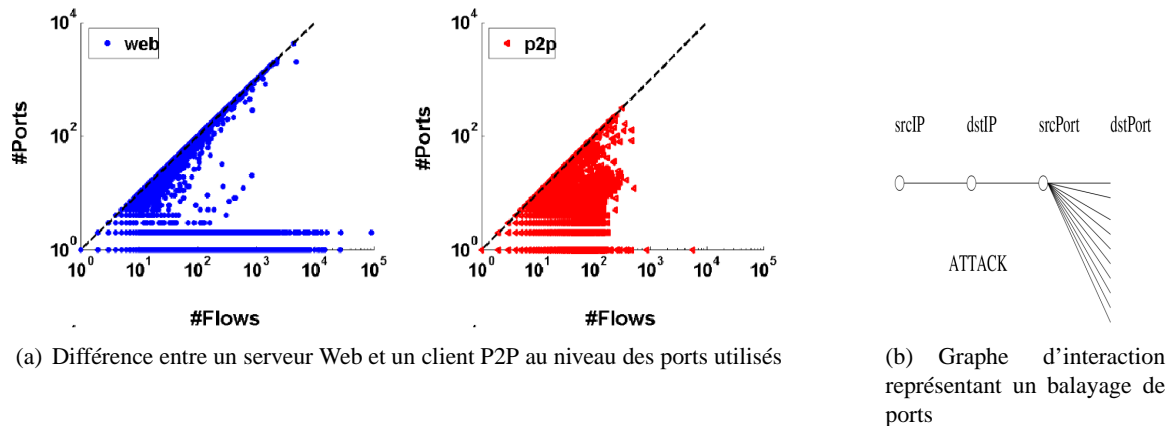
FIGURE 3.4 – Exemples de caractéristiques utilisées dans BLINC
