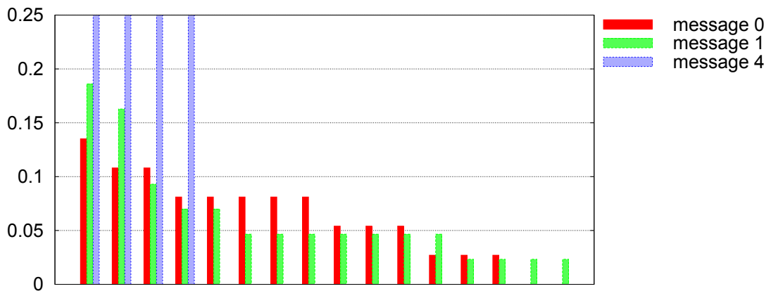
FIGURE 5.6 – Distribution ordonnée des caractères entre les messages chiffrés m_0 \oplus 'd' , m_1 \oplus 'f' et m_4 \oplus 'k'
