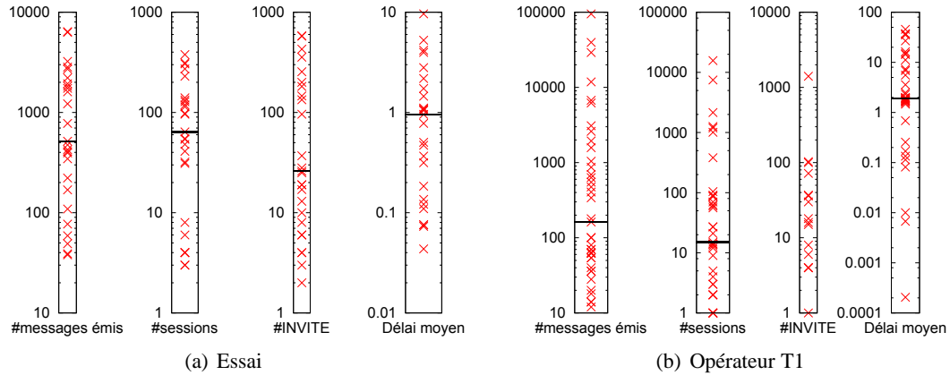
FIGURE 9.1 – Fingerprinting comportemental – Caractéristiques des jeux de données (échelle logarithmique, un point par type, valeur médiane représentée par une barre horizontale)
