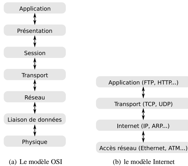
FIGURE 2.1 – Les différents modèles en couches
