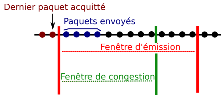
FIGURE 3.3 – Fenêtres TCP de l'émetteur
