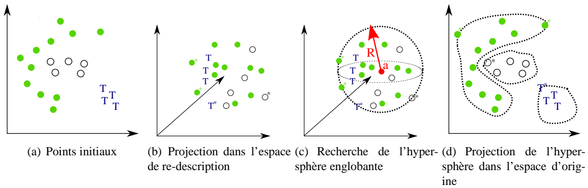
FIGURE A.3 – Les étapes de SVC (Les étoiles symbolisent les vecteurs supports)
