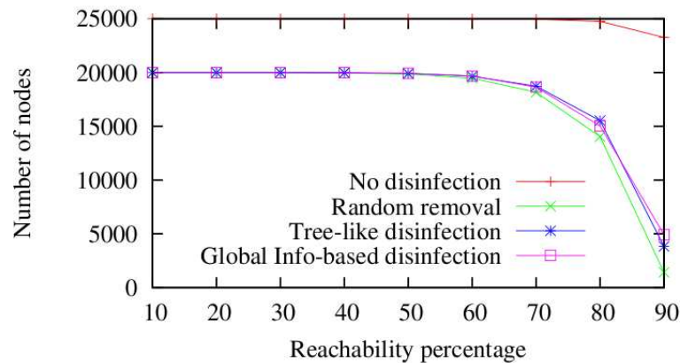
FIGURE 1.11 – Effets similaires des défenses (aléatoires ou ciblées) dans Overnet
