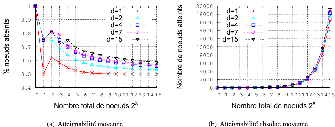
FIGURE 7.11 – Chord – Atteignabilité moyenne
