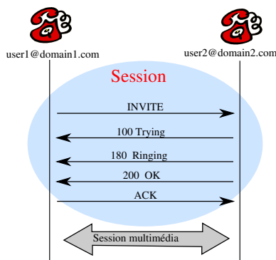
FIGURE 2.2 – Un exemple de session du protocole SIP
