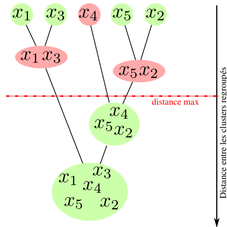
FIGURE A.1 – Partitionnement hiérarchique – les clusters en rouge sont les clusters finaux si une distance maximal représentée par la ligne rouge est spécifiée.
