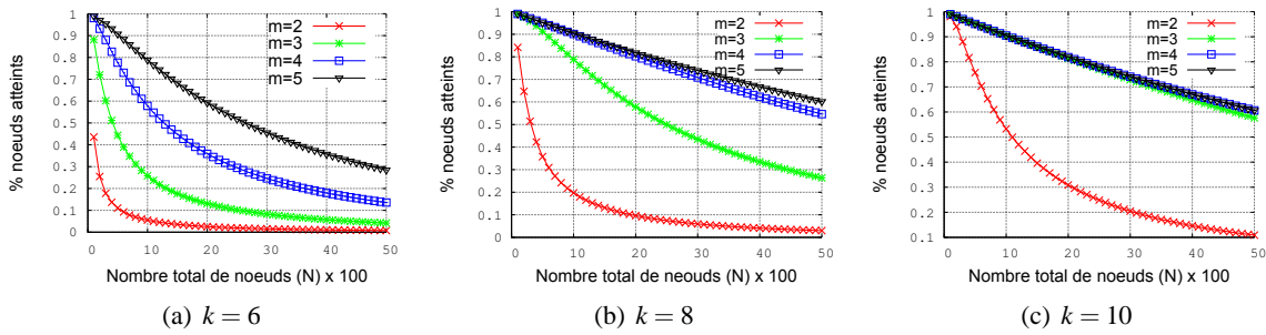
FIGURE 7.7 – Slapper — Influence du nombre de sauts k sur l'atteignabilité
