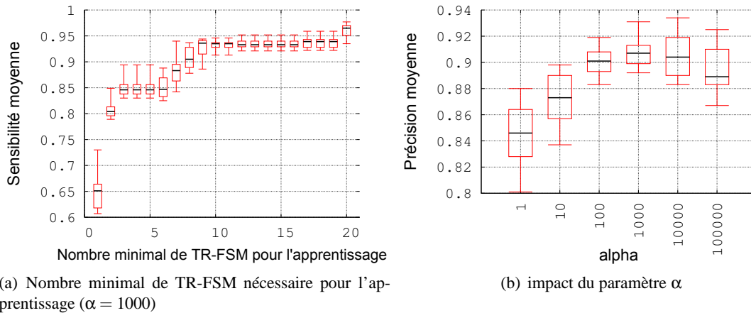
FIGURE 9.2 – Paramétrage du fingerprinting comportemental (taille de test = 10, taille d'apprentissage = 5)
