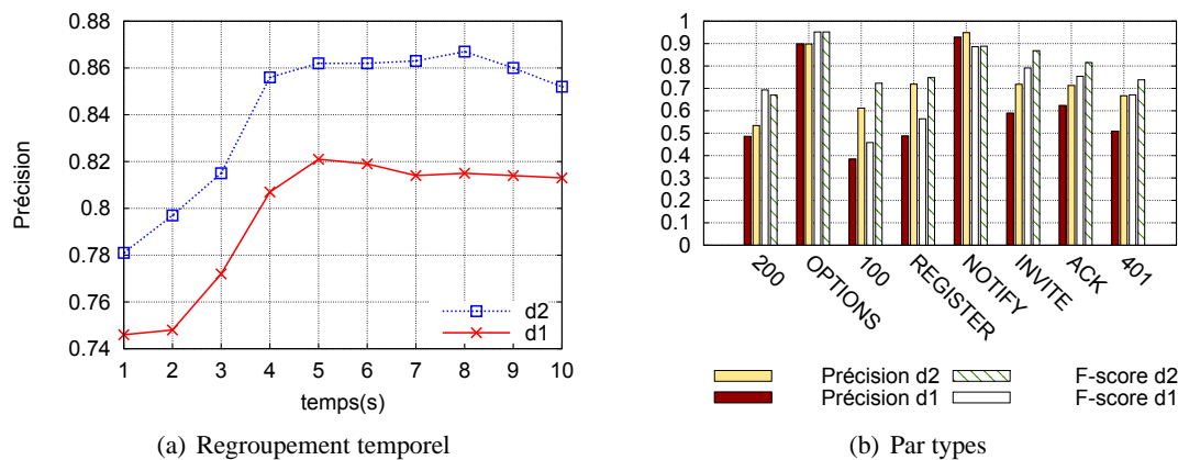
FIGURE 9.5 – Fingerpointing syntaxique non supervisé amélioré
