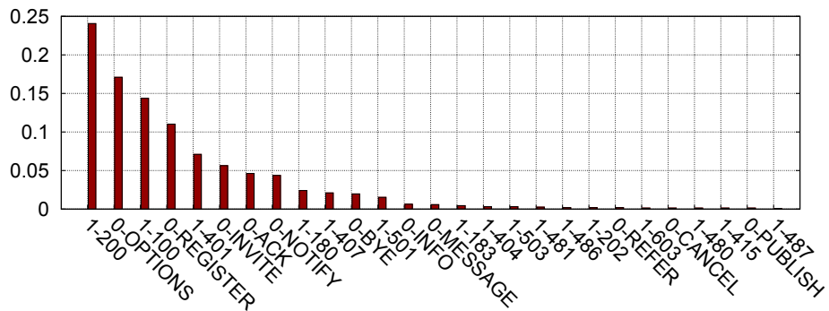
FIGURE 8.2 – Distribution empirique des message SIP (le préfixe 0 indique une requête tandis que 1 préfixe les réponses)
