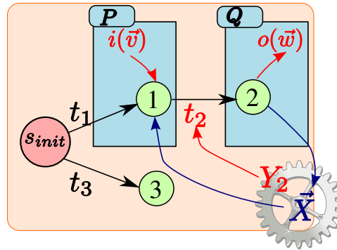
FIGURE 6.2 – Illustration d'un arbre TR-FSM
