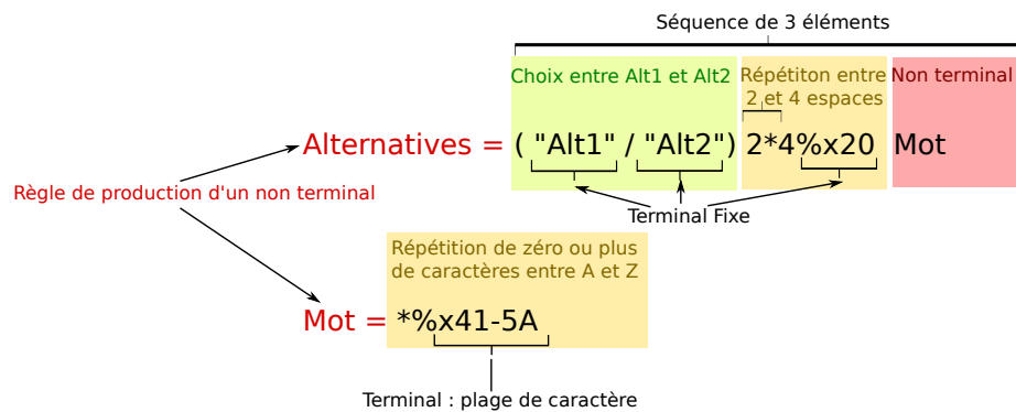
FIGURE 6.6 – Élément de définition d'une grammaire
