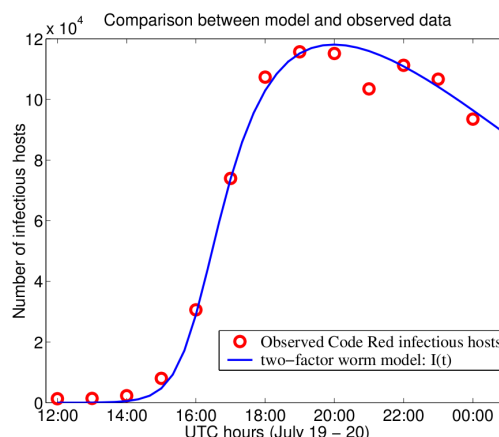
FIGURE 1.8 – Comparaison entre le modèle de [73] et le nombre réel de machines infectées par CodeRed
