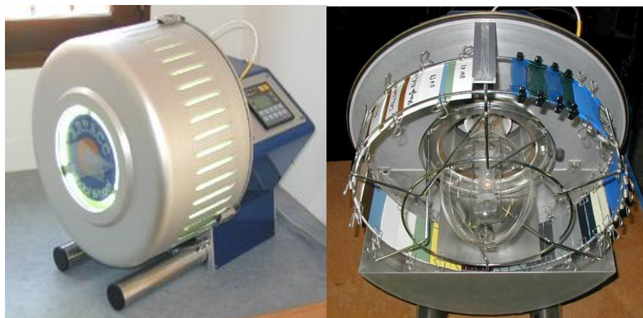
Figure 2-11: Enceinte de photo-vieillissement ARTACC® ( http://www.stationdebandol.com )
