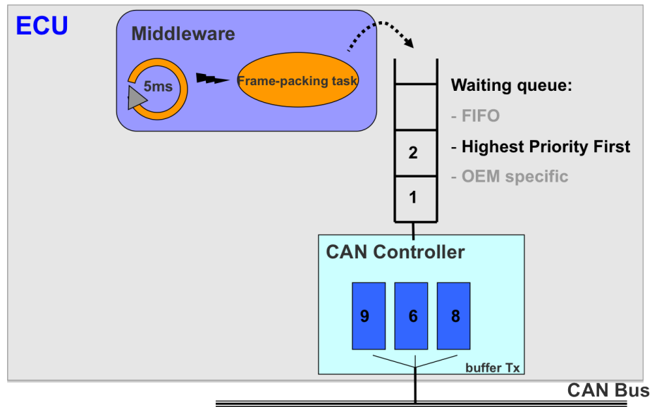
Figure 3.2 – Modèle simplifié de la pile de communication CAN [47]. Au niveau du logiciel middleware (AutoSar), une tâche périodique (de 5ms dans cet exemple) est responsable de la préparation des trames CAN à partir des données à transférer (les signaux). Une fois constituées, ces trames sont alors mises dans une file d'attente avant de pouvoir être copiées dans les buffers de transmission du contrôleur CAN qui est connecté au bus.
