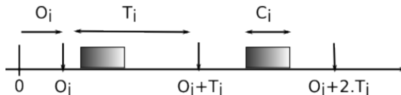
Figure 2.1 – Modèle des runnables. Après son arrivée, une instance d'un runnable doit avoir fini d'être exécutée avant l'arrivée de sa prochaine instance (c.à.d. l'échéance est égale à la période d'un runnable)
