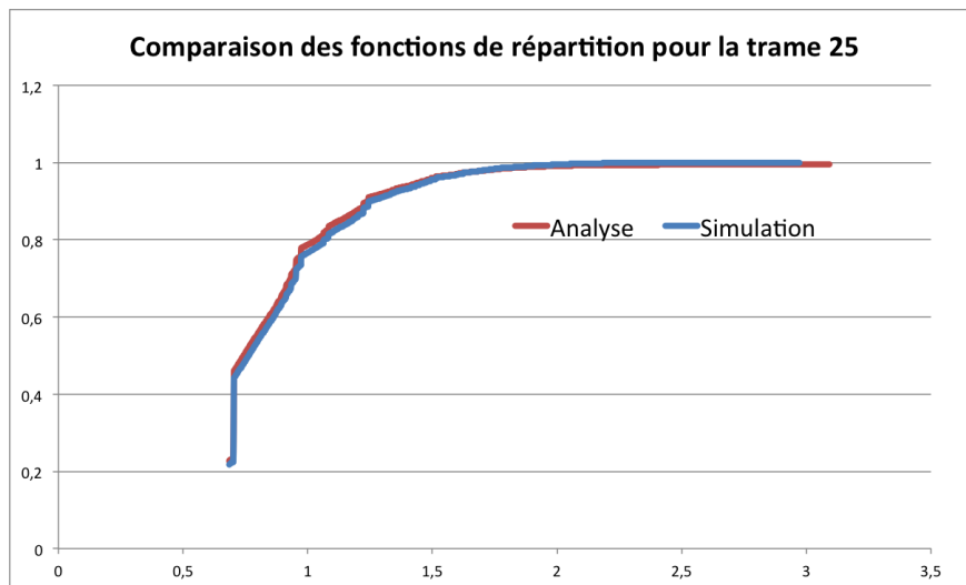
Figure 4.12 – Comparaison des fonctions de distributions pour la trame 25 (25 dans l'ordre de priorité sur 69) du benchmark issue de [64] obtenues par analyse (en rouge) et par simulation (en bleu). Les deux courbes sont très proches mais, comme prévu, nous constatons le même type d'écart avant la partie asymptotique de la courbe.
