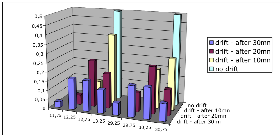
Figure 3.1 – Comparaison des distributions des temps de réponse observés pour une trame pour des simulations avec et sans dérive d’horloge [47]. Les différents couleurs correspondent aux différentes distributions. Les valeurs en abscisses sont les valeurs au centre des intervalles de temps de réponse.
