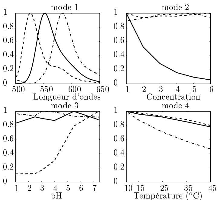
FIGURE 2.21 – Spectres d'émission de fluorescence mesurés ( \lambda de 500 à 650 nm) pour différents mélanges de colorants (Oregon Green 514 (OG514), Rhodamine 6G (R6G), Rhodamine B (RB)) et six différentes valeurs de températures (de 10^{\circ}\text{C} à 45^{\circ}\text{C} ) et six valeurs différentes de pH. Chaque graphique représente les spectres obtenus dans un même puits pour les 6 températures différentes.
