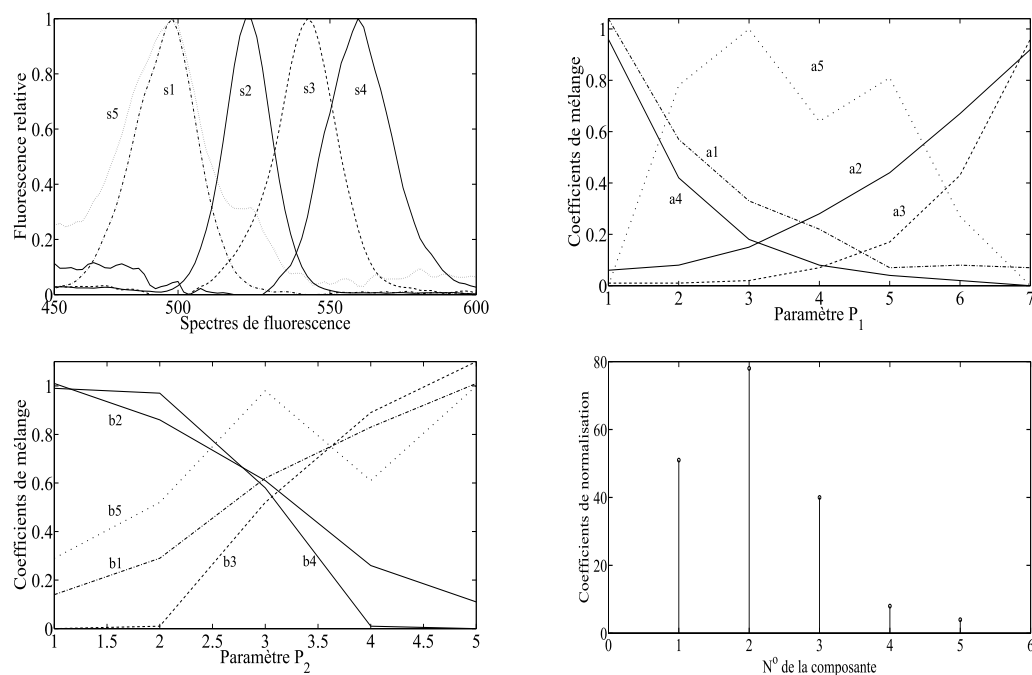
FIGURE 2.13 – Décomposition CP des données pour cinq sources. (a) Spectres de fluorescence. (b) Réponse en fonction du paramètre P_1 . (c) Réponse en fonction du paramètre P_2 . (d) Coefficients de normalisation obtenus par la mise à 1 de la valeur maximale de chaque réponse.
