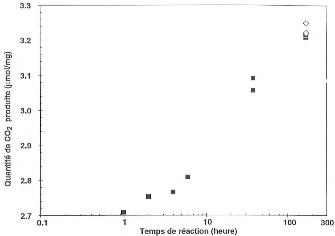
Figure II-21 : Evolution temporelle de la quantité de CO 2 produite par réaction de l'H 3 PO 4 sur des carbonates. Les symboles en noir correspondent à une réaction à 25°C alors que ceux en blanc ont été réalisés à 50°C.
