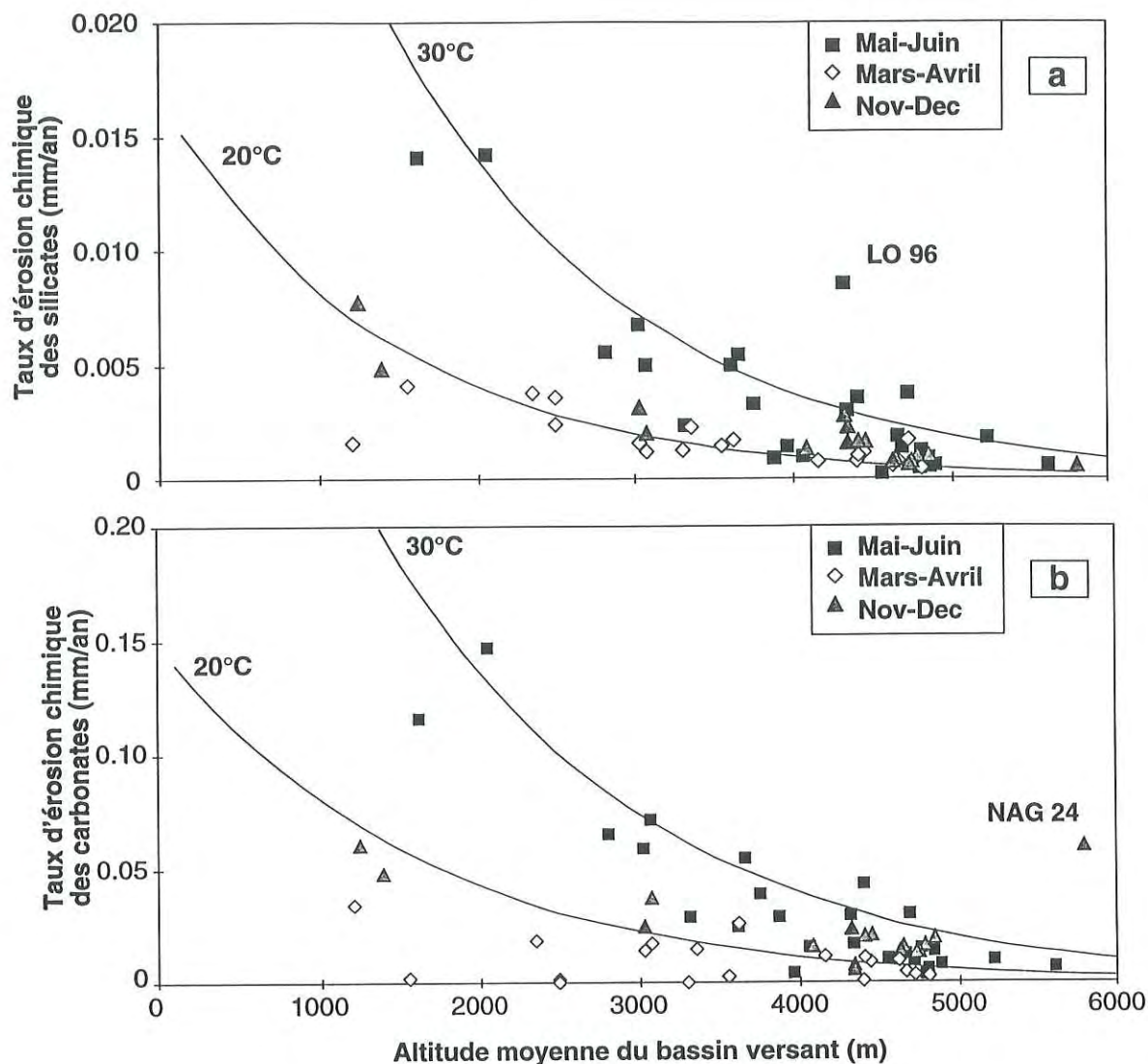
Figure IV-27 : Variation du taux de dénudation des silicates (a) et des carbonates (b) en fonction de l'altitude moyenne des bassins versants et de la saison. Les courbes modélisent une relation de type Arrhenius couplé à un gradient de température linéaire avec l'altitude.
