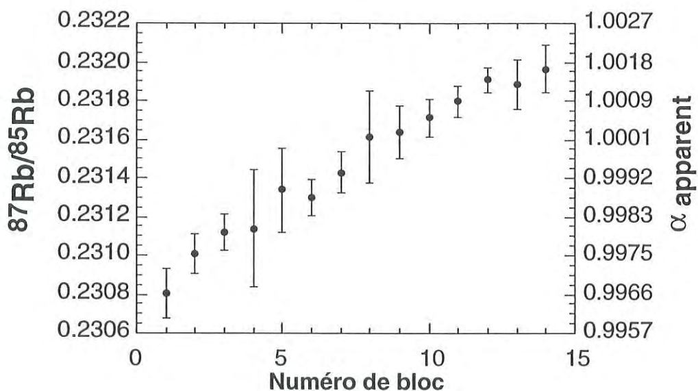
Figure II-1 : Evolution du rapport ^{87}\text{Rb}/^{85}\text{Rb} d'un échantillon spiké au cours d'une analyse.
