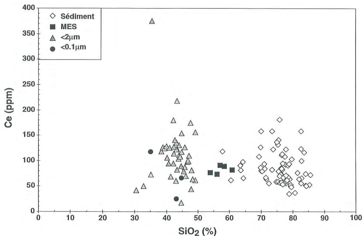
Figure V-10 : Teneur en Ce en fonction de la teneur en \text{SiO}_2 . La teneur en \text{SiO}_2 est celle des silicates, alors que la teneur en Ce est obtenue sur le sédiment total. La variation de la teneur en Ce pour une composition en \text{SiO}_2 donnée est de plus de 100%, ce qui ne peut pas résulter d'un quelconque effet de dilution sur le Ce par les carbonates.
