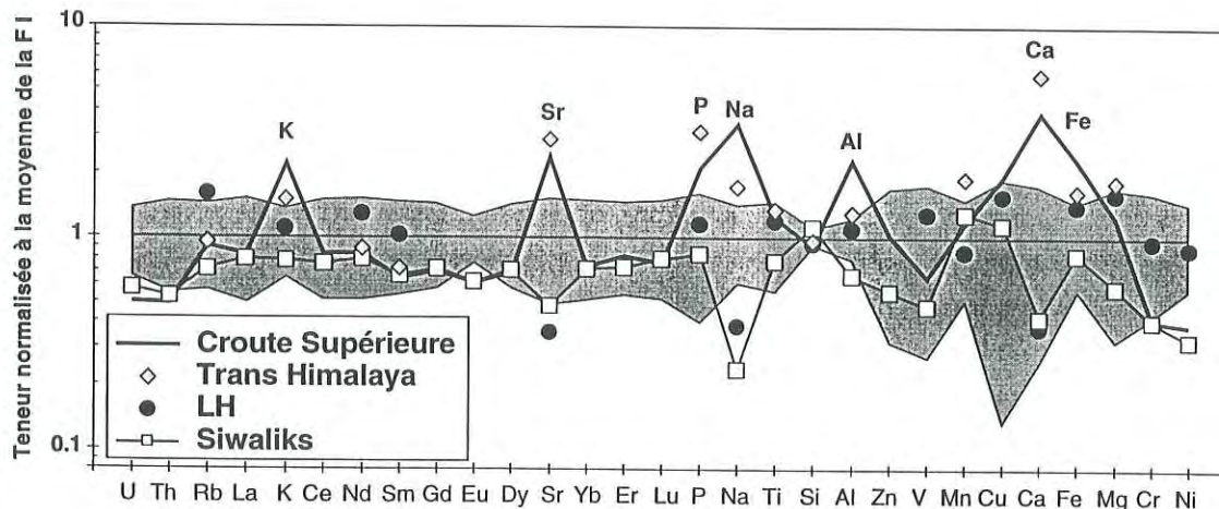
Figure III-5 : composition chimique moyenne des silicates himalayens normalisés à la composition moyenne de la Formation I de la HHC. La bande grisée représente la variabilité de cette formation.
