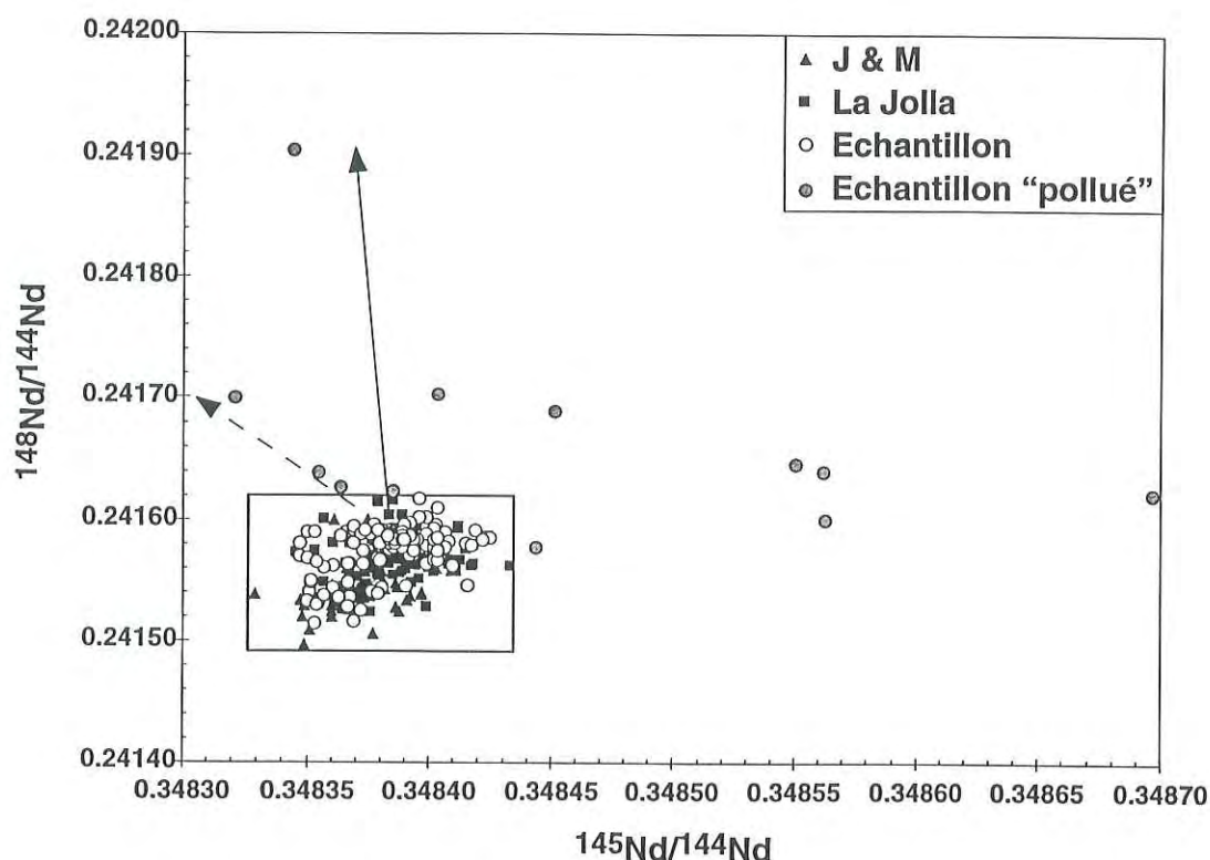
Figure II-16 : Co-variation des rapports ^{145}\text{Nd}/^{144}\text{Nd} et ^{148}\text{Nd}/^{144}\text{Nd} pour les standards et les échantillons. Les mesures notées « polluées » ont été rejetées. Le rectangle correspond à l'ensemble des compositions mesurées des standards. La flèche en pointillé indique une pollution sur la masse 144 et celle en trait plein simule une pollution en Sm.
