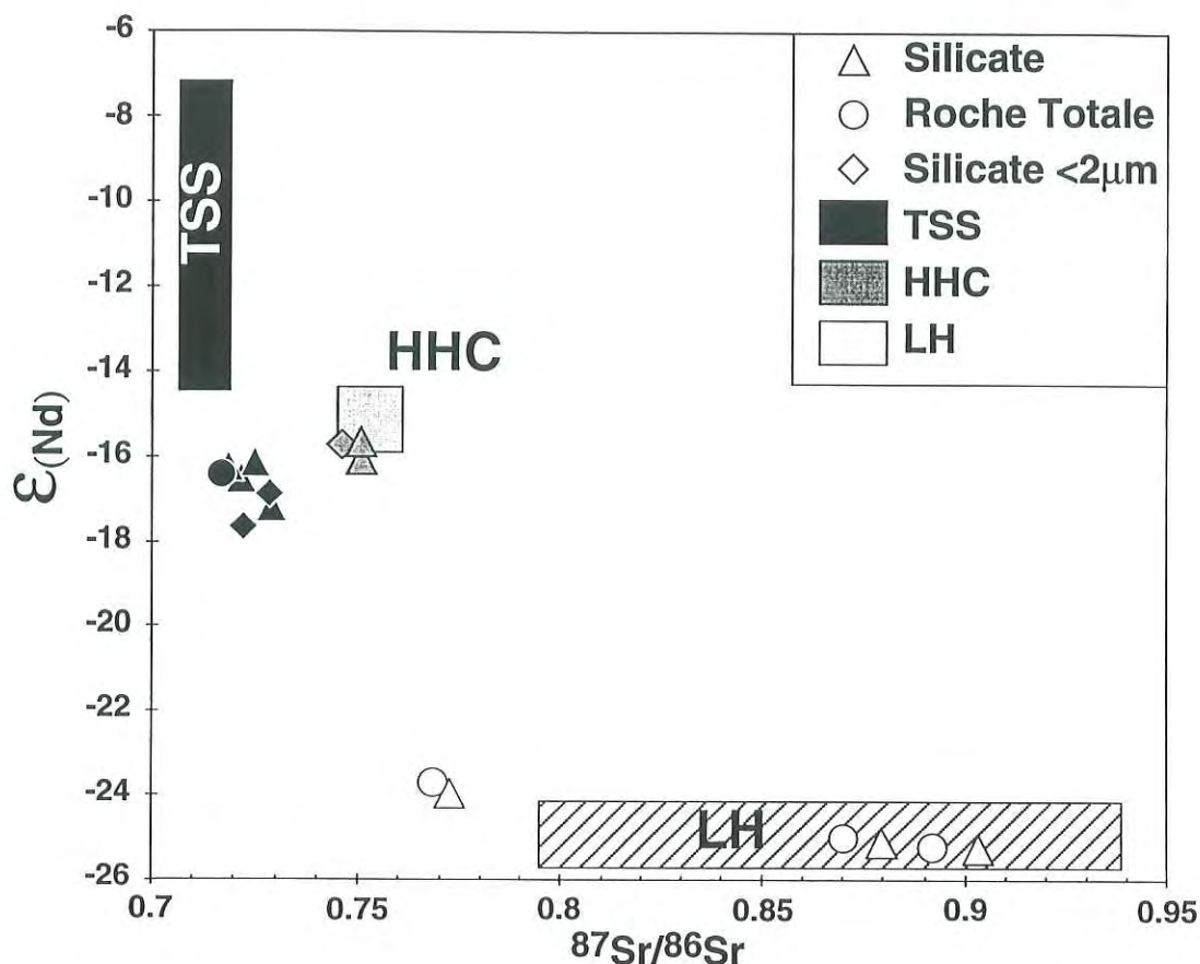
Figure V-14 : Compositions isotopique du Nd en fonction du rapport ^{87}\text{Sr}/^{86}\text{Sr} des sédiments de rivières ne drainant qu'une seule formation himalayenne (NAG 25, 33 et HF 10 ont été considérés comme tel). Les compositions moyennes des 3 principales formations sont aussi représentées (voir Chapitre III).
