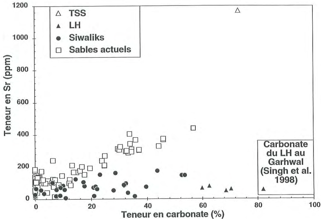
Figure III-15 : Teneur en Sr des carbonates des formations himalayennes (LH, TSS, Siwaliks) et des sables de rivières.
