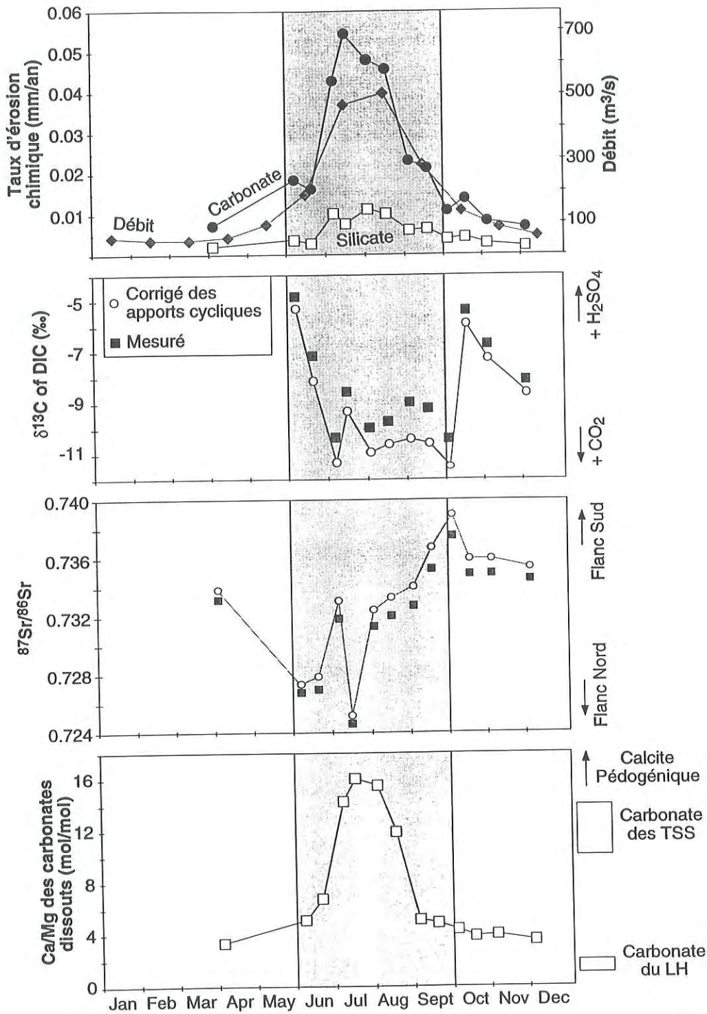
Figure IV-24 : Évolution mensuelle de l'érosion chimique pour le bassin versant de la Trisuli à Betrawati. Le \delta^{13}\text{C}_{\text{DIC}} indique le type d'acide altérant les roches (voir paragraphe IV-1), le ^{87}\text{Sr}/^{86}\text{Sr} est fonction de la région source des éléments dissouts (voir paragraphe IV-3), et le Ca/Mg des carbonates dépend de la mise en solution totale ou de la reprécipitation partielle sous forme de calcite pédogénique.
