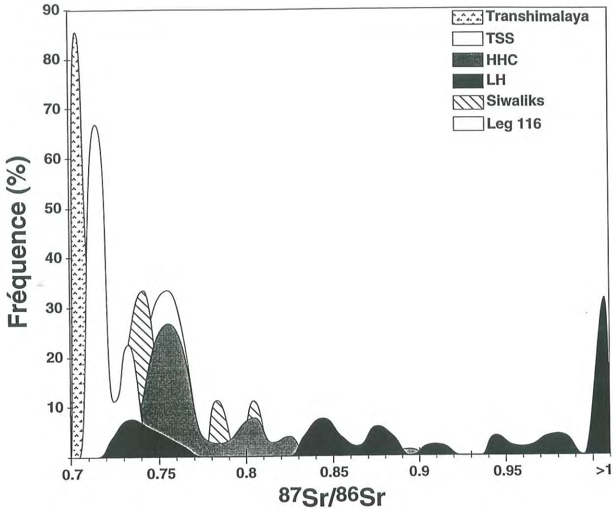
Figure III-14 : Répartition en fréquence des compositions isotopiques du Sr des formations himalayennes et des sédiments du cône du Bengale (Leg 116).
