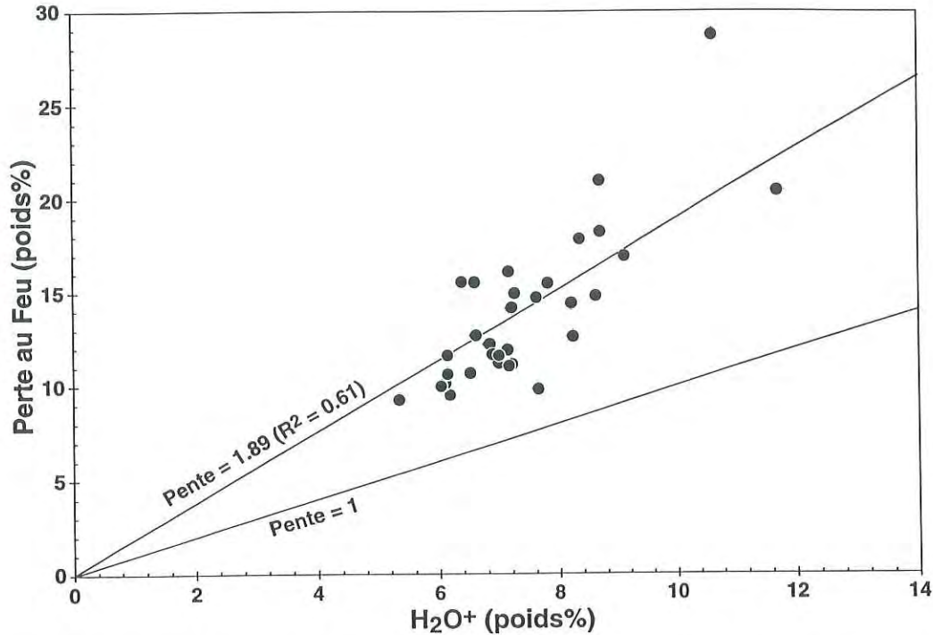
Figure V-5 : Perte au feu en fonction de la teneur en H_2O^+ . La perte au feu est effectuée sur de matériel préalablement étuvé à 110^\circ C , alors que la teneur en H_2O^+ est mesurée sur du matériel traité par un plasma froid d' O_2 et déshydraté à 120^\circ C sous vide.
