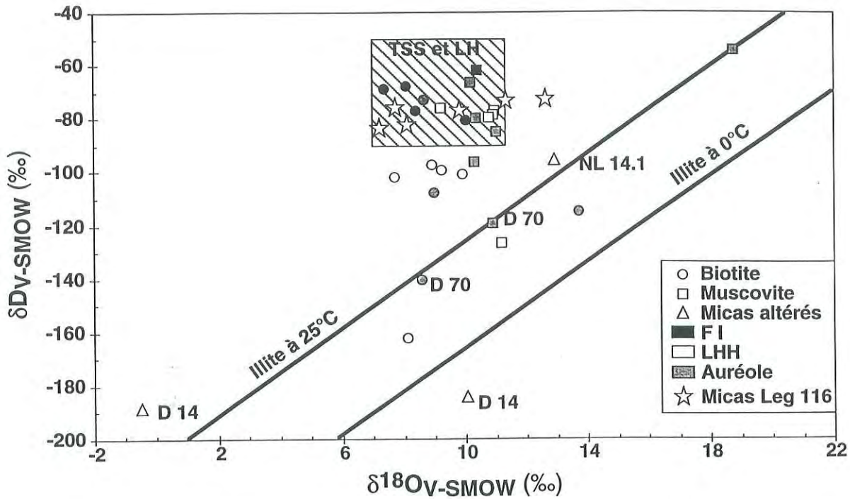
Figure III-20 : Composition isotopique en hydrogène et oxygène des phyllosilicates himalayens. Le champ hachuré pour les TSS et le LH est le champ communément utilisé pour des formations crustales.
