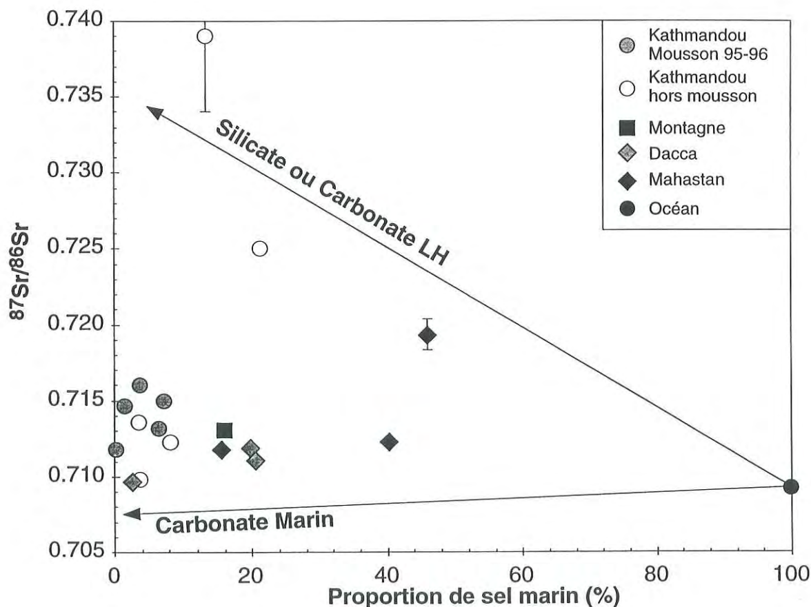
Figure III-28 : Composition isotopique du Sr des précipitations, en fonction de la proportion de Sr marin, sur la base du Cl (voir, paragraphe III-8-2-1). La composition isotopique du Sr marin est de 0.70917 \pm 0.00002 (Hodell et al. , 1990).
