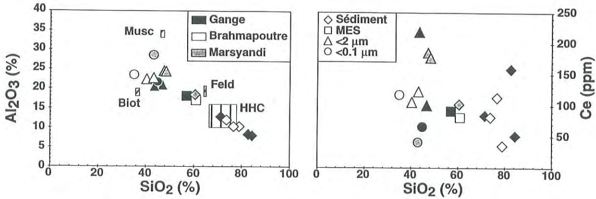
Figure V-11 : Teneur en Al 2 O 3 et en Ce en fonction de la teneur en SiO 2 . Pour les différentes fractions granulométriques du Gange, Brahmapoutre et Marsyandi. Le décalage entre les sables et les MES de part et d'autre de la composition de la roche provient du fractionnement minéralogique et permet de calculer la proportion de matériau transporté par la charge de fond.
