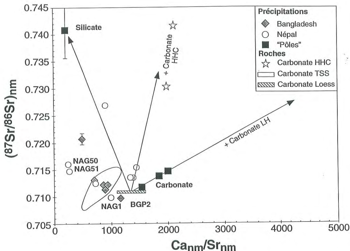
Figure III-29 : Composition isotopique du Sr dissous d'origine non marine en fonction du rapport molaire entre le Ca et le Sr d'origines non marine (corrigeés sur la base du Cl). Le pôle silicaté correspond à GK 4 et le pôle carbonaté à NAG 53, 54 et GK 8. Les compositions des carbonates des TSS sont dans la Table III-8. Les carbonates de la HHC sont similaires aux carbonates disséminés décrits par Blum et al. (1998), mais proviennent des environs de Kathmandou (voir chapitre IV). Les carbonates du LH ont des rapports \text{Ca}/\text{Sr} > 5000 . Les carbonates des lœss sont d'après Gallet et al. (1996), en supposant une minéralogie de calcite pour le Ca.
