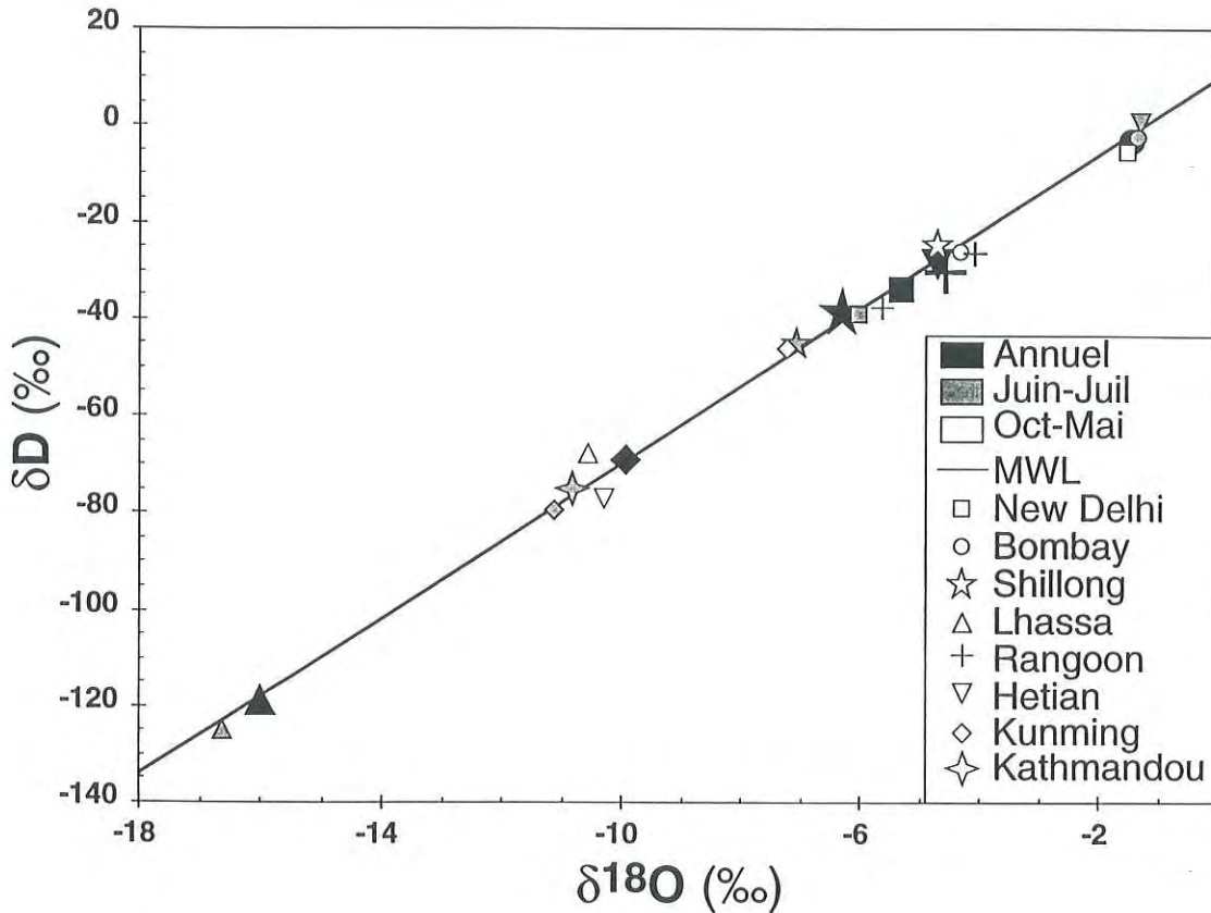
Figure III-23 : Compositions isotopiques (O et H) moyennes des eaux de pluies pour différentes stations de l'IAEA ainsi que la période de mousson 1997 à Kathmandou.
