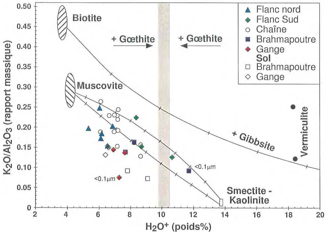
Figure V-6 : Variation du rapport K_2O/Al_2O_3 en fonction de la teneur en H_2O^+ des fractions argileuses et comparaison avec la composition des principaux minéraux argileux. Les données sur les biotites et les muscovites sont d'après France-Lanord, (1987) ; Guillot, (1993), voir chapitre III. Les vermiculites proviennent du Leg 116 et sont mesurées à la sonde électronique. Leur teneur en eau est estimée par différence (Galy, 1992). Les pôles smectite et kaolinite sont d'après Deer et al. , (1992), et ont permis le calcul des relations de mélange, graduées de 10 en 10%. Les pôles gibbsite et goëthite sont respectivement Al(OH)_3 et FeO(OH) pur.
