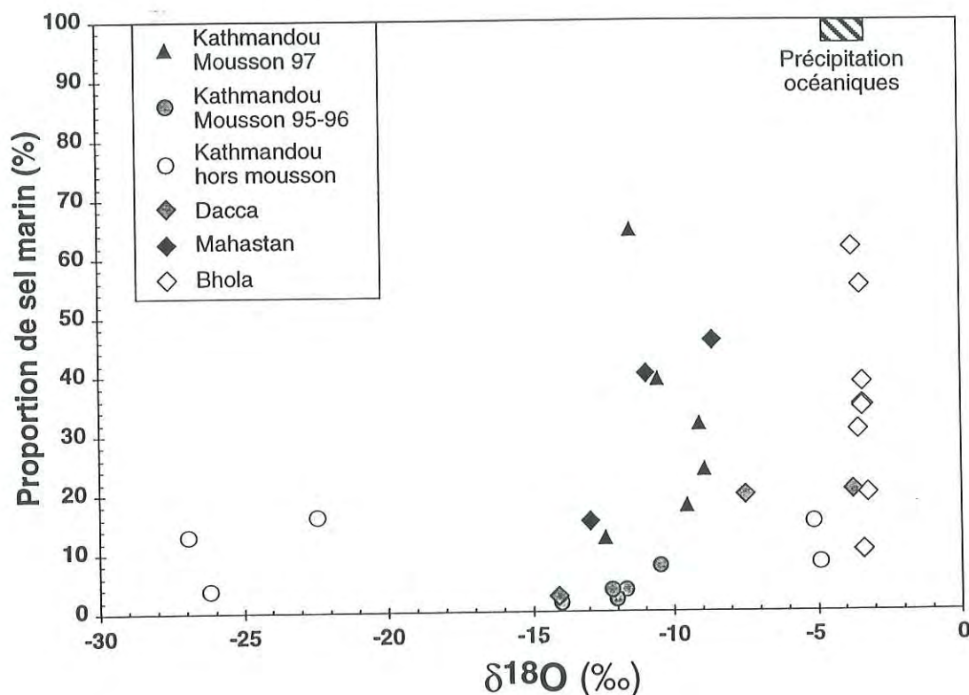
Figure III-26 : Contribution des sels marins à la chimie des eaux de pluies du Népal et Bangladesh en fonction de leur composition isotopique en oxygène.
