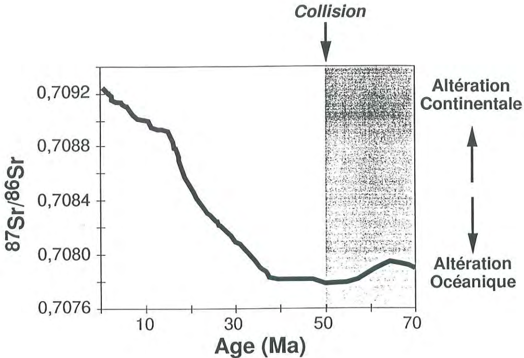
Figure 1 : Variation de la composition isotopique du Sr dissous dans l'océan au cours du temps, d'après Palmer et Elderfield, (1985).
