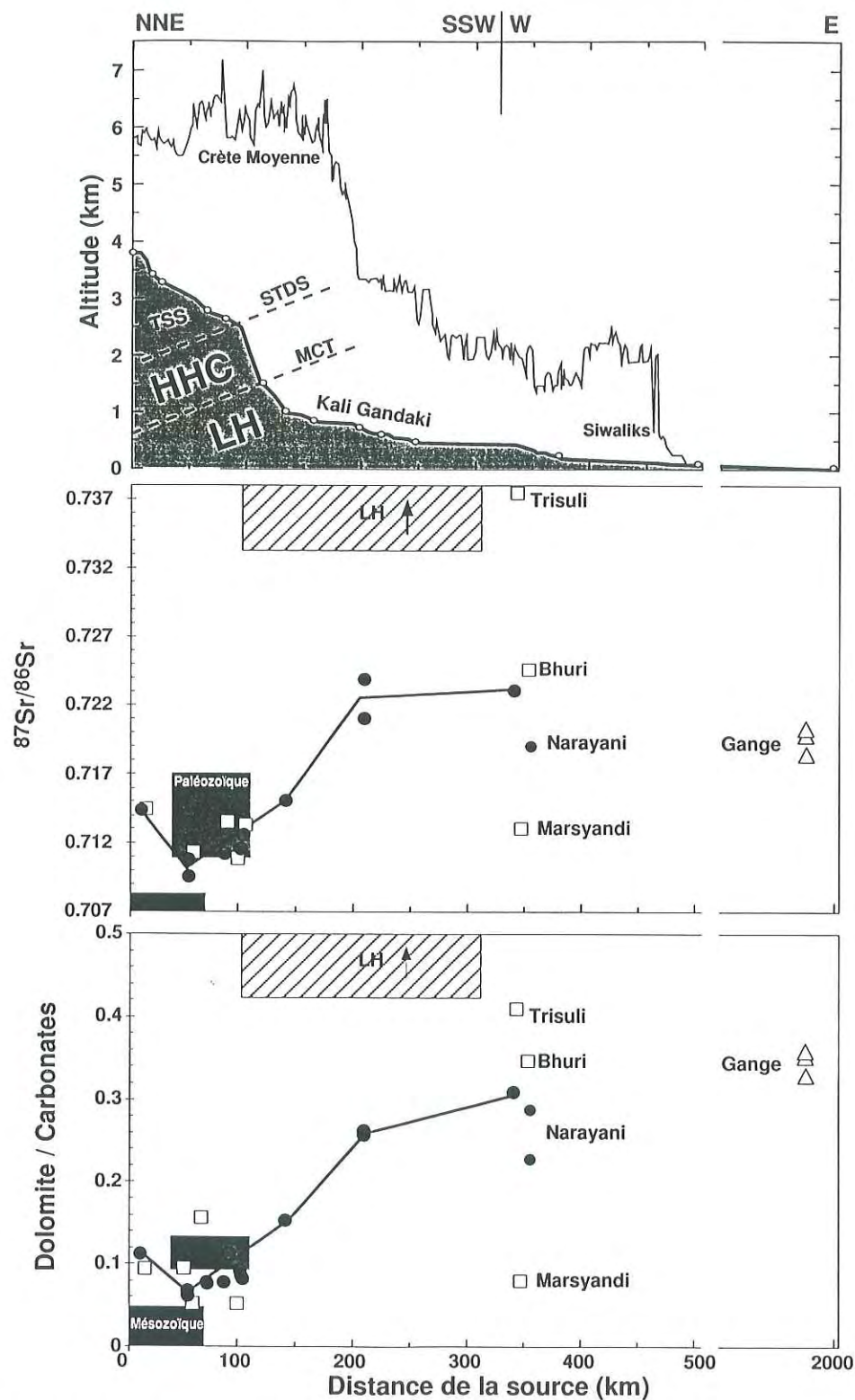
Figure V-17: Variation de la composition isotopique du Sr et de la minéralogie des carbonates des sédiments de rivières le long du profil de la Kali Gandaki, depuis sa source en flanc nord de la chaîne, jusqu'à son entrée dans la plaine du Gange. Le profil topographique est d'après Hurtrez (1998).
