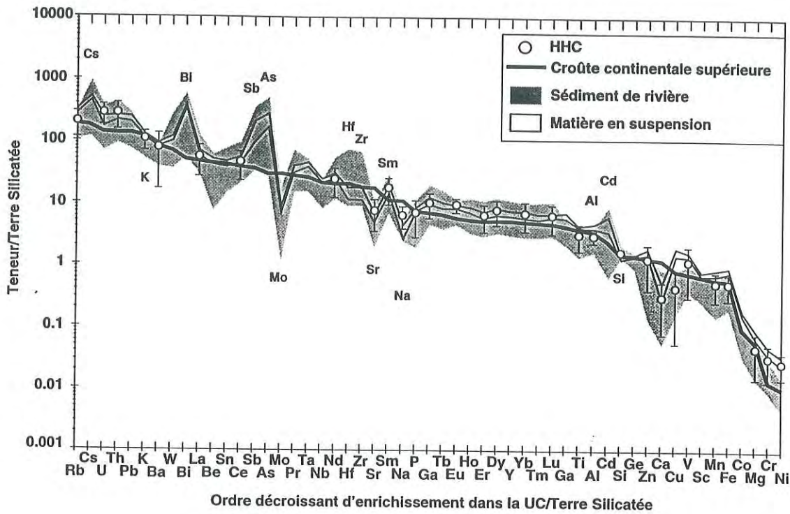
Figure IV-11 : Composition chimique des éléments majeurs et traces des sables des principales rivières analysées, des MES du Bangladesh et de la HHC normalisé à la chimie de la terre silicatée. La composition de la croûte continentale est d'après Taylor et McLennan, (1995) ; Plank et Langmuir, (1998). Les éléments tels que As, Bi, Cs, Mo et Sb ont des teneurs significativement différentes de celle de la CCS. Le manque de données sur la HHC ne permet pas de dire si c'est un caractère lié à la chimie des roches sources ou si cela provient d'une incorporation de ces éléments par les sables lors du transport.
