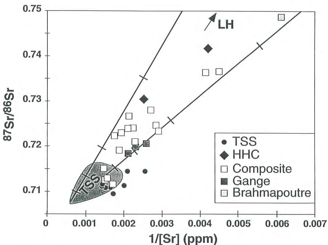
Figure V-18 : Composition isotopique du Sr en fonction de 1/[Sr] dans les sédiments de rivières. Les deux droites correspondent à un mélange entre le LH ([Sr] = 50 ou 100 ppm et ^{87}\text{Sr}/^{86}\text{Sr} = 0.845) et les TSS ([Sr] = 700 et ^{87}\text{Sr}/^{86}\text{Sr} = 0.713 ou [Sr] = 1600 et ^{87}\text{Sr}/^{86}\text{Sr} = 0.7079). Les compositions des sédiments de rivières impliquent que le pôle non radiogénique du LH (voir Chapitre III) n'est pas physiquement érodé.
