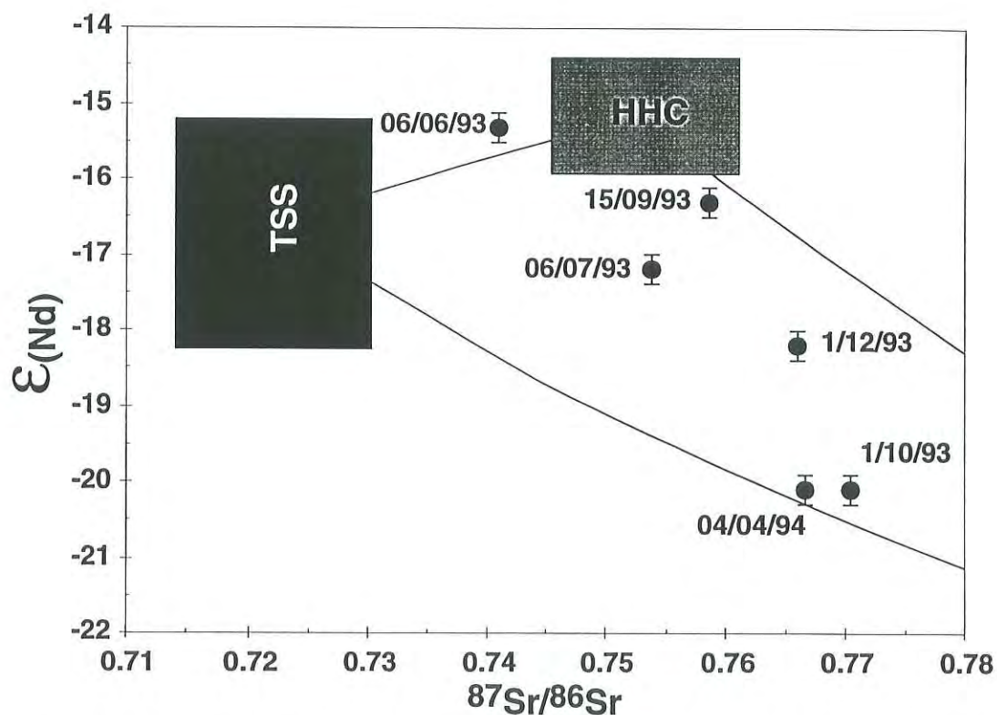
Figure V-26 : Composition isotopique du Nd en fonction de celle du Sr pour la fraction silicatée des sédiments de la Trisuli à Betrawati. La date de prélèvement est indiquée à proximité de chaque point. Les échantillons des périodes sèches contiennent plus de matériel dérivé du LH.
