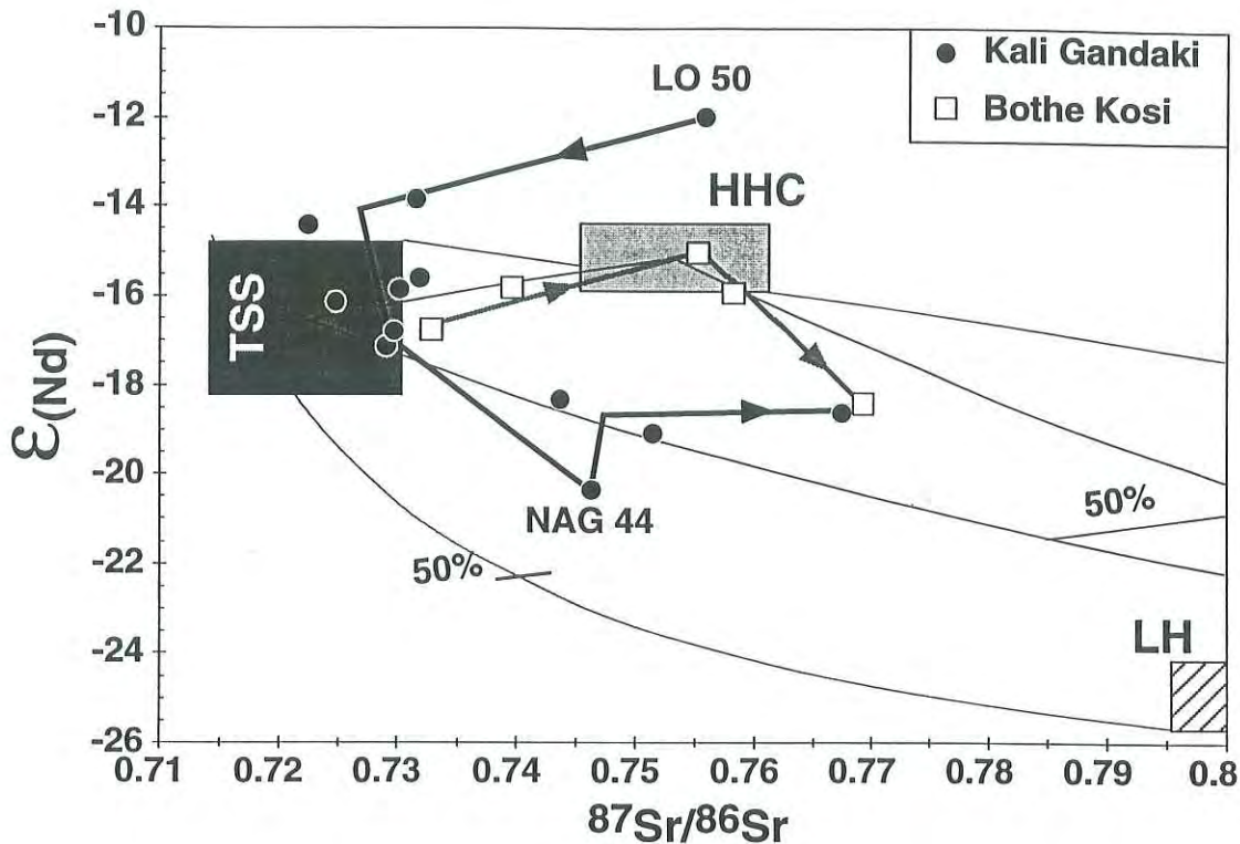
Figure V-23 : Composition isotopique du Nd en fonction de celle du Sr pour la fraction silicatée des sédiments de la Kali Gandaki (cette étude) et des roches totales de la Bhote Kosi (Harris et al. , 1998). Les pôles et courbes de mélanges sont similaires à la figure V-21. La Kali Gandaki documente un mélange leucogranite TSS dans sa partie supérieure puis TSS-LH dans sa partie moyenne, avant de voir l'influence de la HHC, après NAG 44. La Bhote Kosi montre plutôt un mélange TSS-HHC puis l'ajout du LH.
