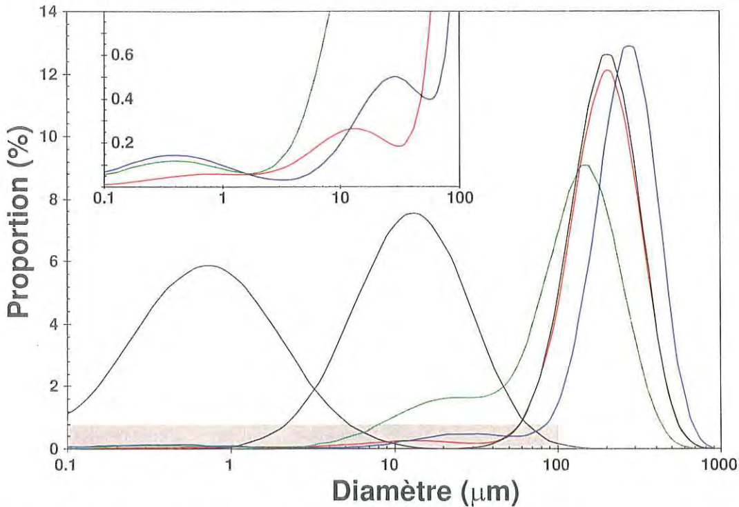
Figure V-2 : Convolution de 3 répartitions granulométriques qui suivent une loi de Poisson : la courbe rouge correspond à la somme dans les proportions de 1/3.5/95.5 des trois répartitions de Poisson en noir. Les courbes bleu et verte sont obtenues en faisant varier le mode de ces trois répartitions et les proportions de mélange. La zone grisée correspond à l'encart.
