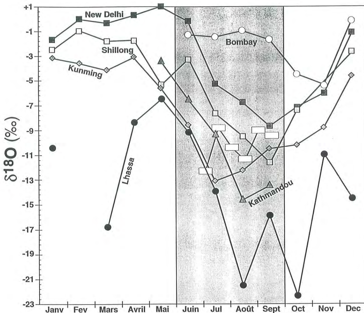
Figure III-24 : Variation mensuelle des \delta^{18}O des précipitations pour les stations de l'IAEA, la moyenne des évènements individuels (triangles) et de l'échantillonnage intégré de la mousson 1997 (rectangles blancs) à Kathmandou.
