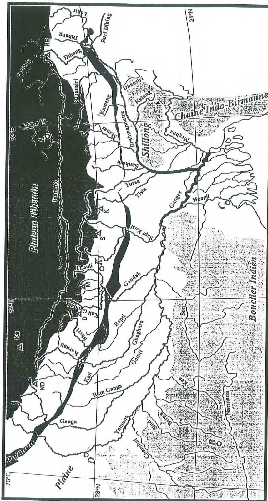
Figure I-3 : Réseau Hydrographique du bassin du Gange-Brahmapoutre. B : Bhopal ; D : Delhi ; K : Kathmandou ; L : Lhasa
