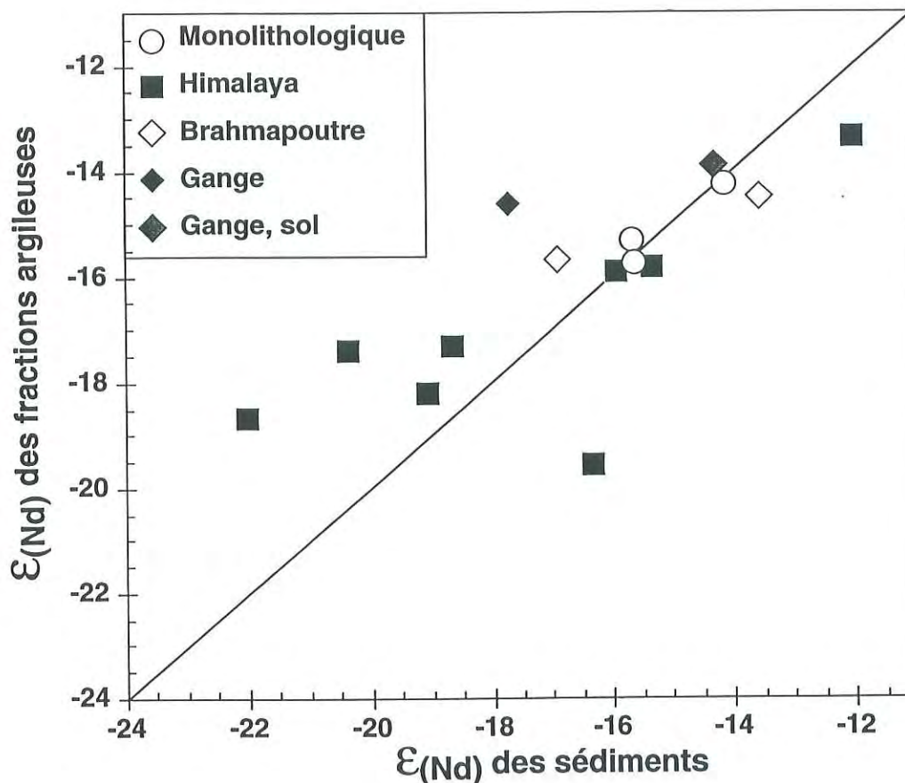
Figure V-30 : Variation de la composition isotopique du Nd des silicates de la fraction <math><2\mu\text{m}</math> en fonction de la composition du silicate total. Les bassins ne drainant qu'une seule formation ne montrent pas de différence entre la fraction argileuse et le silicate total. Pour les bassins versant plus importants, la différence entre les argiles et le sédiment total implique une origine différente de ces 2 fractions. La fraction argileuse est généralement plus enrichie en matériel dérivé du Haut Himalaya.
