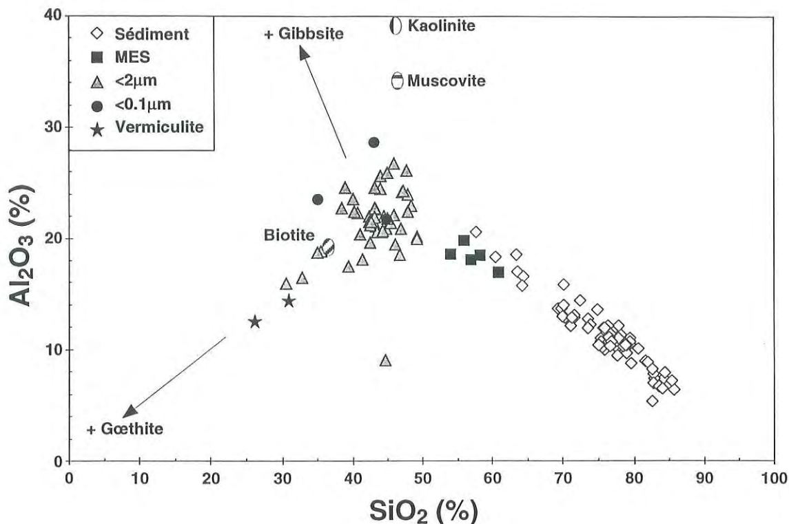
Figure V-8 : Variation de la teneur en Al_2O_3 en fonction de la teneur en SiO_2 pour la fraction silicatée des sédiments, celle des MES et les fractions granulométriques <2µm et <0.1µm. La composition de certains minéraux est rappelée.
