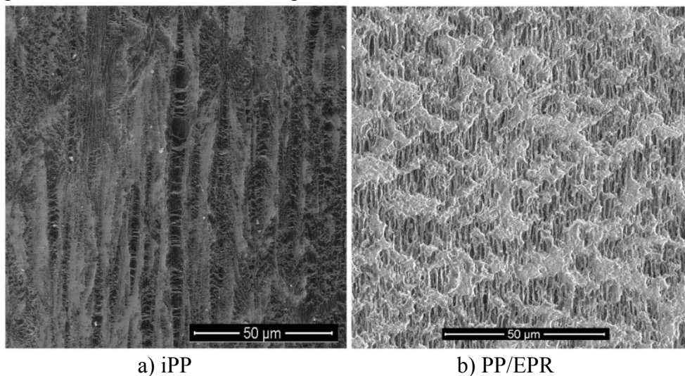
Figure IV.3.6 : Observations post mortem MEB a) du iPP et b) du PP/EPR après une traction uniaxiale jusqu'à la déformation vraie 1,2 à 5 \cdot 10^{-3} \text{ s}^{-1} et 22 \text{ }^\circ\text{C} . L'axe vertical correspond à l'axe de traction.
