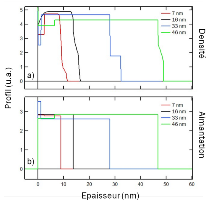
Figure 59 : Profils des a) densités obtenues par les mesures de réflectivité en neutrons et b) de l'aimantation des différents échantillons.
