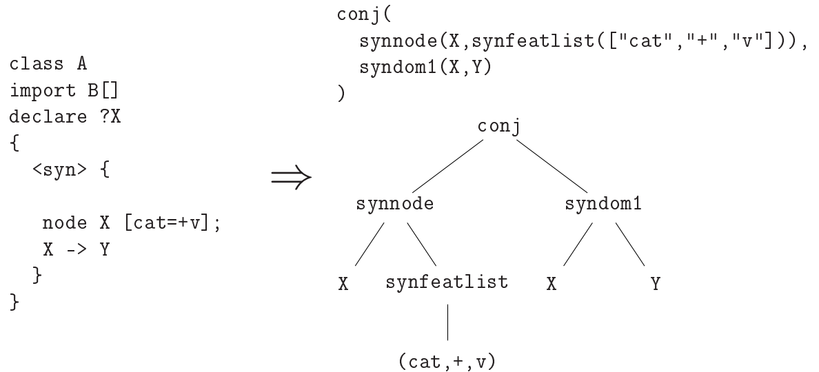
FIG. 3.1 – AST correspondant
