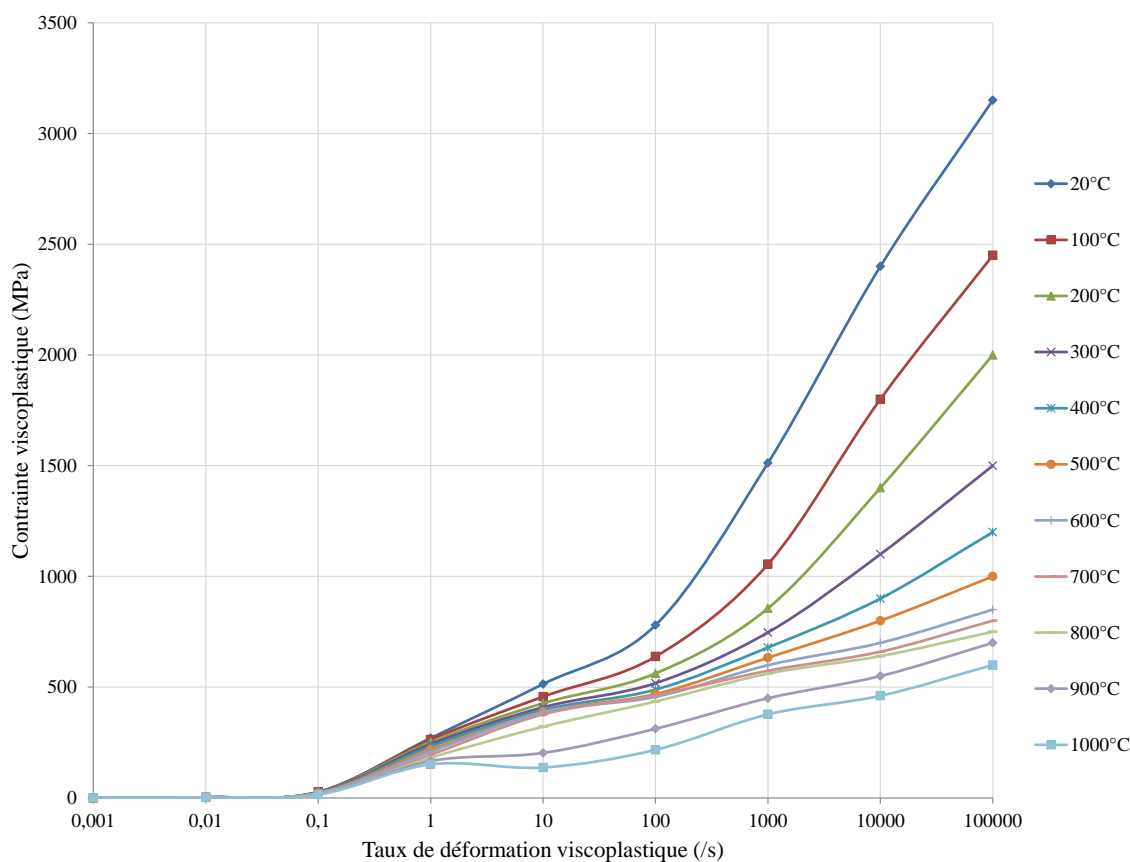
Figure 92: Contrainte de cisaillement fonction du taux de déformation et de la température
