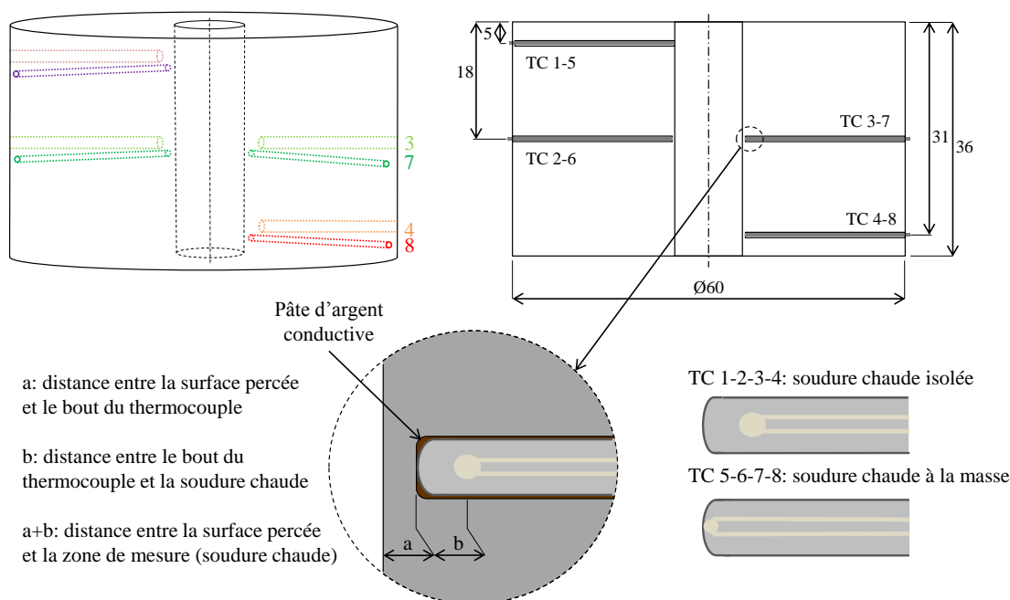
Figure 24: Implantation des thermocouples dans l'échantillon
