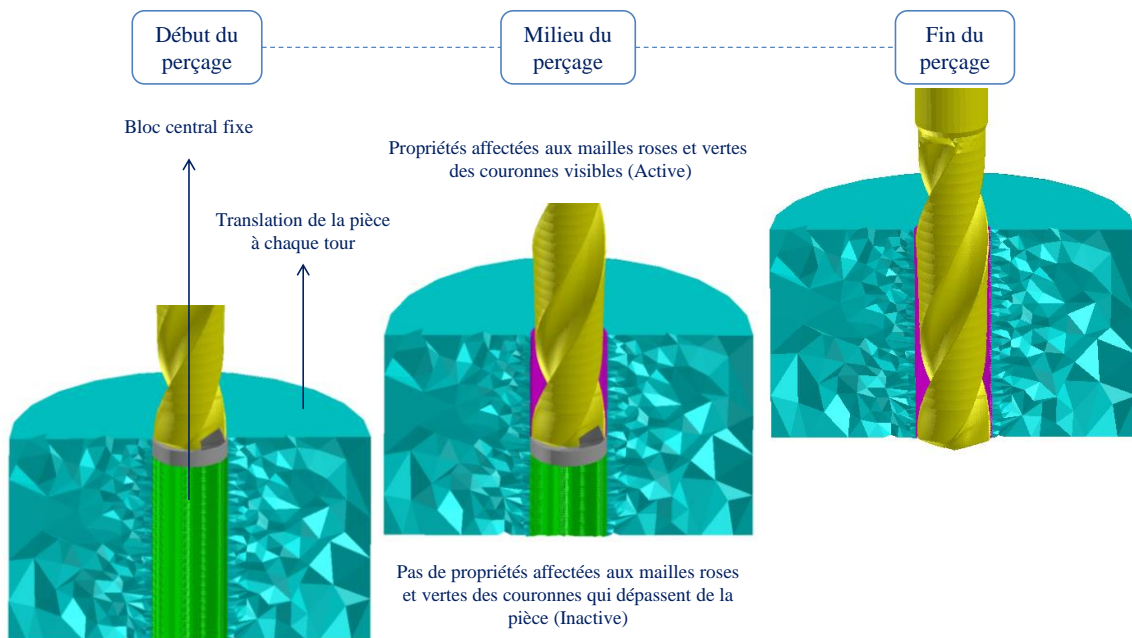
Figure 83: Positionnement des éléments de maillage à différentes étapes de calcul
