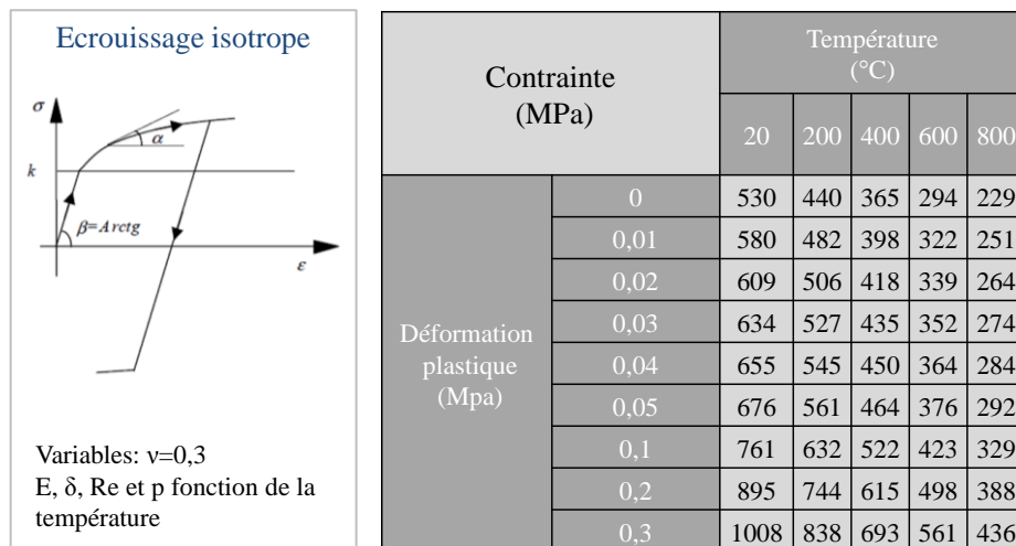
Figure 118: Description du comportement thermoélastoplastique du matériau
