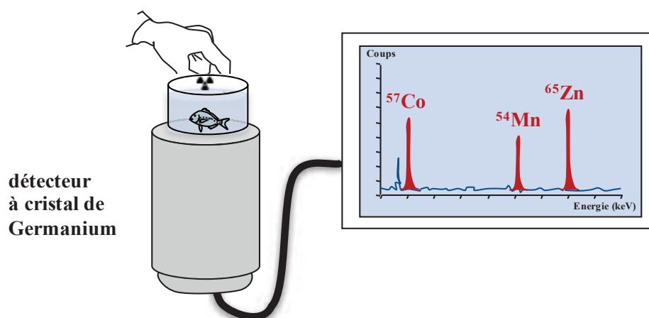
Figure 4. Schéma simplifié d'un protocole expérimental de single-feeding basé sur l'utilisation de radiotraceurs. Ici est illustré comme exemple une expérience fictive visant à étudier l'effet d'une réduction de pH de l'eau sur le transfert trophique d'éléments traces essentiels (Co, Mn et Zn). Plus de précisions concernant les méthodologies utilisées pour le contrôle et la régulation des facteurs étudiés sont fournies dans les sections « Materials and Methods » des articles disponibles en Annexes (voir Articles 2-9 ).
