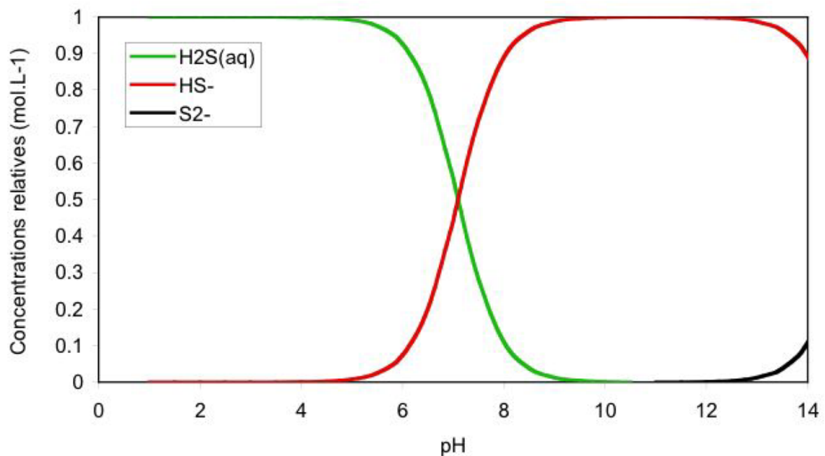
Figure 1. Diagramme de stabilité des espèces dissoutes du soufre dans à 25°C.
