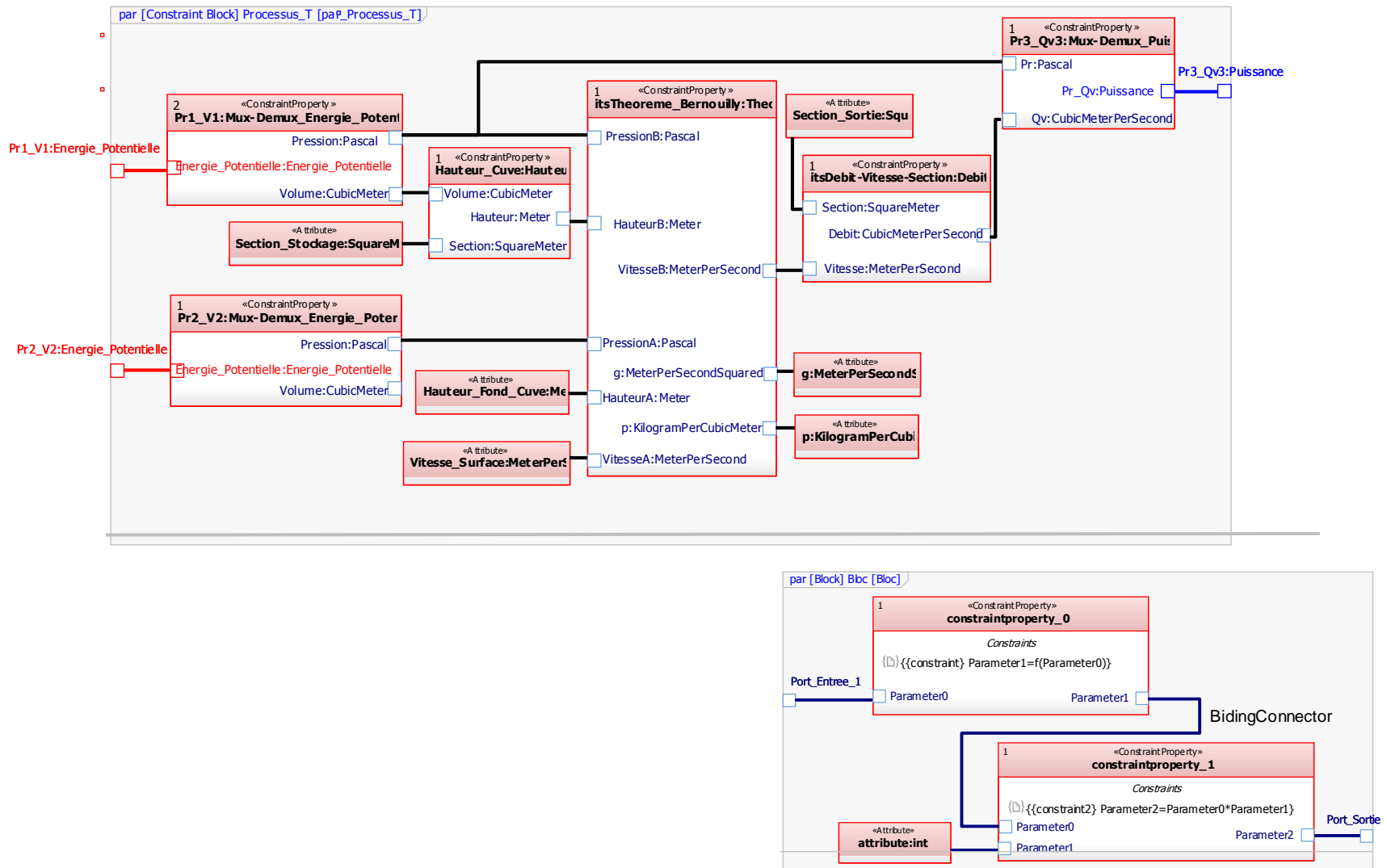
Figure 95 : Diagramme paramétrique SysML – Dynamique du processus T
