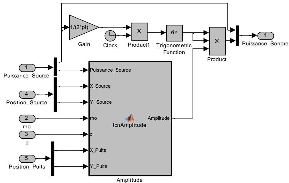
Figure 163 : Bloc Simulink – Interaction fonctionnelle de propagation sonore
