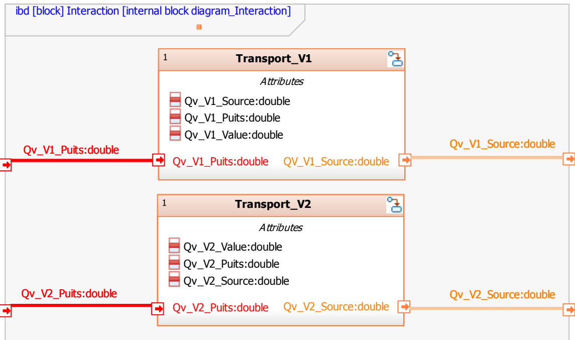
Figure 192 : Spécification des fonctions de transport par les voies V1 et V2 entre la plate-forme CISPI et son environnement
