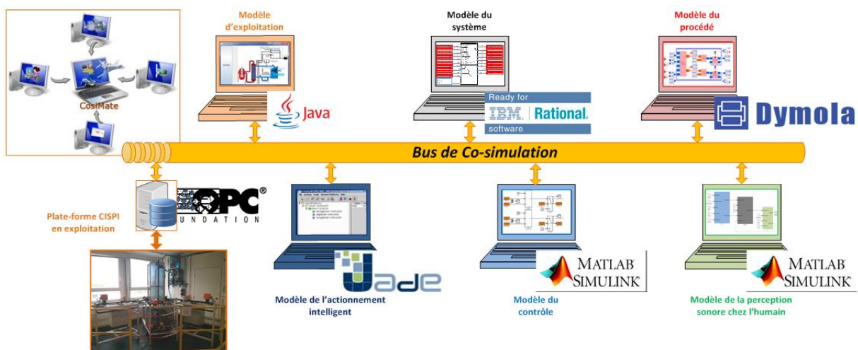
Figure 60 : Environnement de co-modélisation de la plate-forme CISPI
