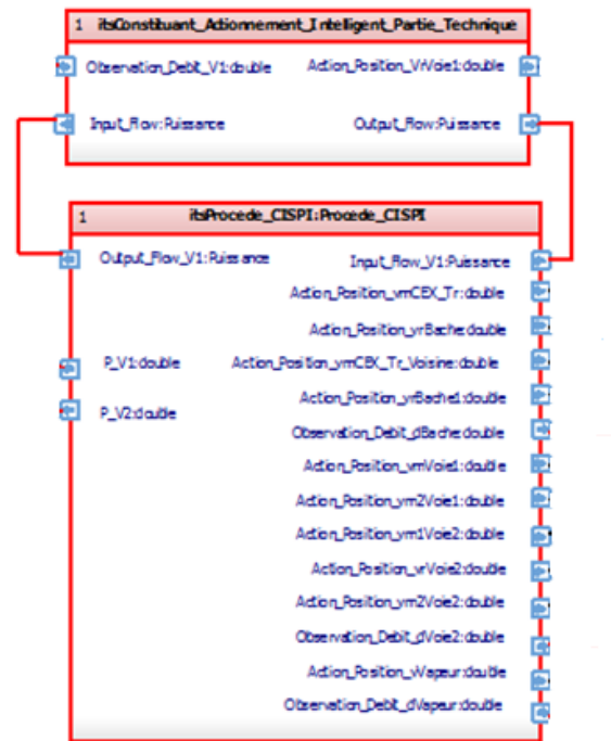
Figure 143 : Spécification ( S_{IPhy\_SysML} ) des interfaces externes du processus CISPI à un niveau d'abstraction logique
