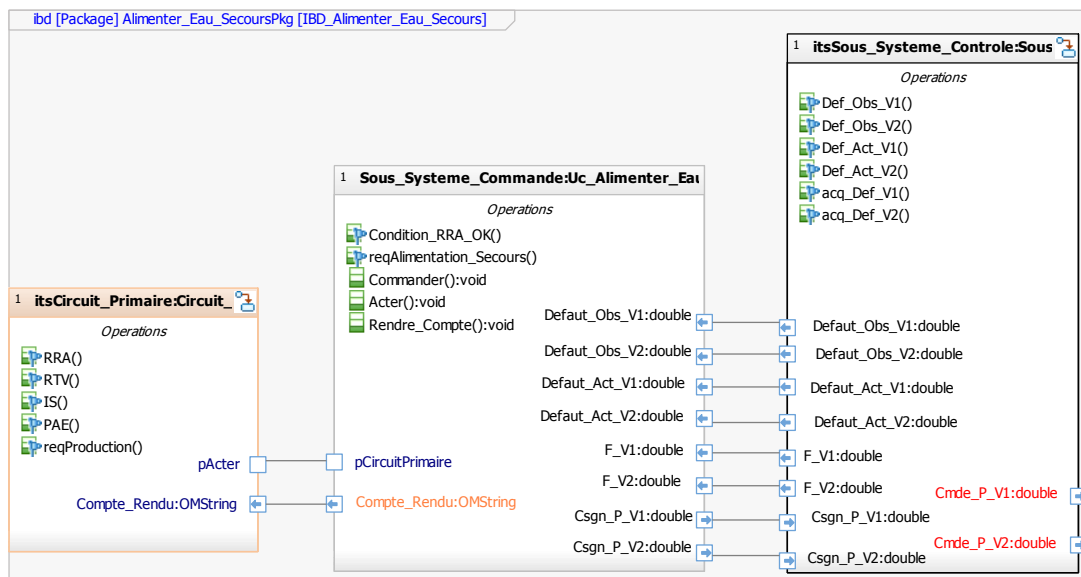
Figure 120 : Diagramme interne de blocs SysML - Interactions entre le sous-système de commande et le système extérieur (Circuit_Primaire + Sous_Systeme_Control)
