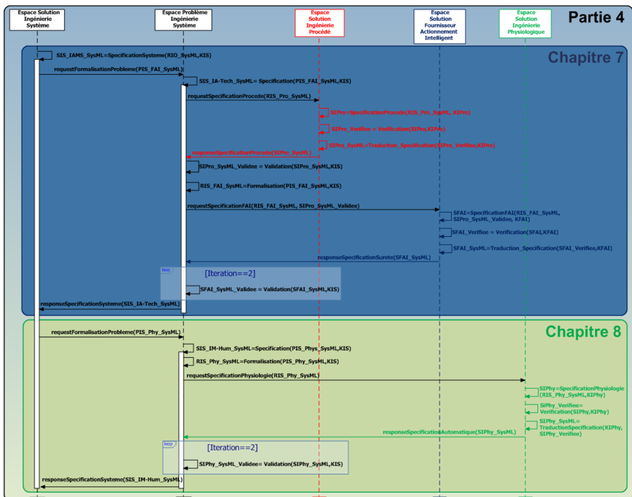
Figure 126 : Diagramme de séquence (seq) SysML - Scénario de co-spécification d'un système d'actionnement et de mesure intelligent
