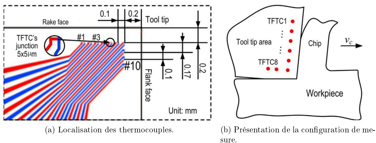
FIGURE 2.14 – Mesure de température lors d'interactions de coupe à l'aide de thermocouples intégrés à l'outil [Li et al. 2013].
