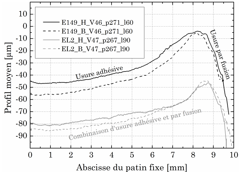
FIGURE 4.11 – Combinaison d'usure adhésive à haute température et d'usure par fusion
